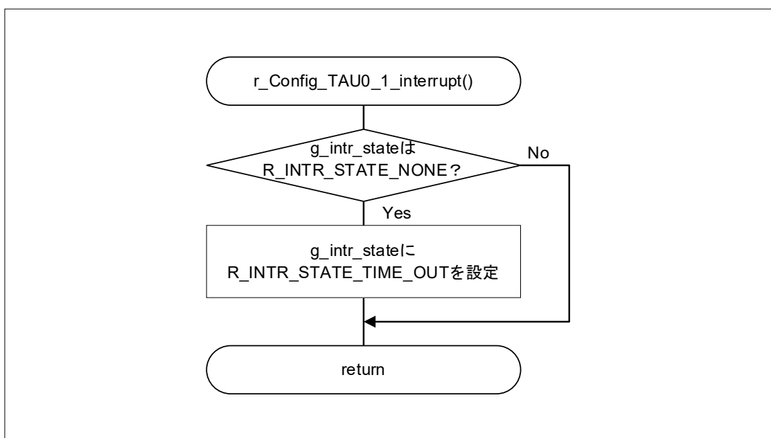
図 4-8 STOP モード移行用タイマ割り込み
