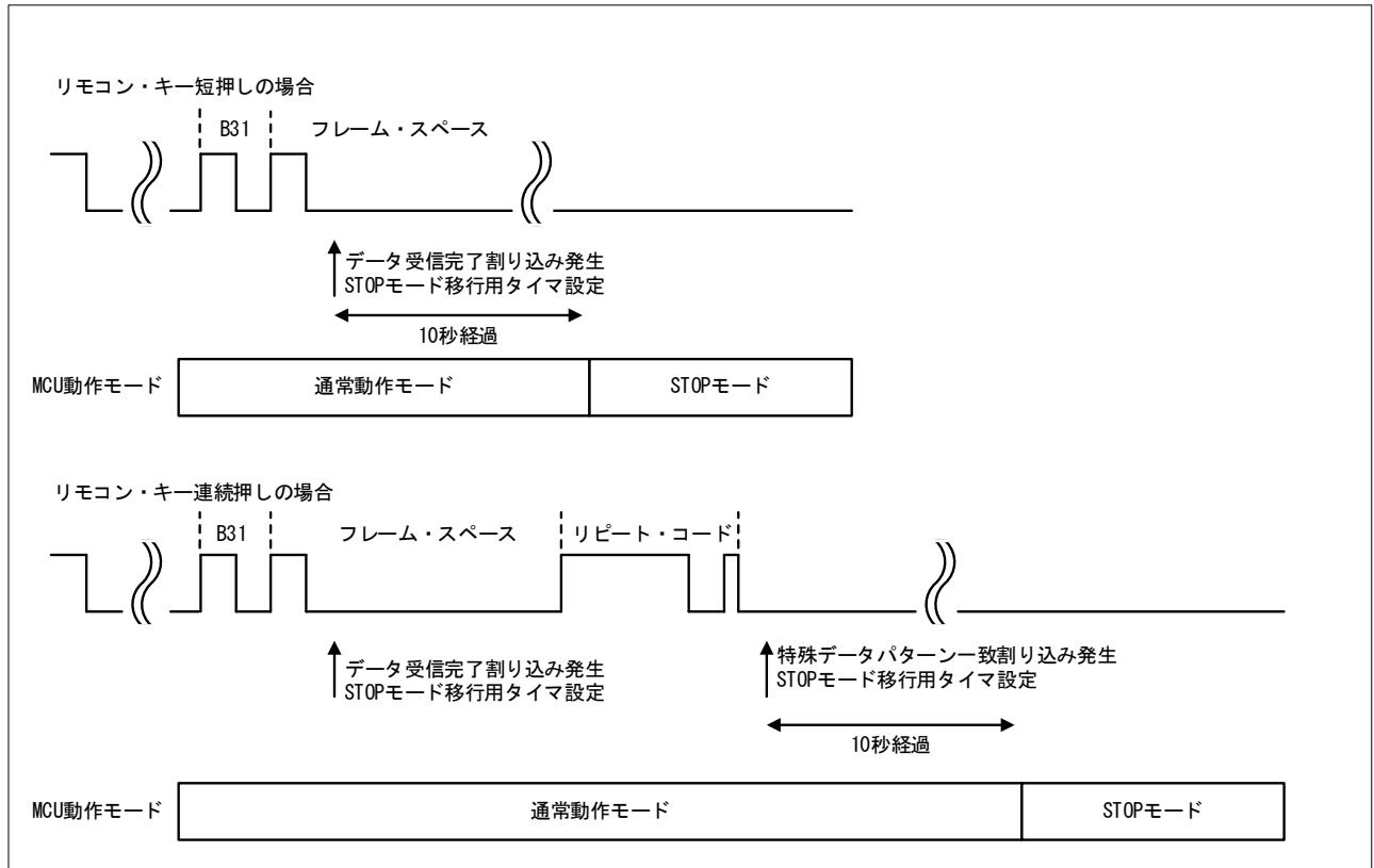
図 1-3 STOP モードへ移行するタイミング
