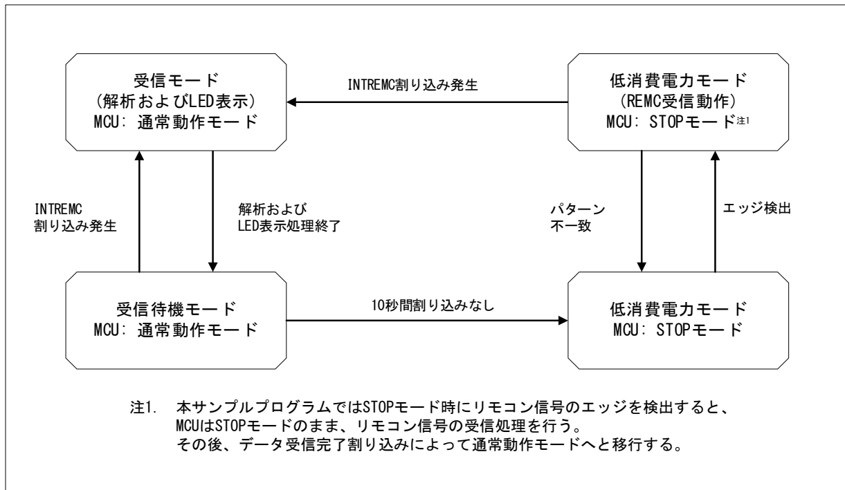
図 1-4 リモコン信号受信の状態遷移図
