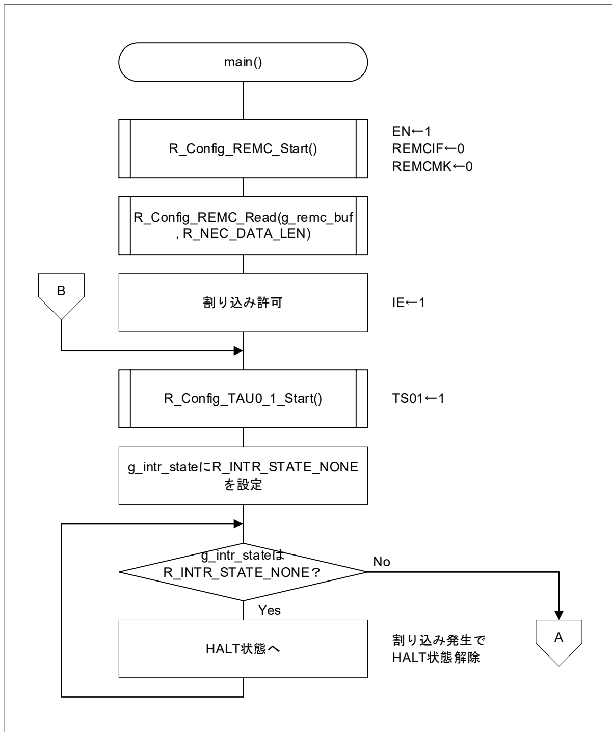
図 4-1 メイン処理 (1/2)
