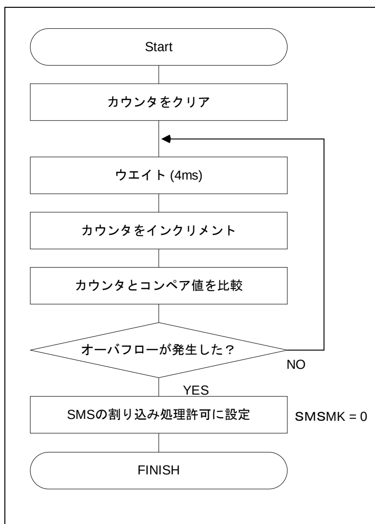
図 4-5 SNOOZE モード・シーケンサの処理
