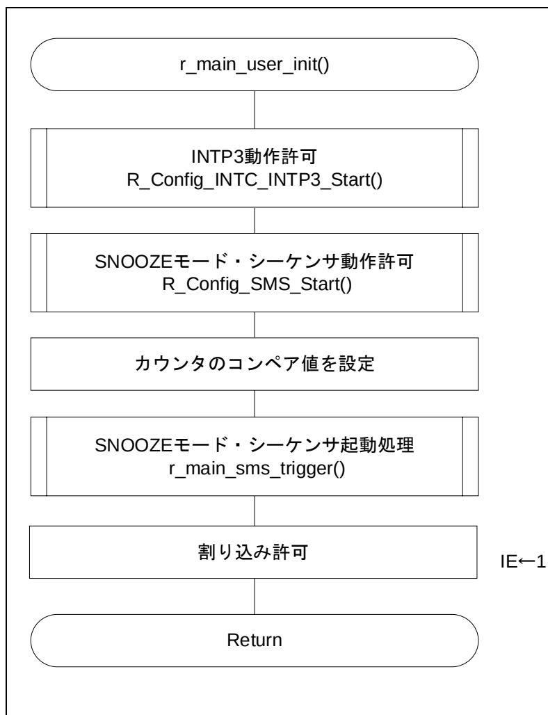
図 4-2 メイン・ユーザー初期設定
