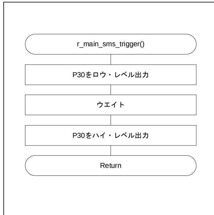
図 4-3 SNOOZE モード・シーケンサ起動処理
