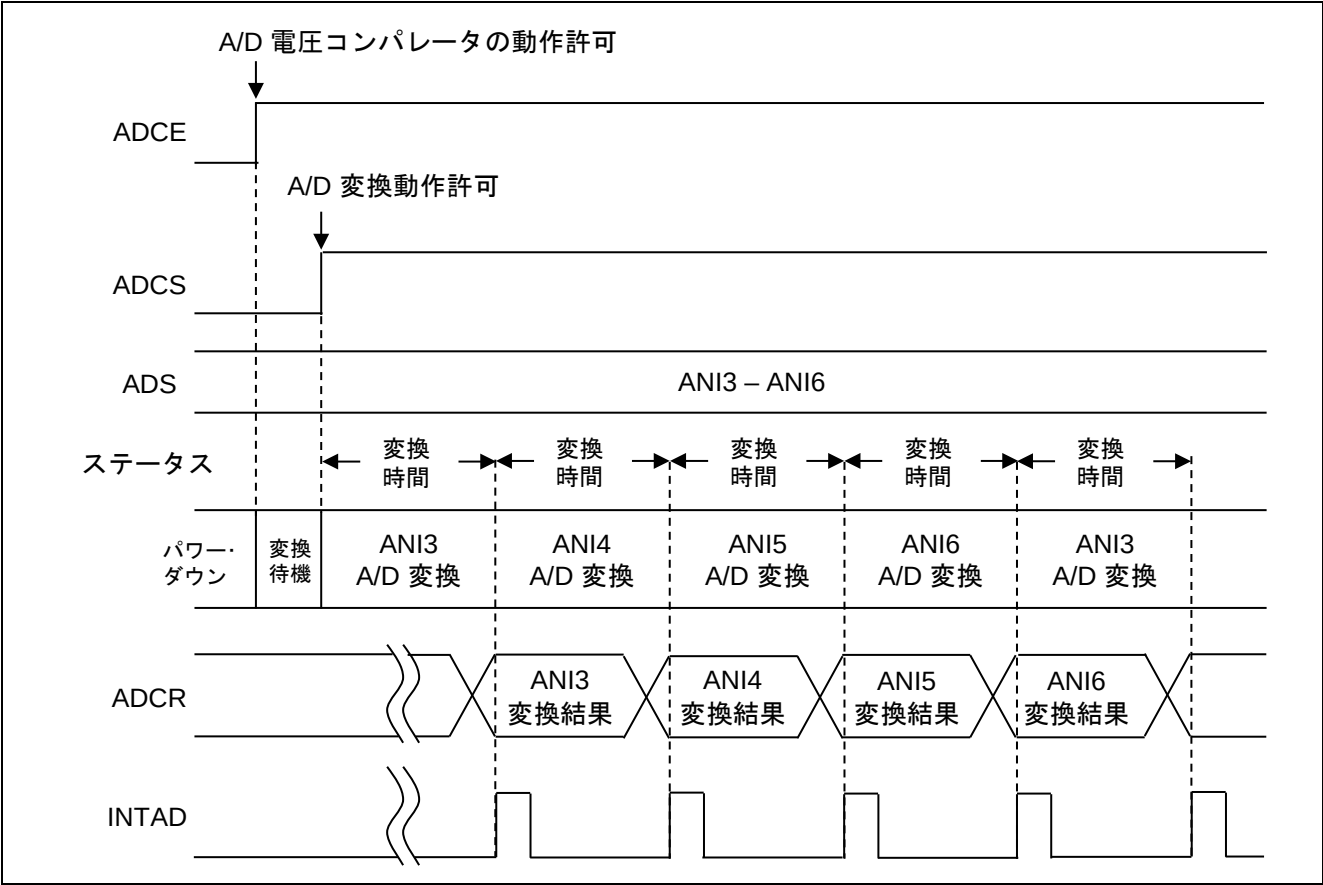
図 1 - 1 A/D コンバータの変換動作
