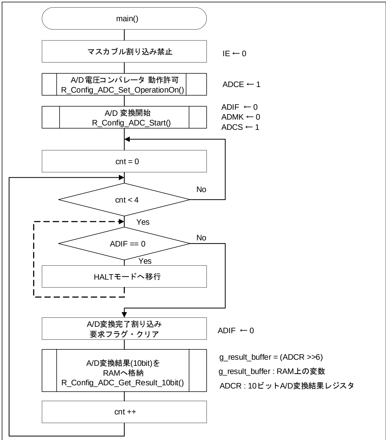
図 3 - 1 メイン処理
