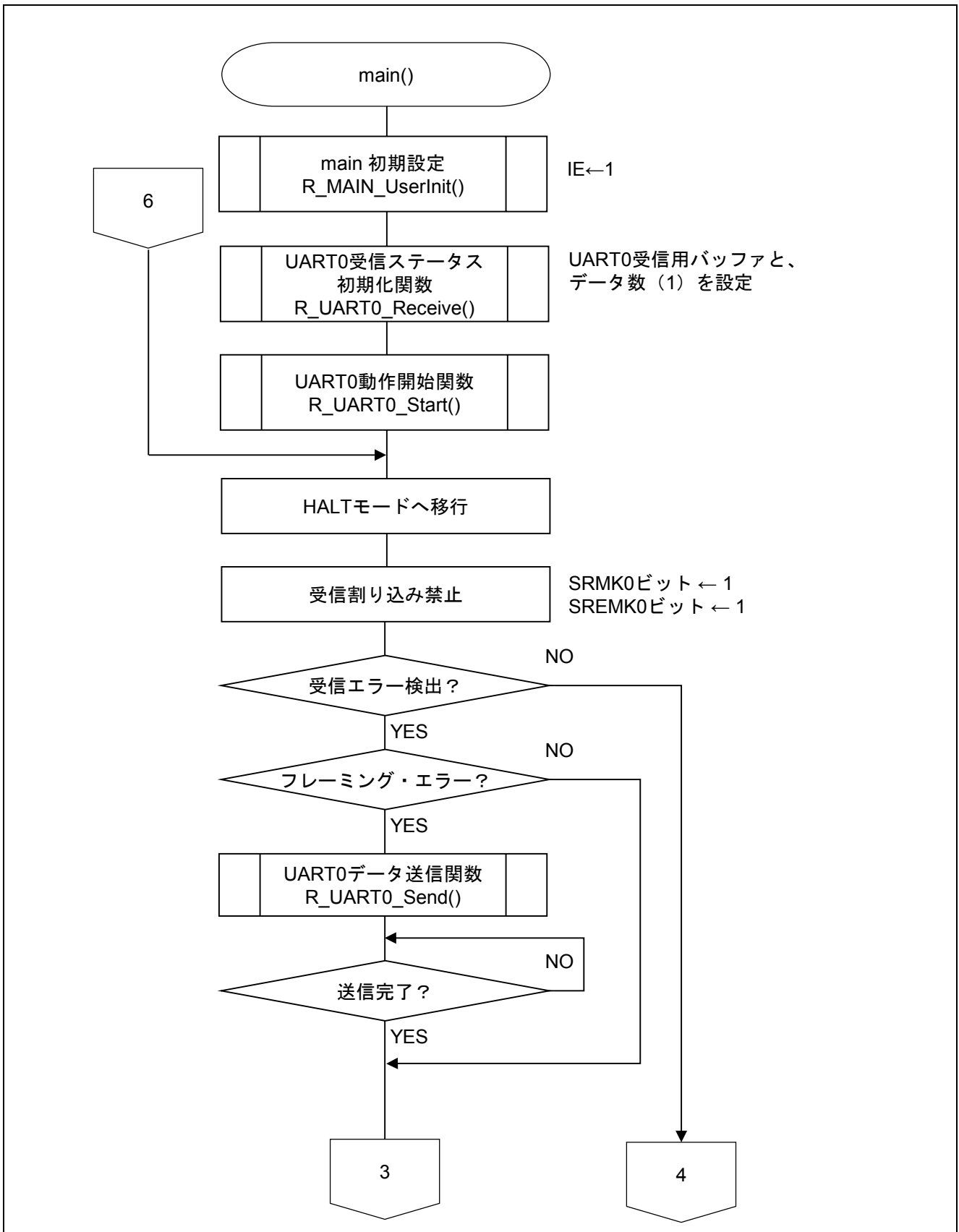
図 5.10 メイン関数 (1/3)
