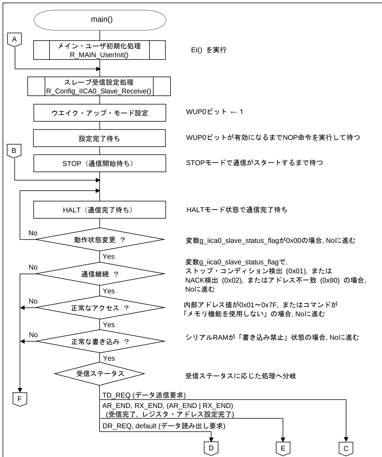
図 5.1 メイン処理(1/2)
