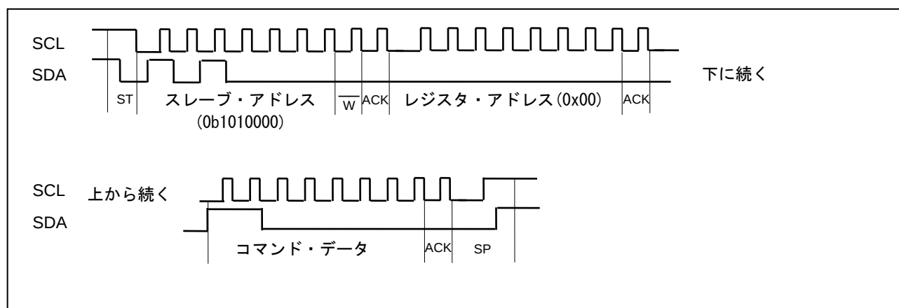
図 1.10 コマンド設定のタイミング・チャート
