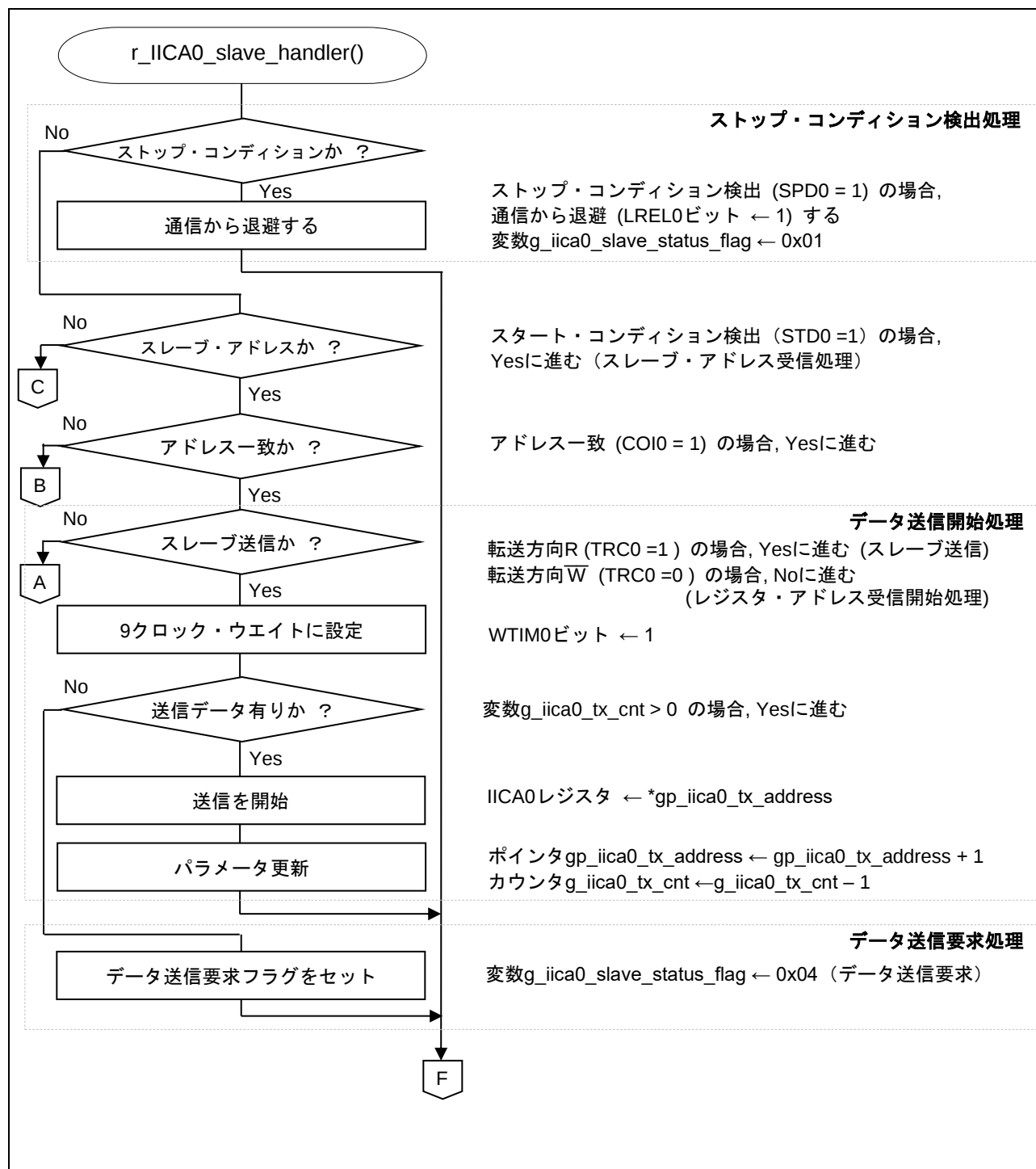
図 5.8 IICA0 割り込み内スレーブ処理 (1/3)
