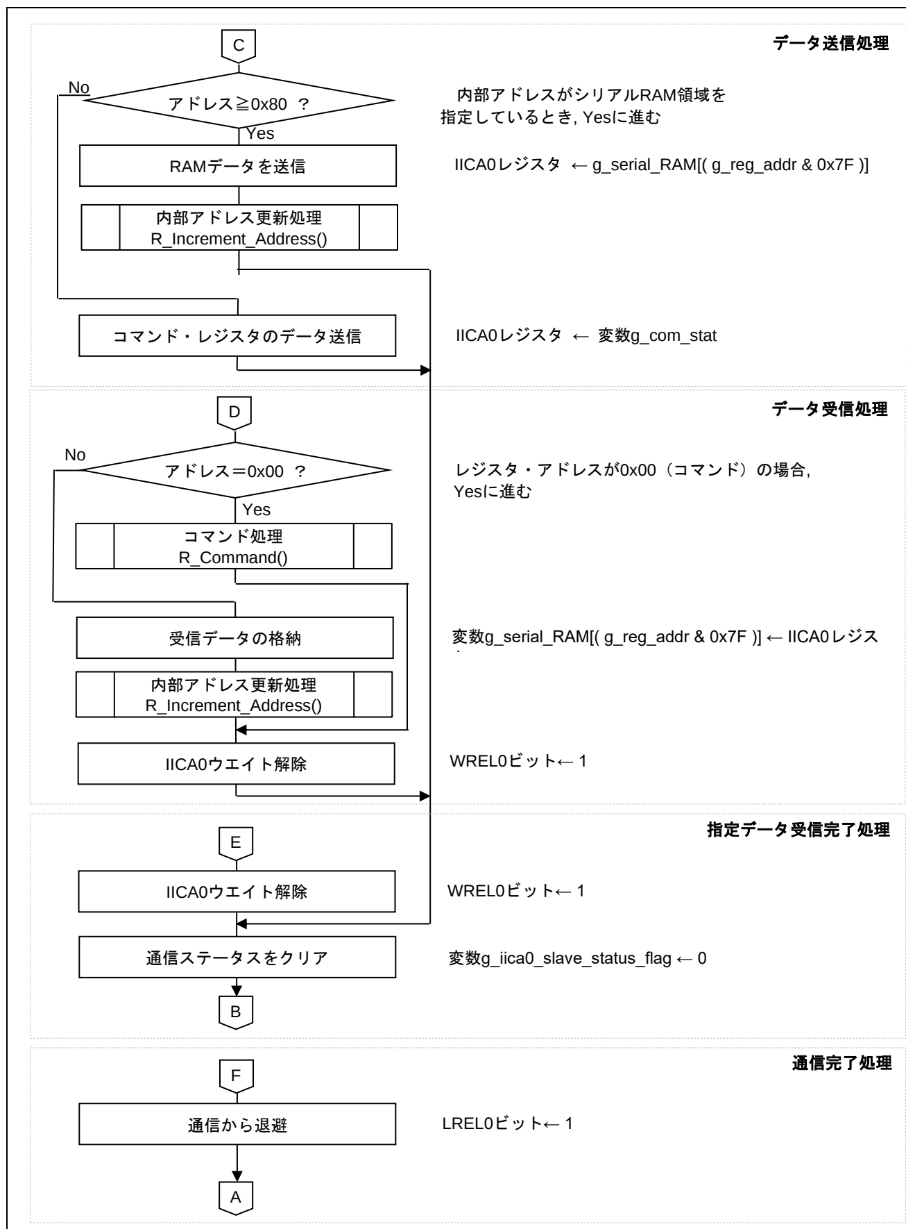
図 5.2 メイン処理 (2/2)
