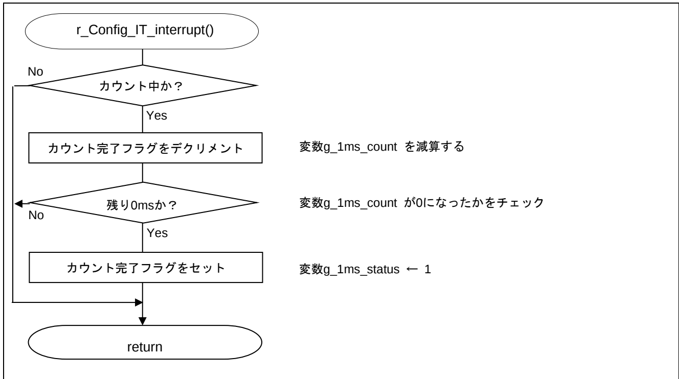
図 5.7 12 ビット・インターバル・タイマ割り込み処理
