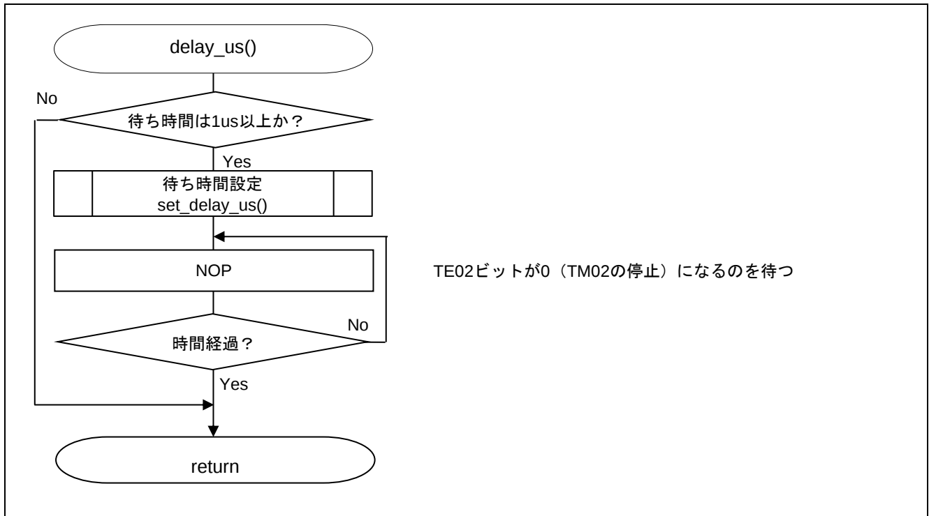
図 5.21 us 単位での時間待ち処理
