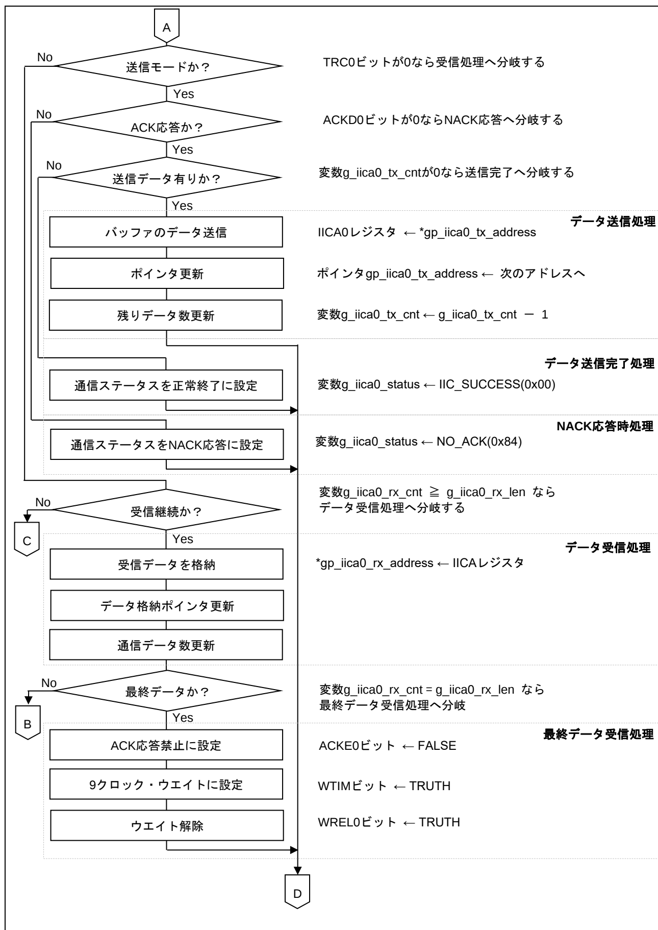
図 5.19 IICA0 割り込み処理 (2/3)
