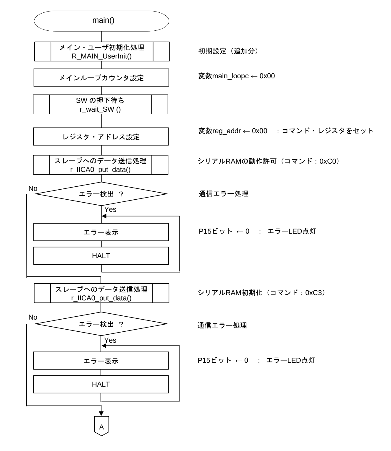
図 5.1 メイン処理（1/3）
