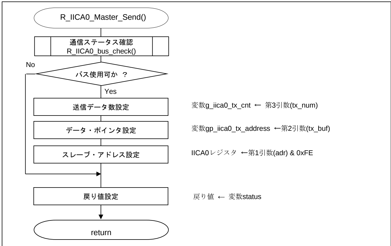
図 5.12 IICA0 マスタ送信起動関数
