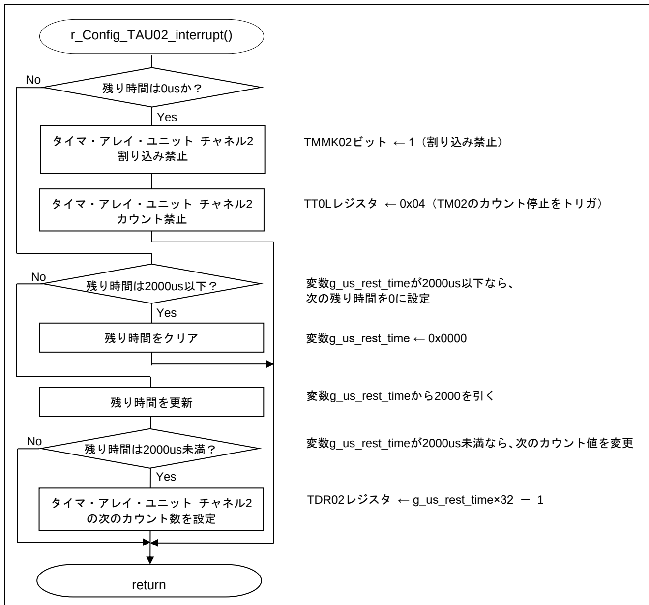
図 5.23 タイマ・アレイ・ユニット チャンネル 2 割り込み処理
