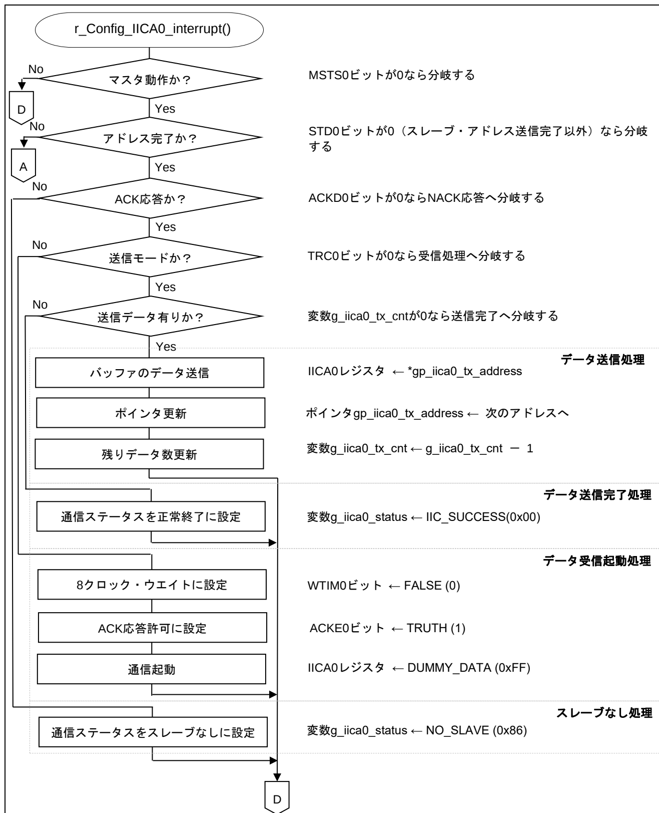
図 5.18 IICA0 割り込み処理 (1/3)
