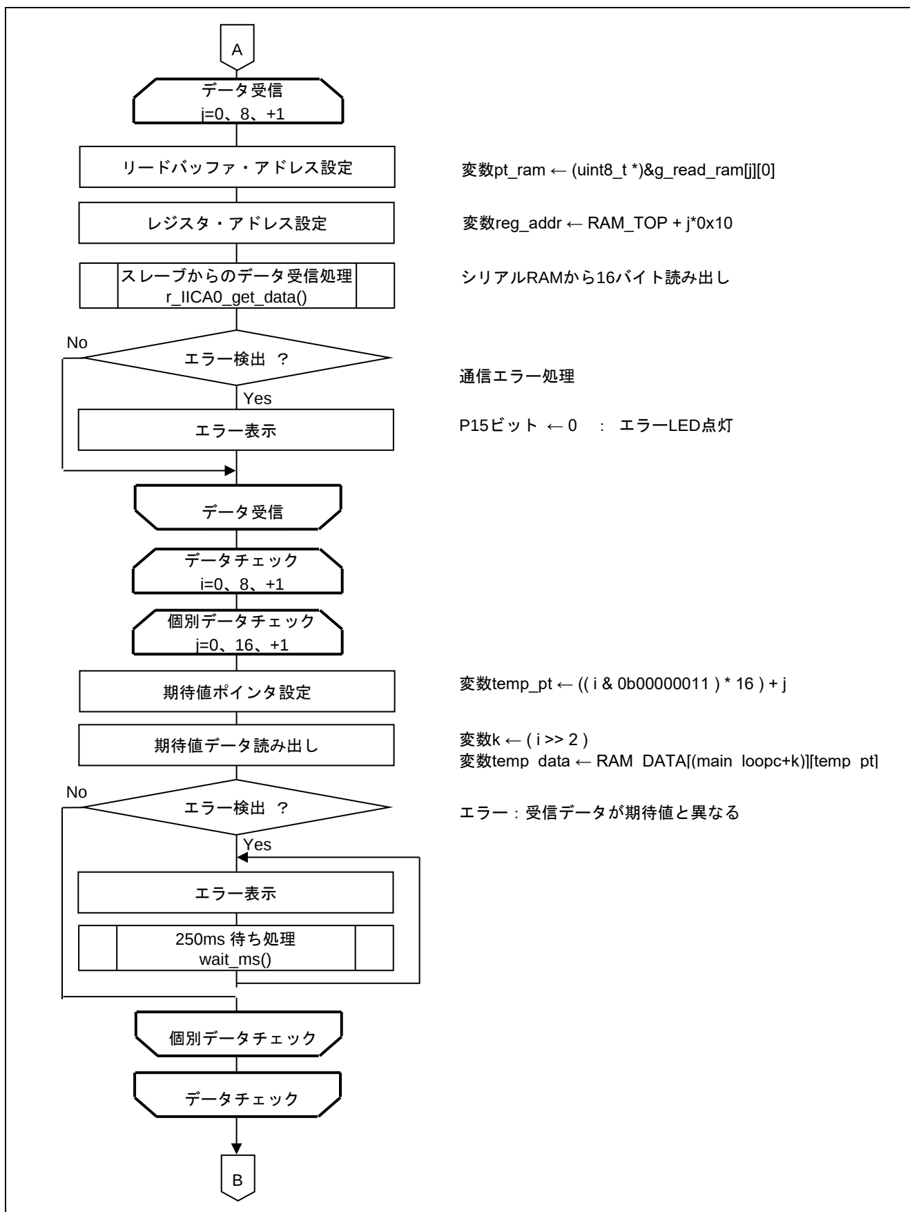
図 5.2 メイン処理 (2/3)
