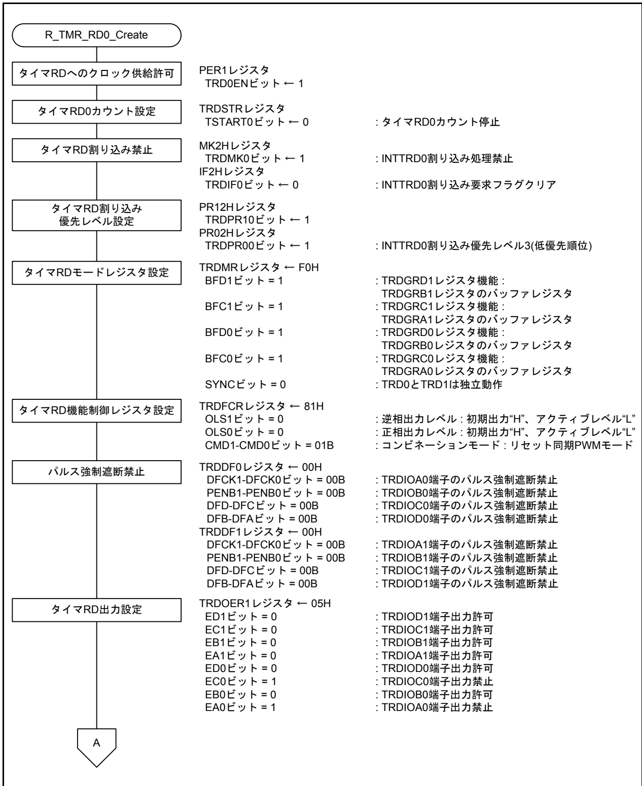
図 4.6 タイマRD初期設定(1/2)
