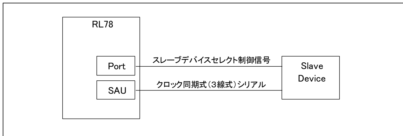
図 1-1 使用例
