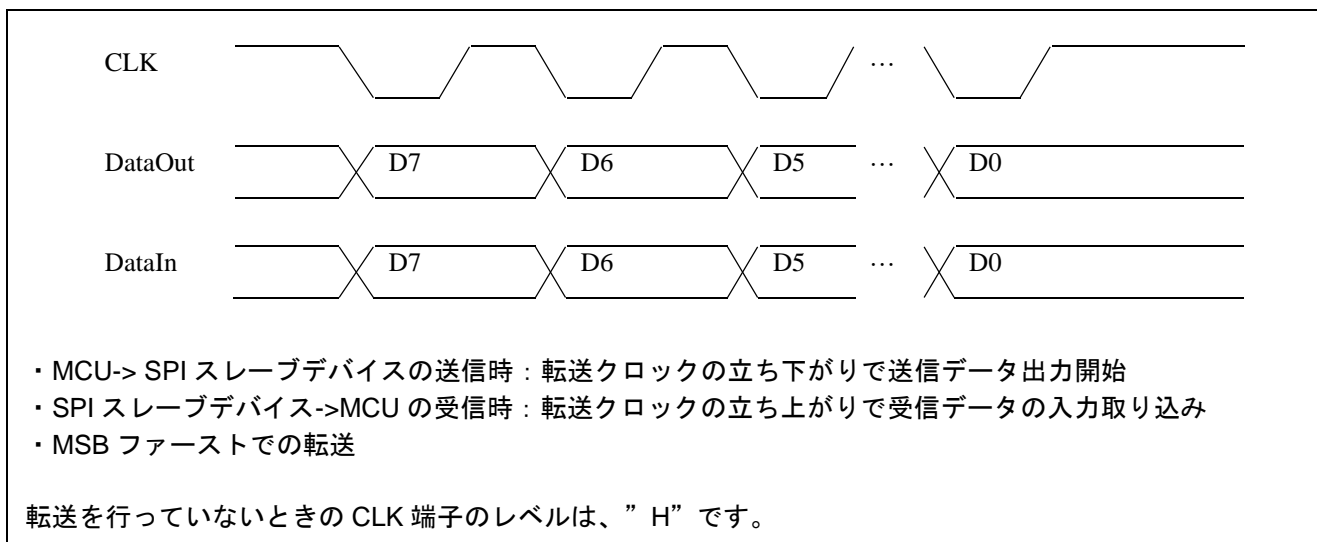
図 5-2 クロック同期式モード タイミング設定
