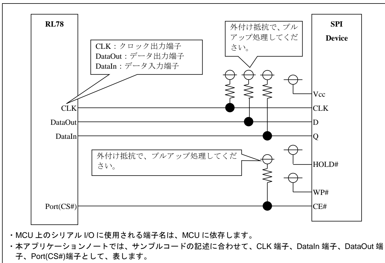
図 4-1 RL78 ファミリ MCU シリアル・アレイ・ユニットと SPI スレーブデバイスの接続例
