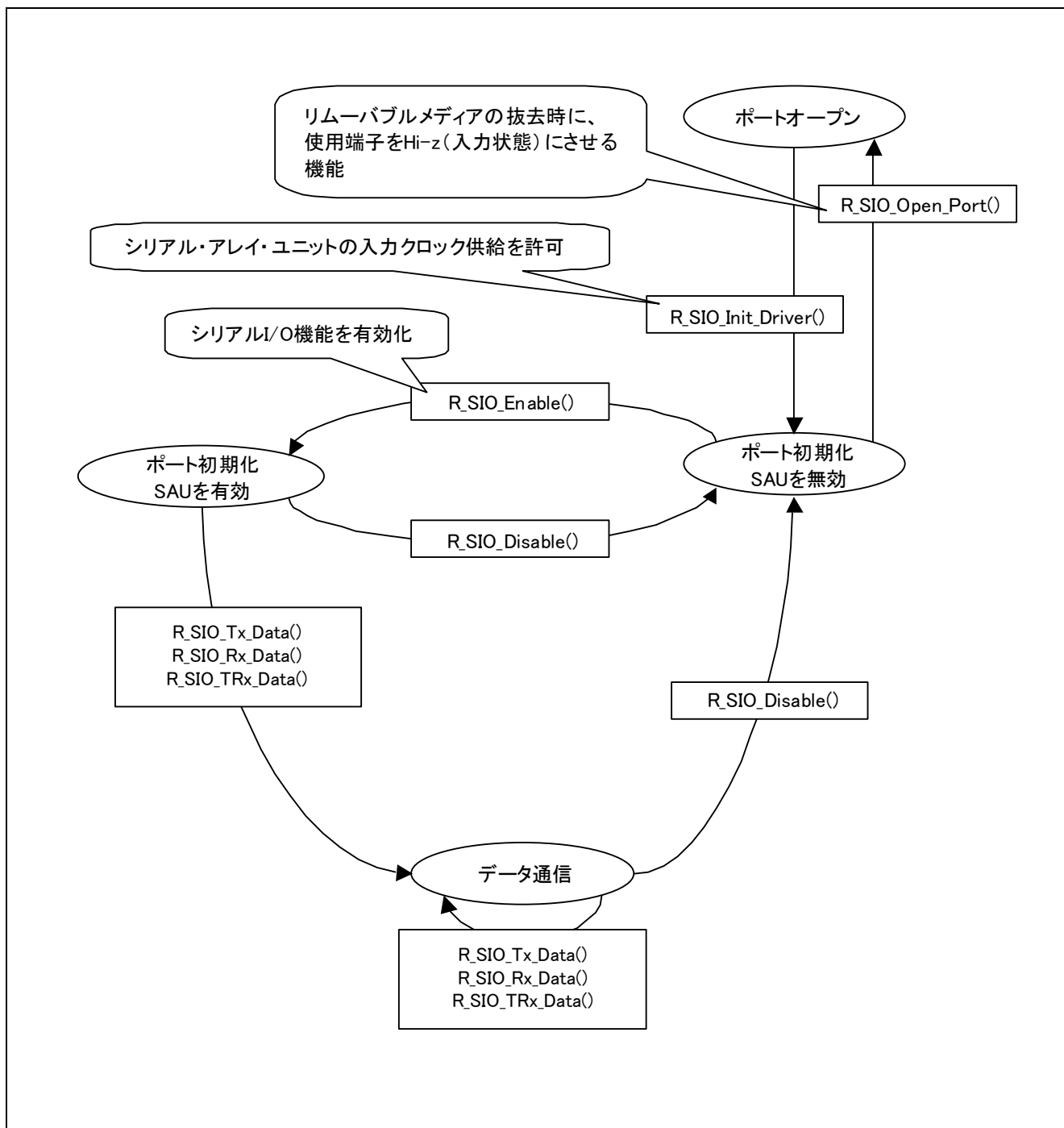
図 5-11 状態遷移図
