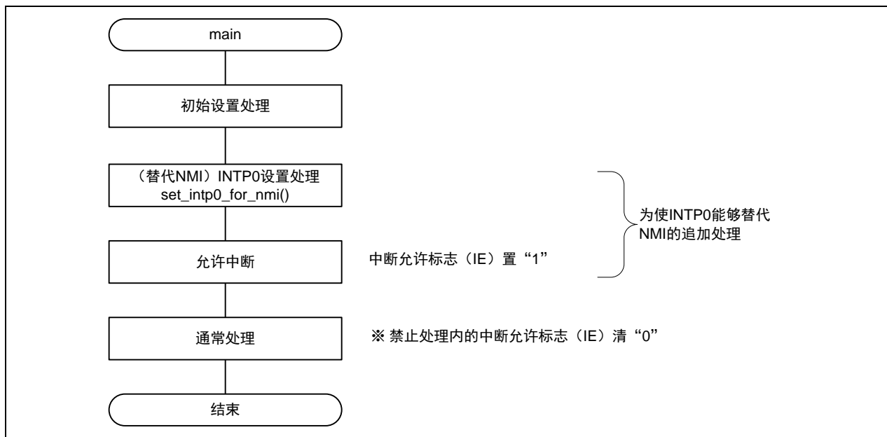
图 3.3 以 INTPO 替代 NMI 中断时的主函数处理流程
