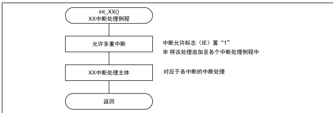
图 3.2 以 INTPO0 替代 NMI 中断时的 INTPO0 中断以外的中断处理流程
