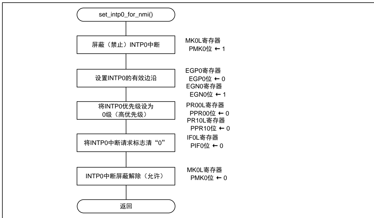
图 3.1 替代 NMI 中断的 INTPO0 设置处理流程
