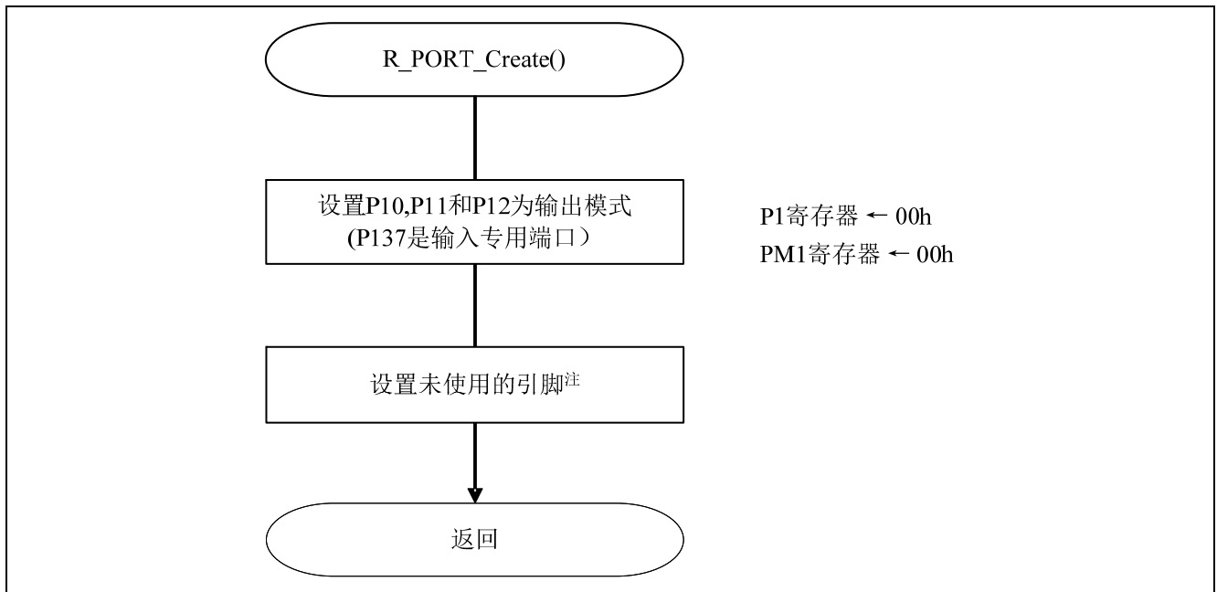
图 5.5 I/O 端口设置
