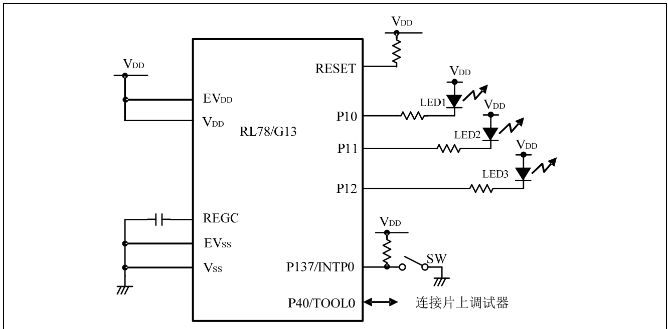
图 4.1 硬件配置
