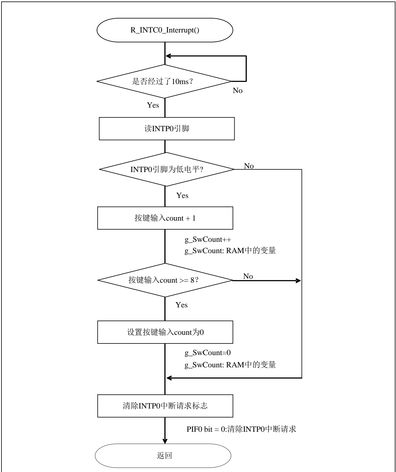
图 5.10 INTPO 中断处理
