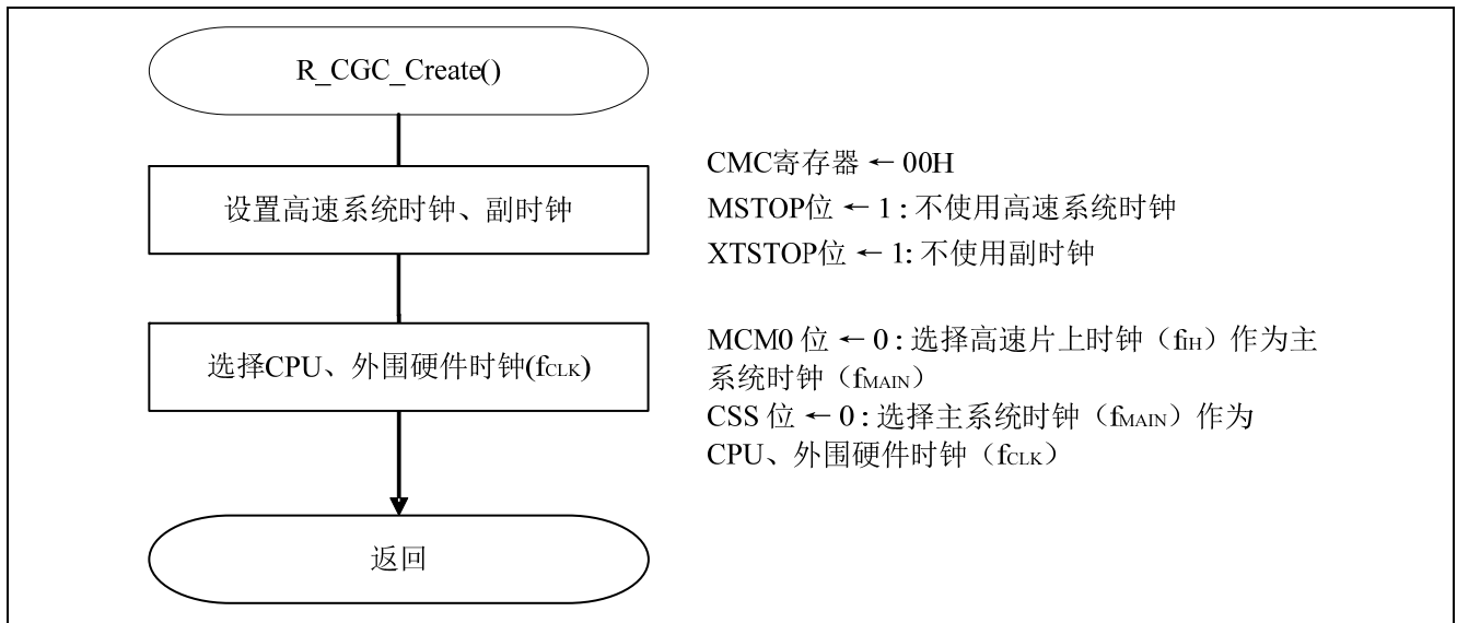
图 5.6 CPU 时钟的设置
