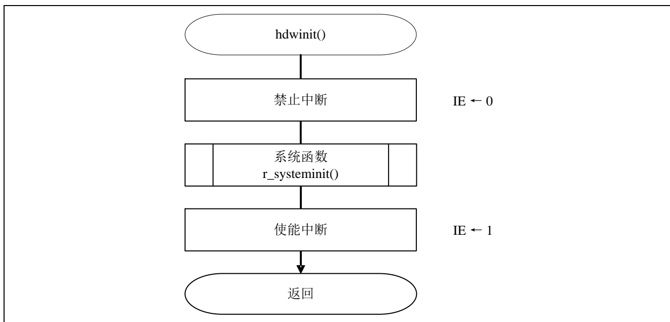
图 5.3 初始化函数
