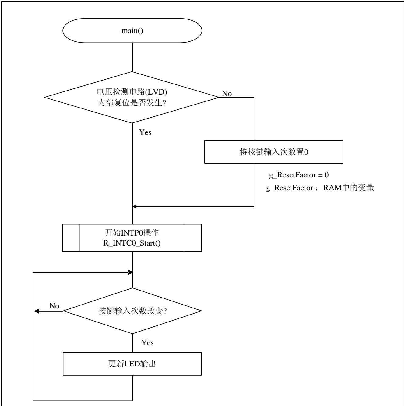
图 5.8 主函数处理
