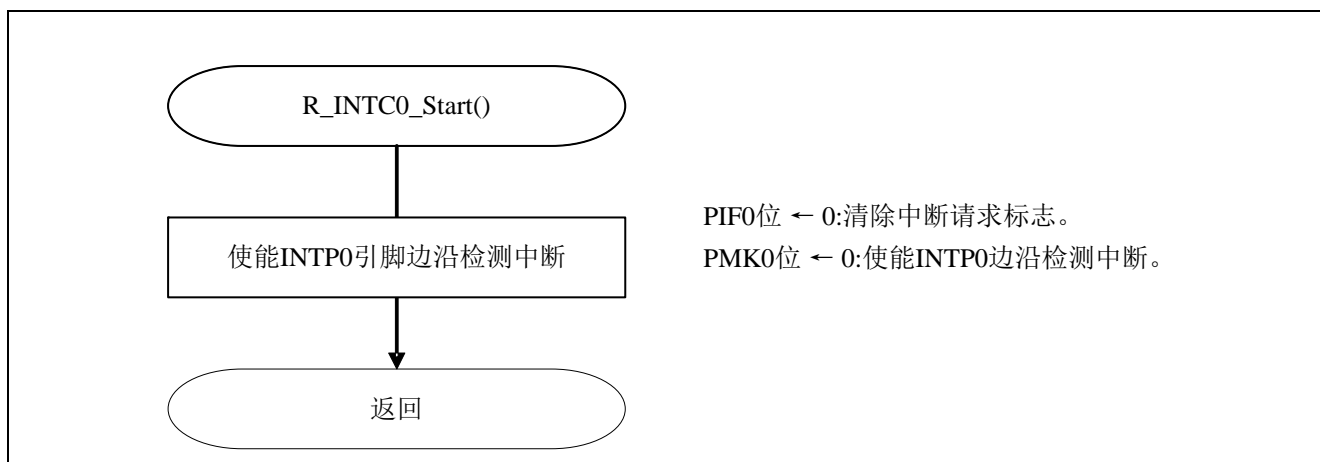
图 5.9 开始 INTP0 操作
