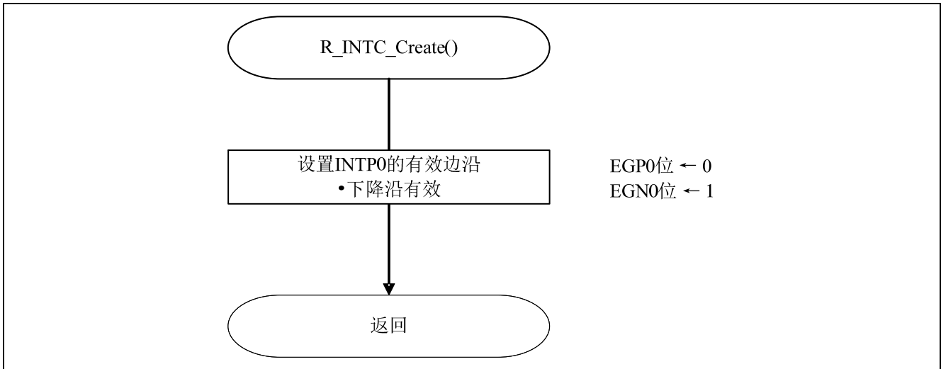
图 5.7 初始化 INTP0
