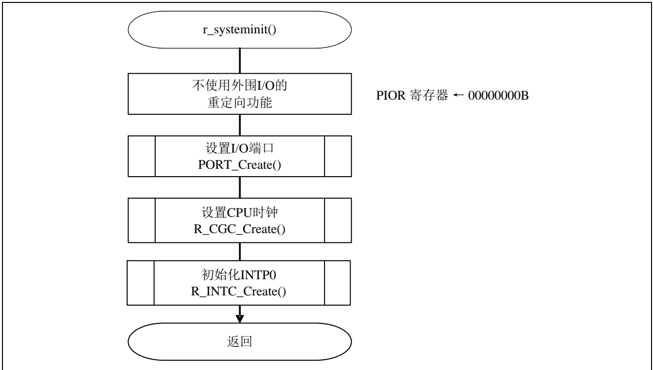
图 5.4 系统函数
