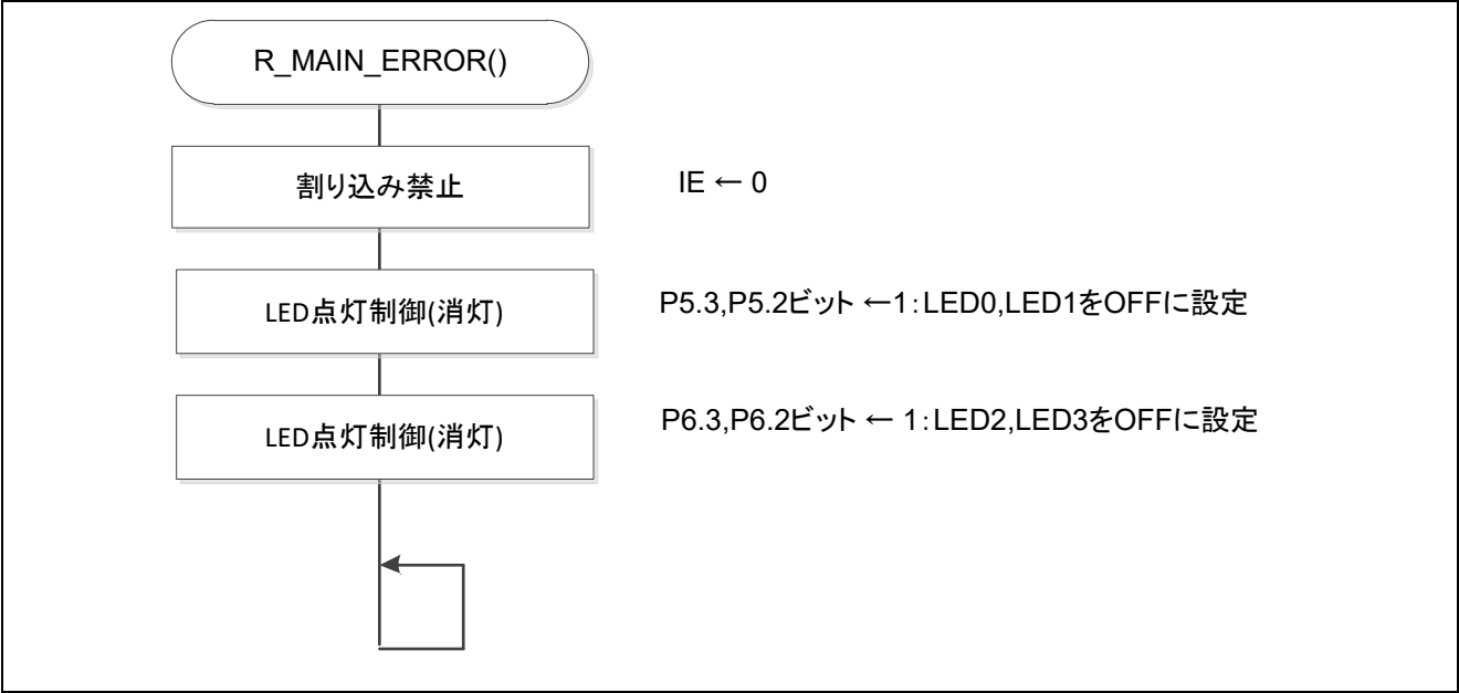
図 5.14 状態移行エラー処理
