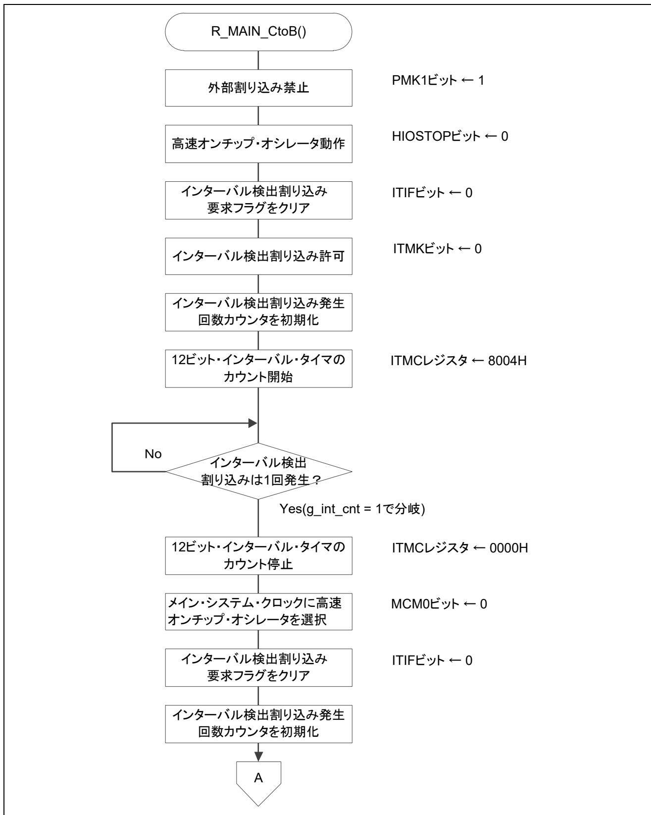
図 5.29 状態移行 CtoB(1/2)
