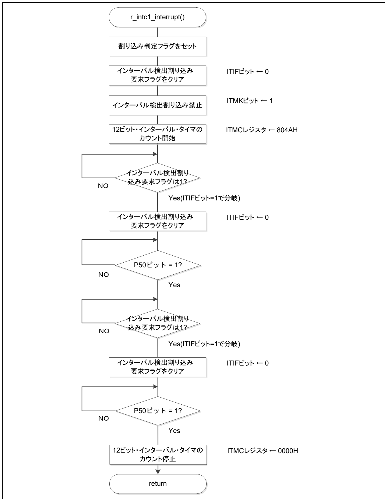
図 5.39 外部割り込み処理
