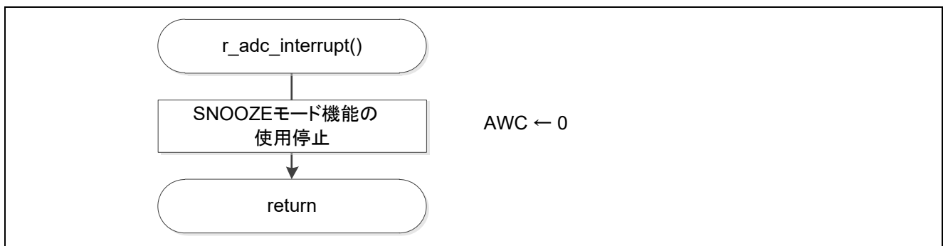
図 5.41 A/D 変換終了割り込み処理
