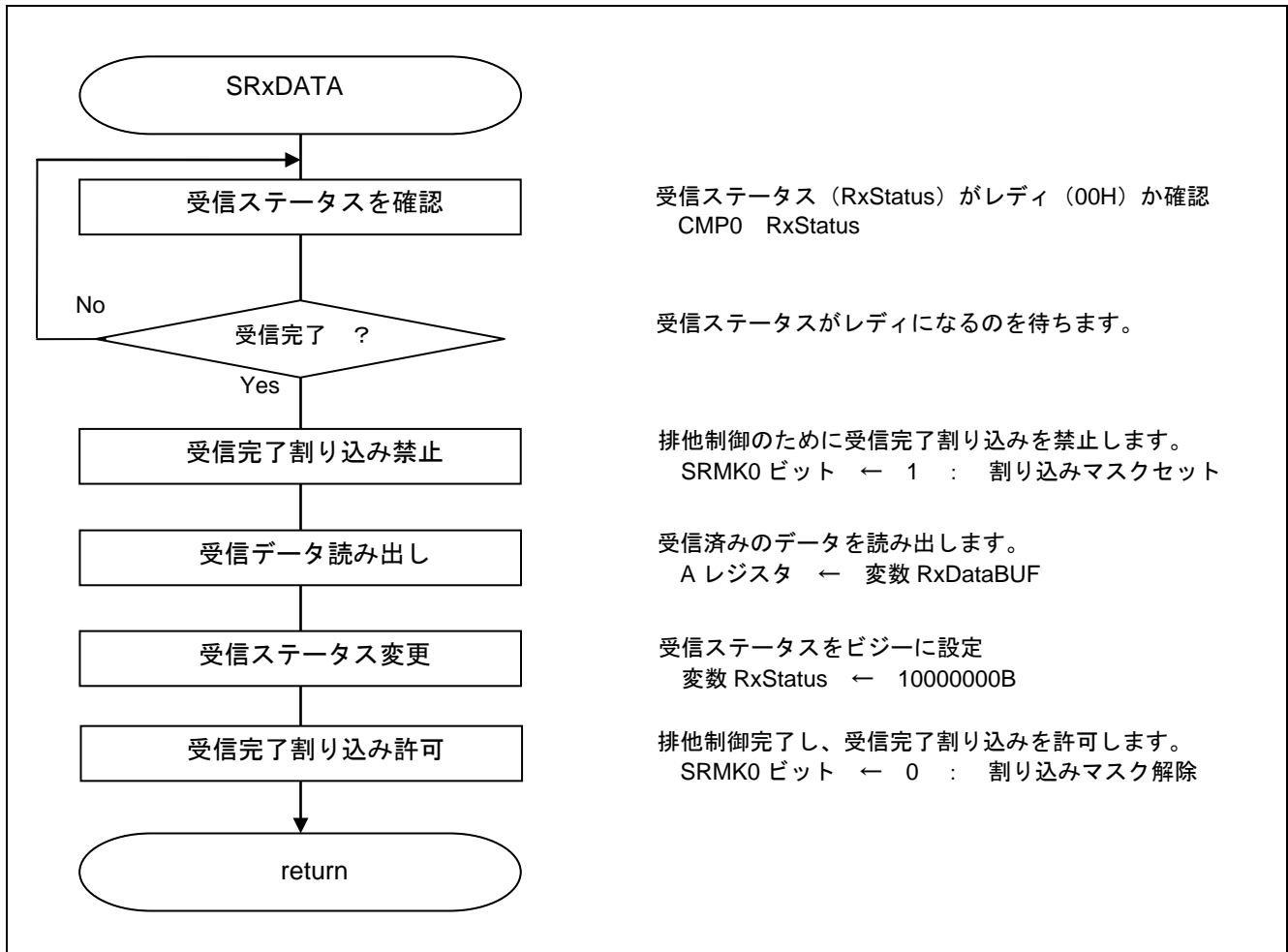
図 5.14 1 キャラクタ受信処理
