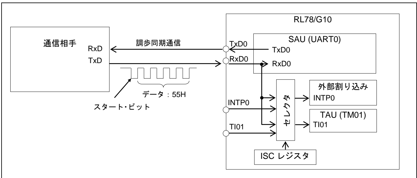
図 1.1 ボー・レート測定の構成
