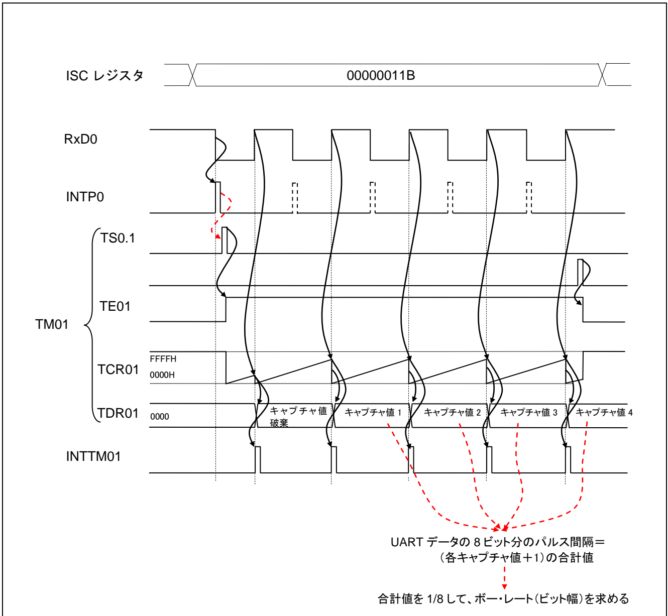
図 1.2 ボー・レート測定のタイミングチャート
