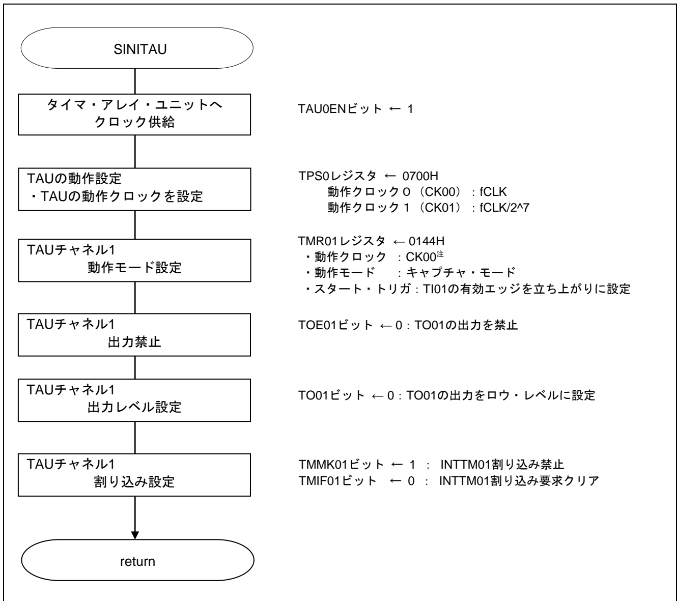
図 5.5 タイマ・アレイ・ユニットの設定
