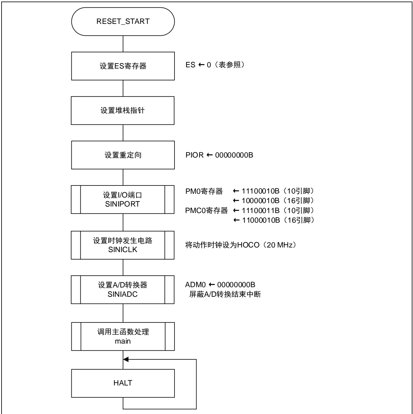
图 5.2 CPU 初始化函数
