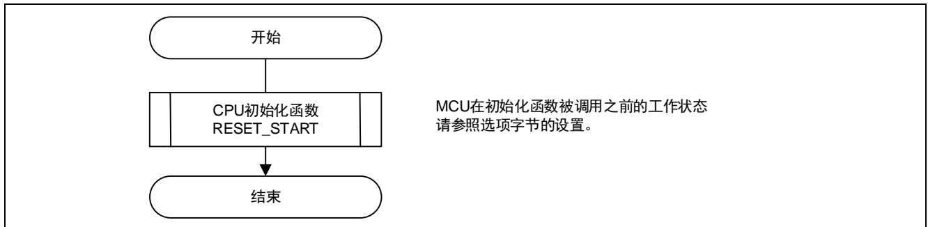
图 5.1 整体流程图
