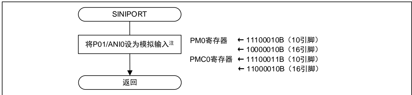
图 5.3 设置 I/O 端口的函数
