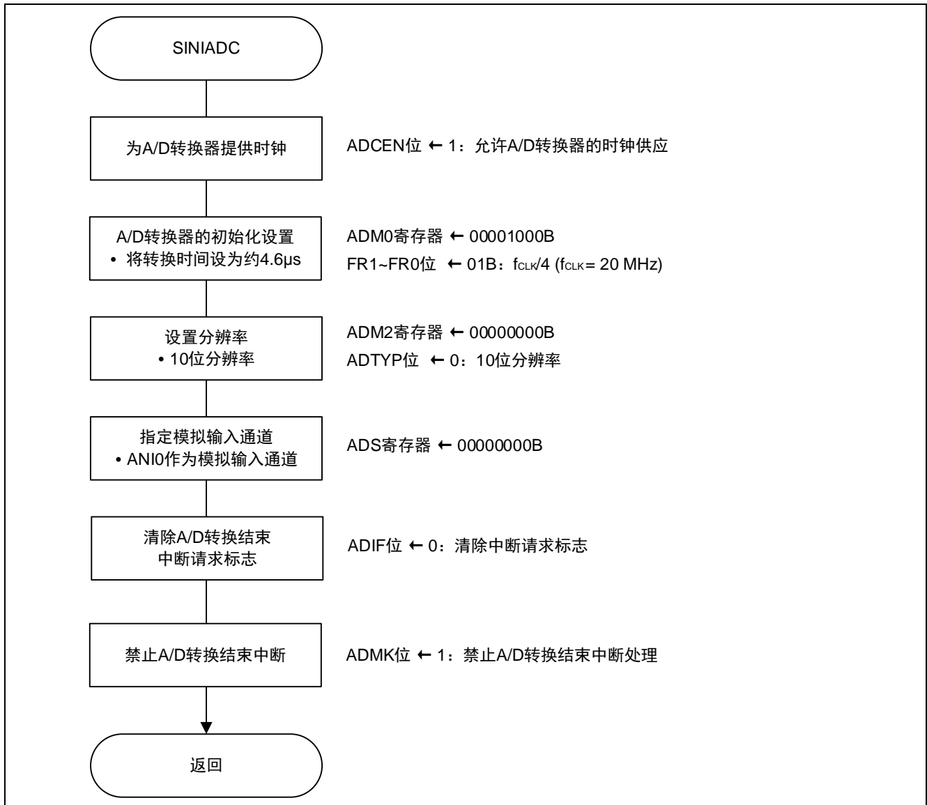
图 5.5 设置 A/D 转换器
