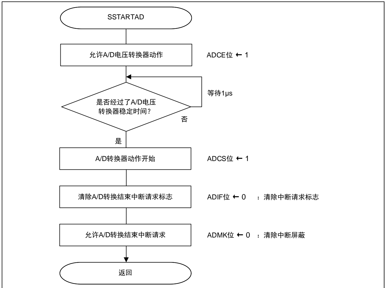
图 5.7 A/D 转换开始处理
