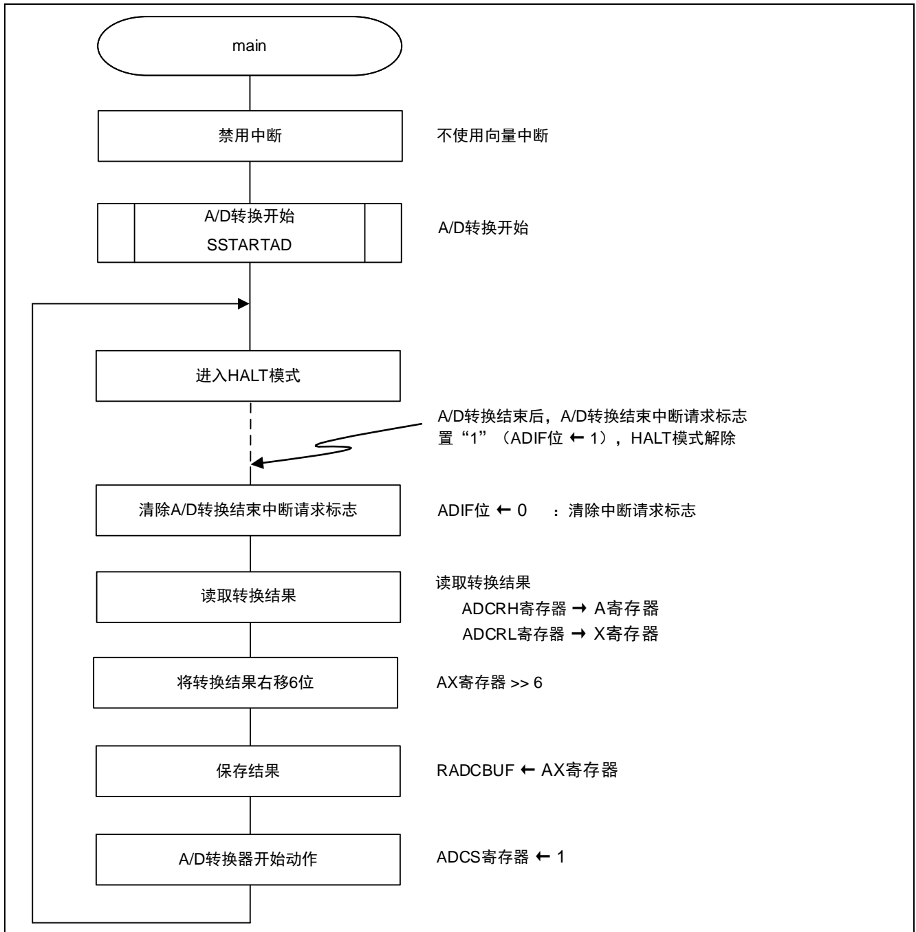
图 5.6 主函数处理
