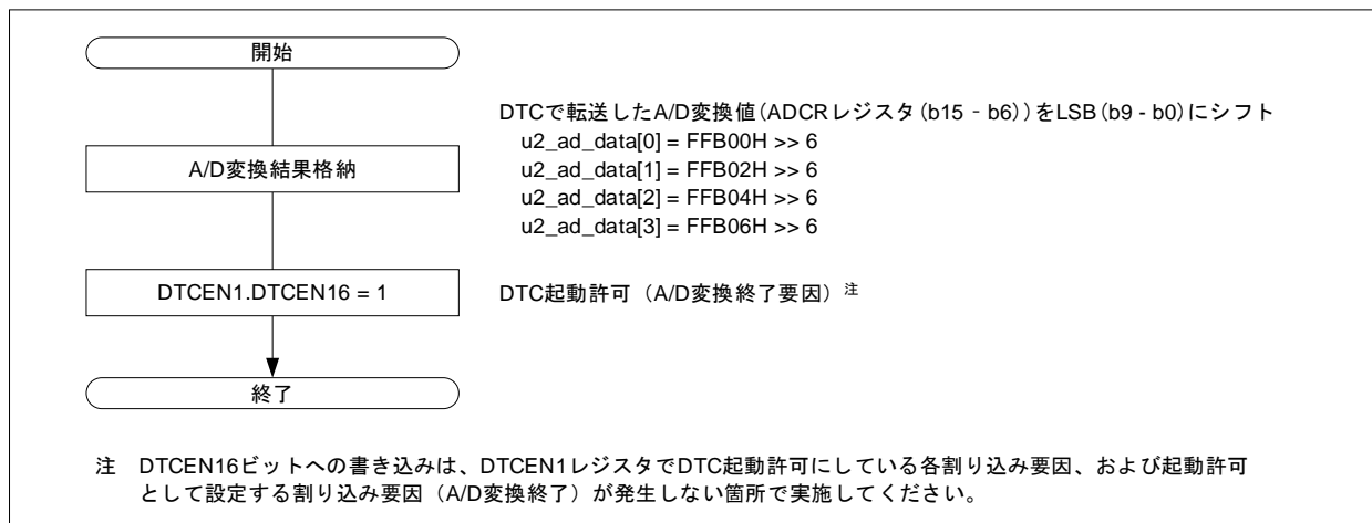
図 3.6 DTC 転送完了割り込み処理（A/D 変換終了割り込み）
