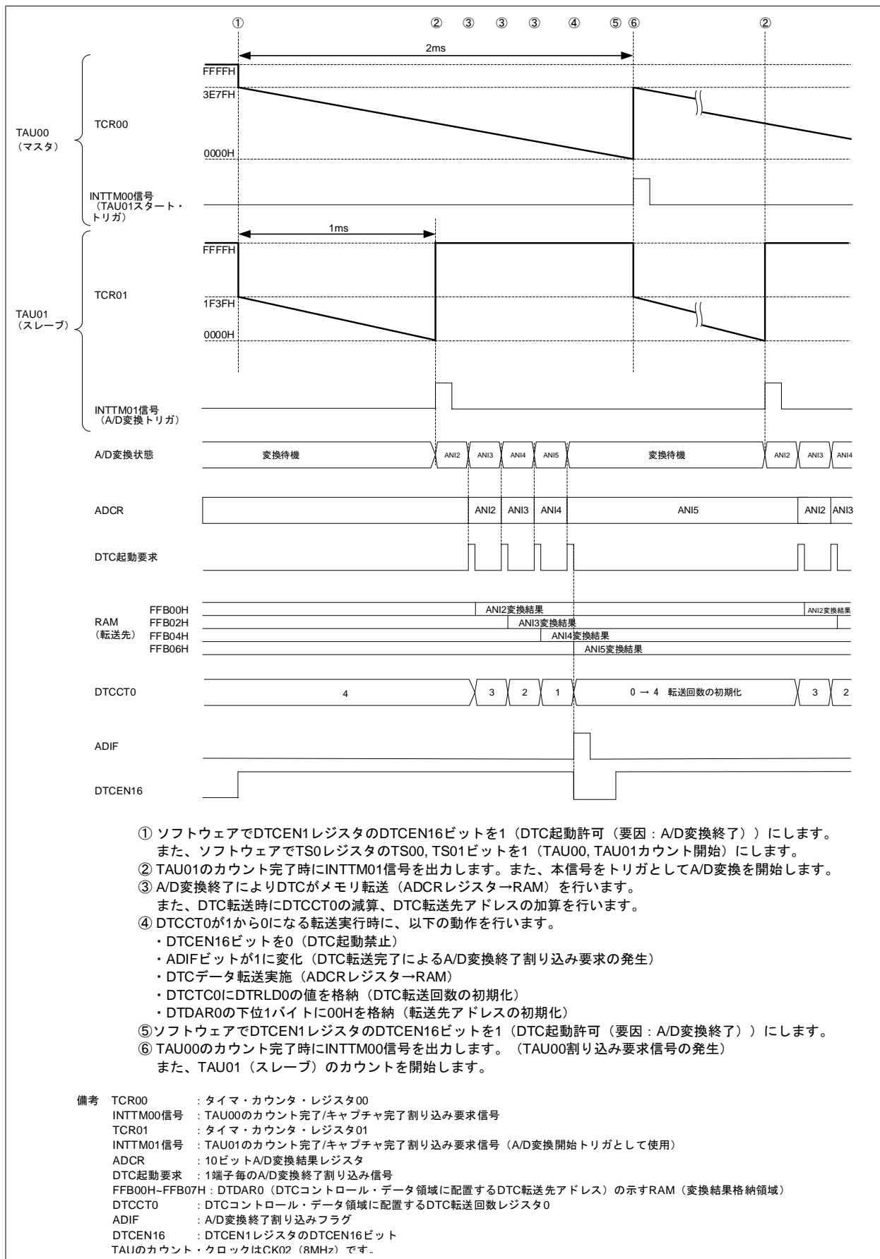
図 2.3 DTC 転送タイミング
