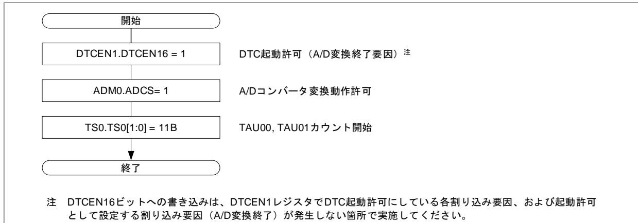
図 3.5 周辺機能の動作許可（DTC 転送開始）手順
