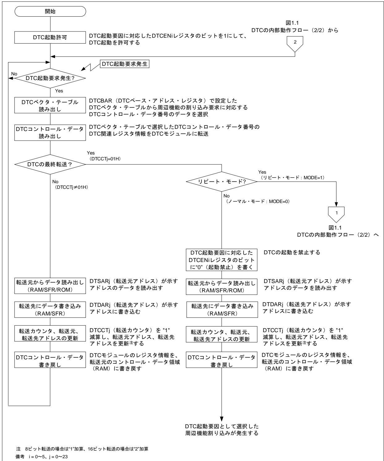
図 1.1 DTC の内部動作フロー (1/2)
