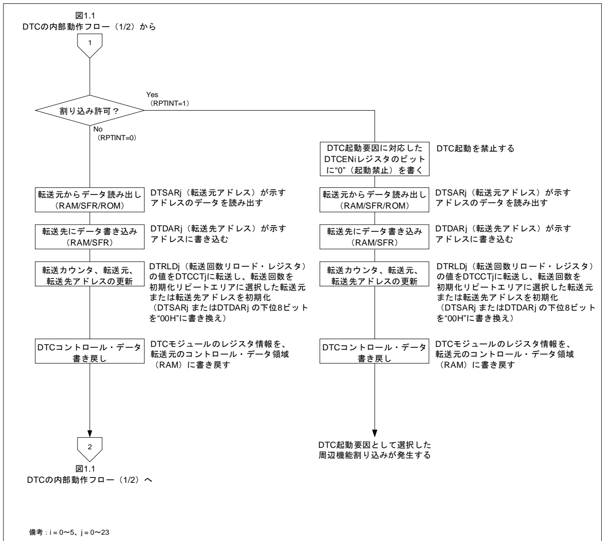
図 1.1 DTC の内部動作フロー (2/2)
