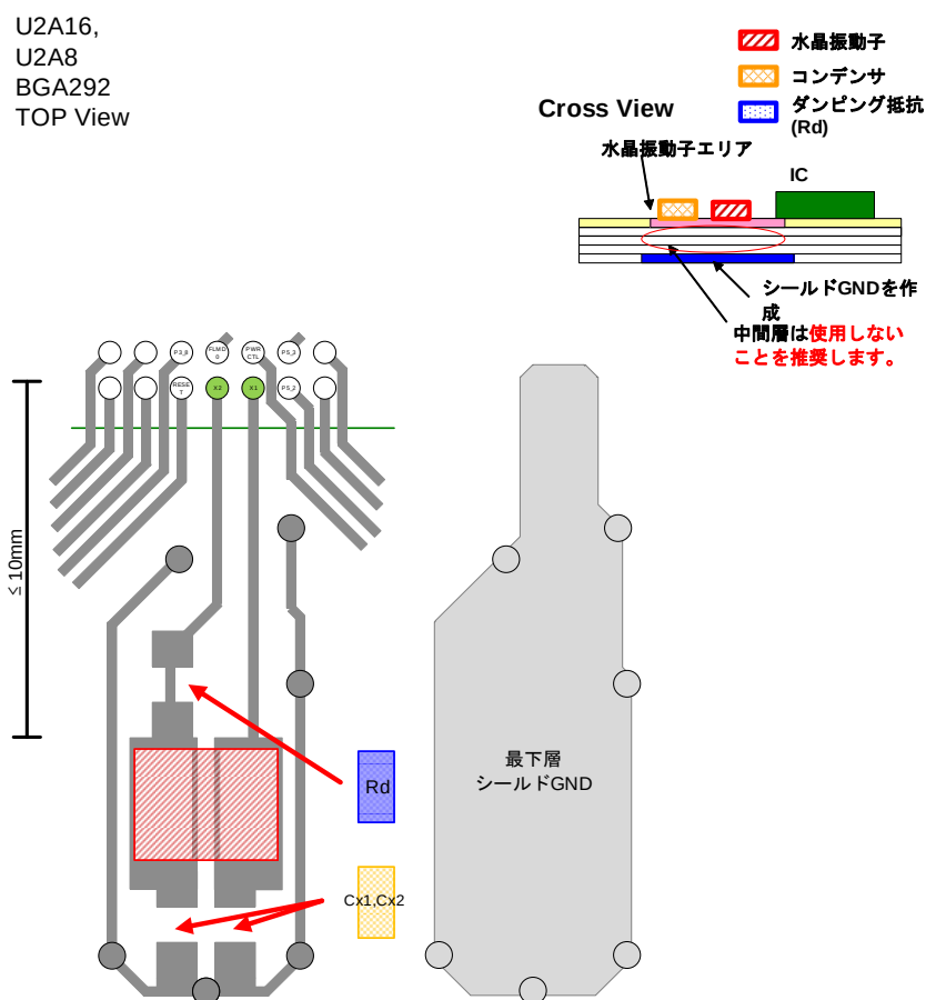
図. 5 安定発振のためのボードパターン例 (U2A16,U2A8 BGA292の場合)
