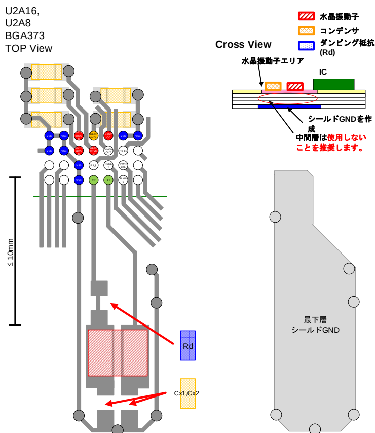
図. 4 安定発振のためのボードパターン例 (U2A16,U2A8 BGA373の場合)
