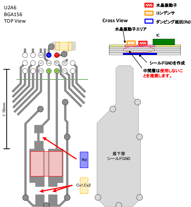
図. 7 安定発振のためのボードパターン例 (U2A6 BGA156の場合)
