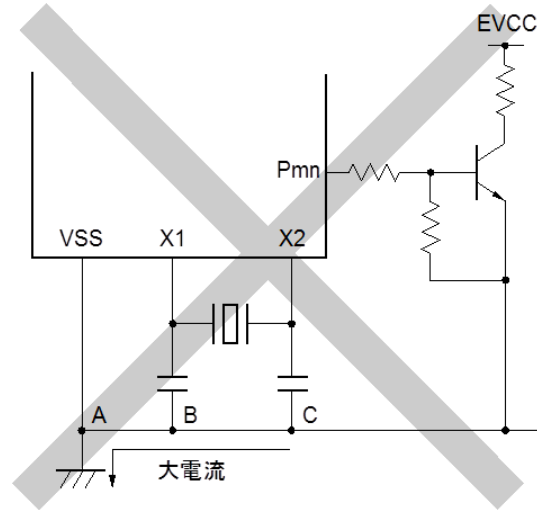
(f) 発振回路部のグランド・ライン上に電流が流れる (A点、B点、C点の電位が変動する)
