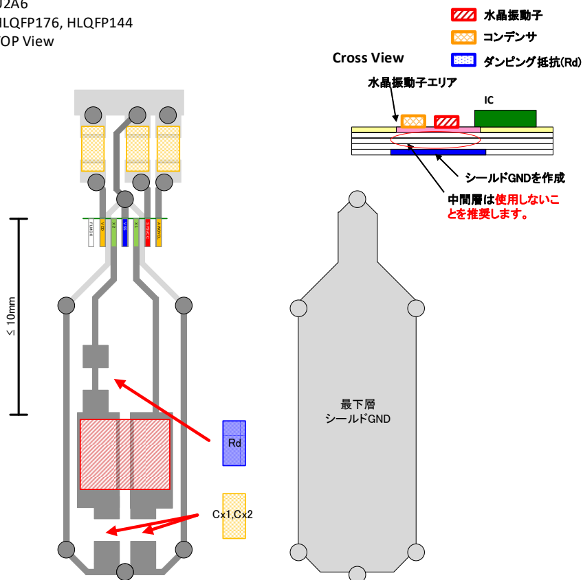
図. 6 安定発振のためのボードパターン例 (U2A6 QFP176, QFP144の場合)
