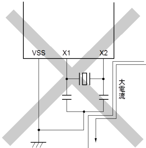
(e) 変化する大電流が信号線に近接している
