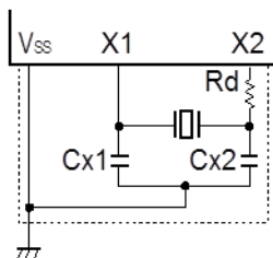
図. 10 外付け回路例
