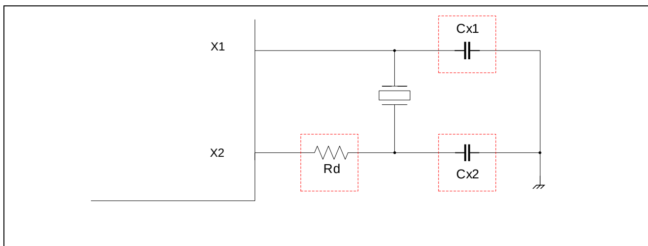
図. 1 水晶振動子の接続推奨回路
