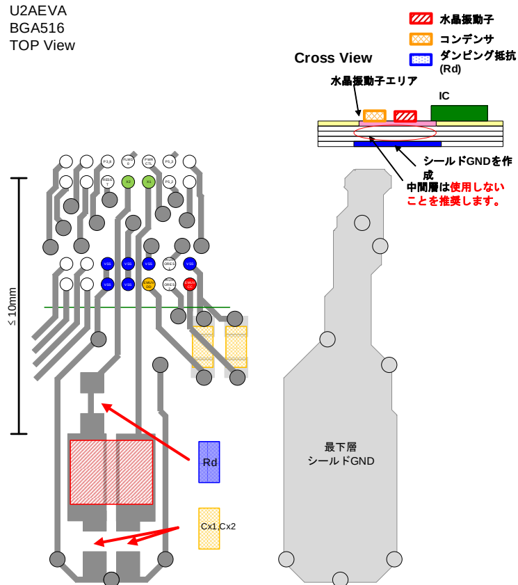
図. 2 安定発振のためのボードパターン例 (U2A-EVA BGA516の場合)
