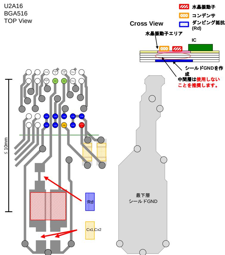
図. 3 安定発振のためのボードパターン例 (U2A16 BGA516の場合)
