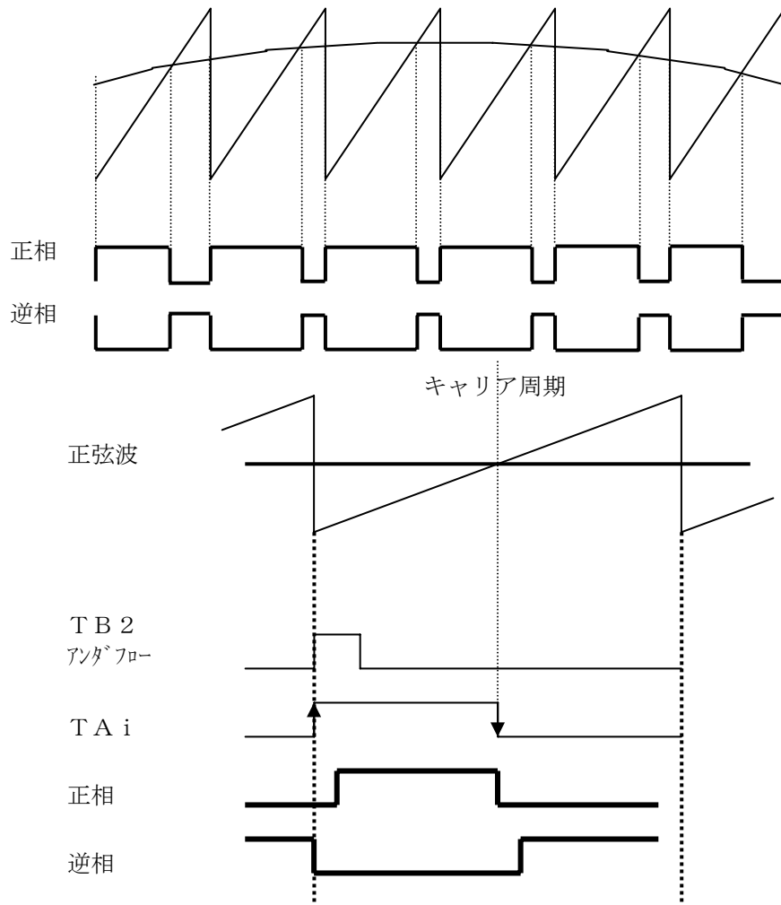
図 3.2.4 短絡防止時間を設定した場合の鋸波変調時のタイマとPWMの関係
