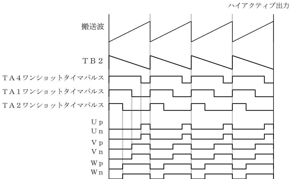
図 3.1.3 三相モード0（鋸波変調）
