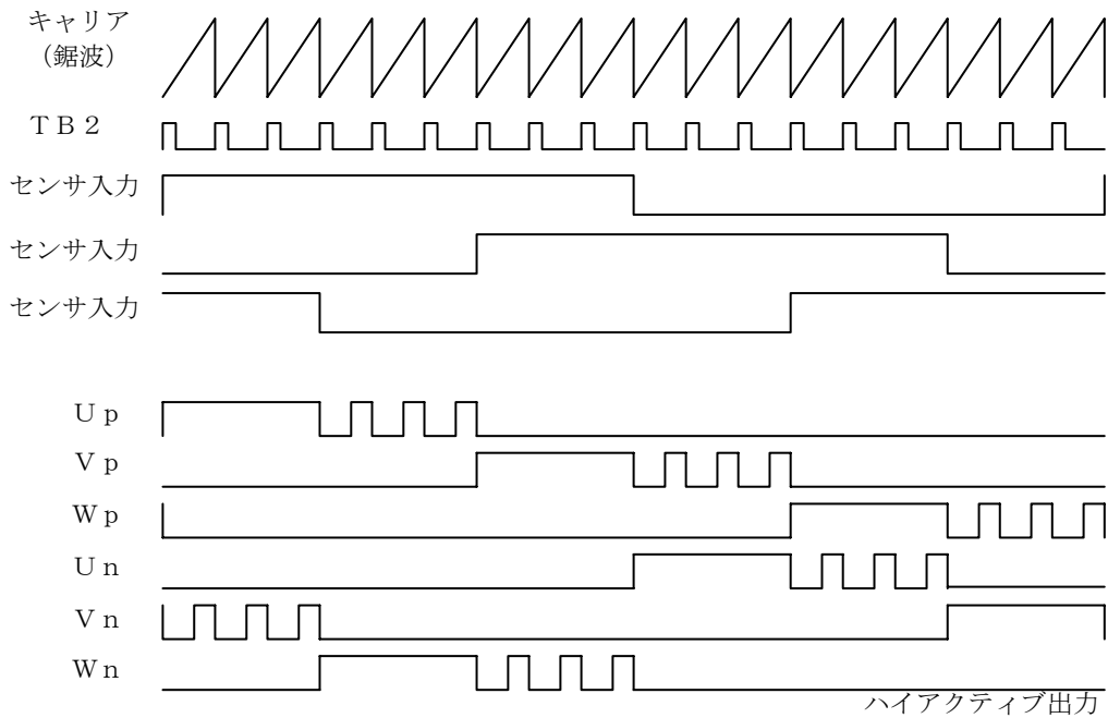
図 3.2.5 120° 通電矩形波駆動のセンサ入力と波形出力の関係
