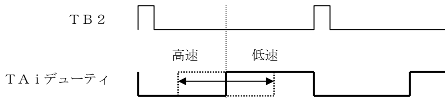
図 3.2.7 回転数指令値とTAiの関係
