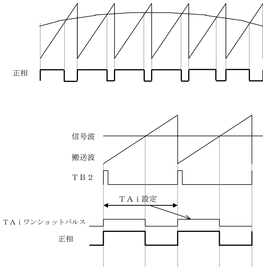
図 3.2.3 鋸波変調時のタイマとPWMの関係
