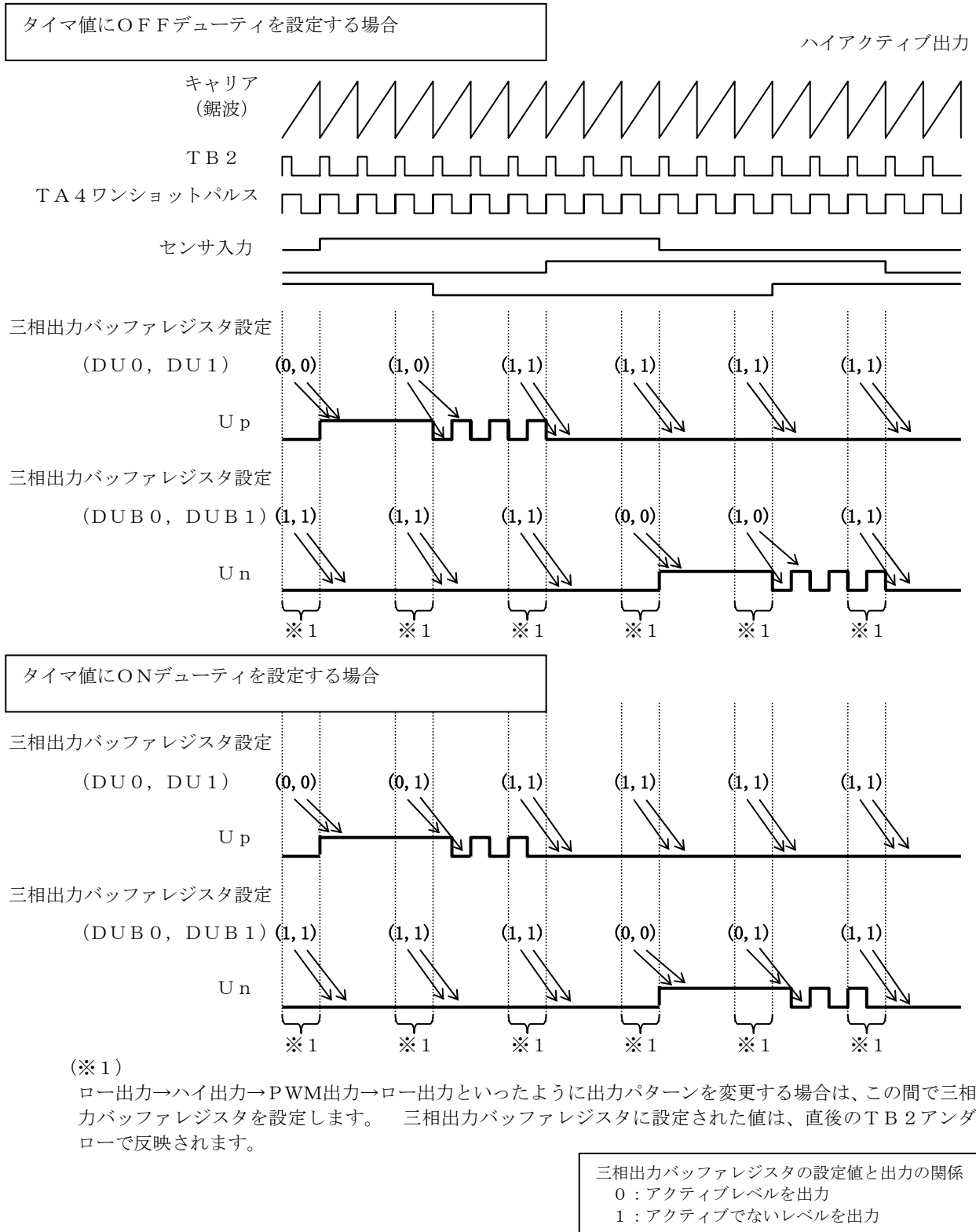
図 3.2.6 三相出力バッファレジスタの設定方法
