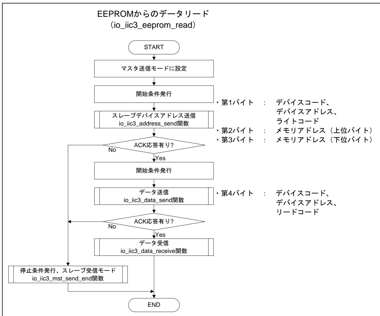
図11 参考プログラムの処理フロー (6)
