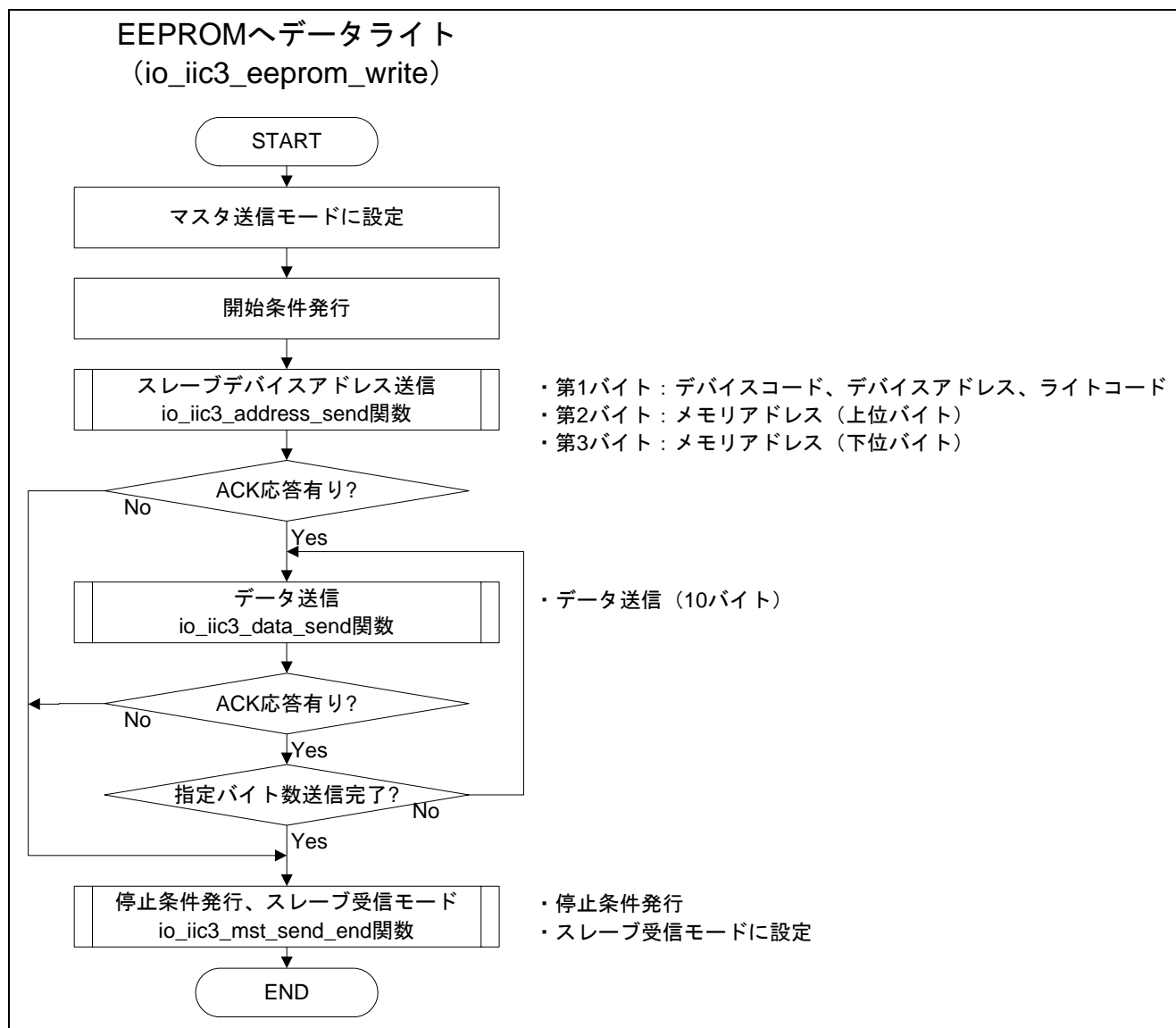
図7 参考プログラムの処理フロー（2）
