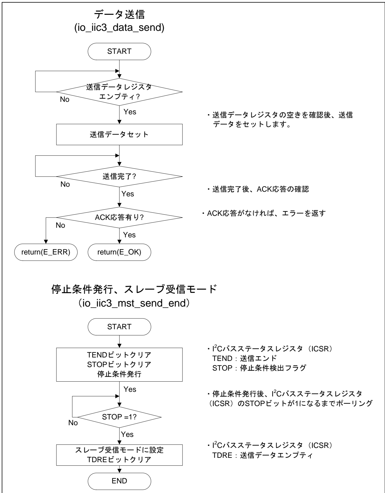
図9 参考プログラムの処理フロー (4)
