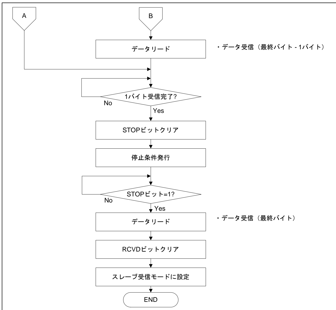
図13 参考プログラムの処理フロー (8)
