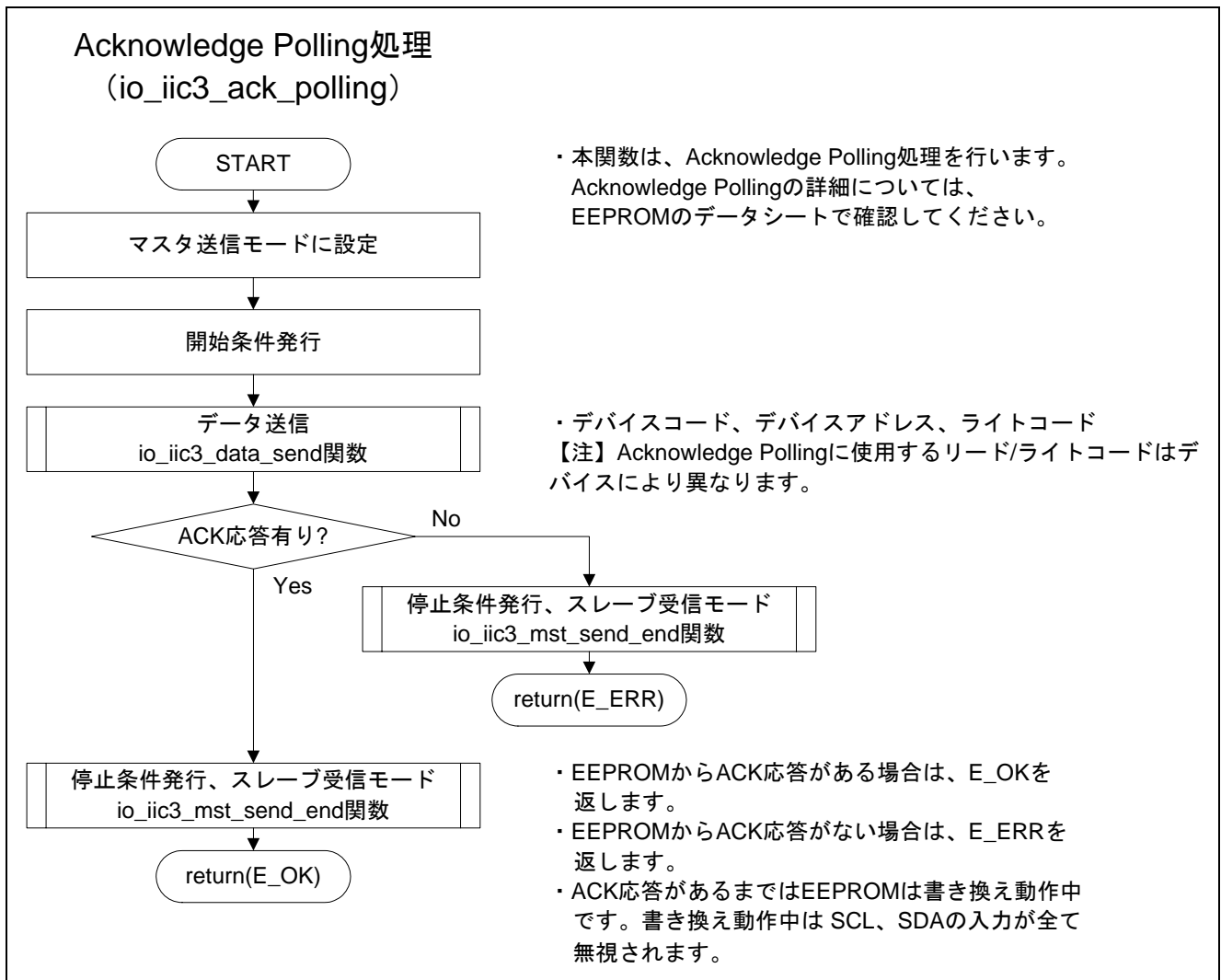
図10 参考プログラムの処理フロー (5)
