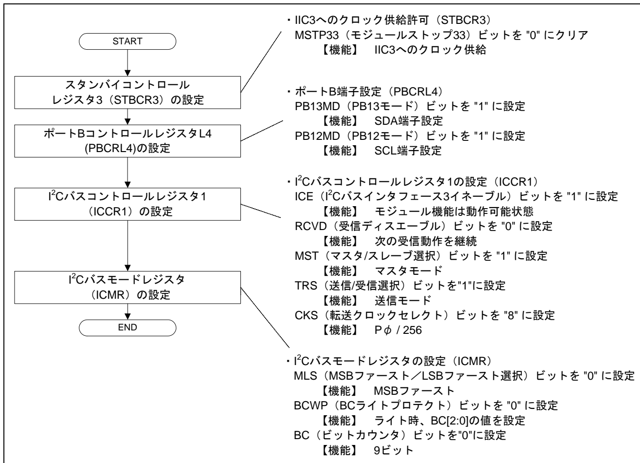
図2 IIC3 の初期設定フロー例
