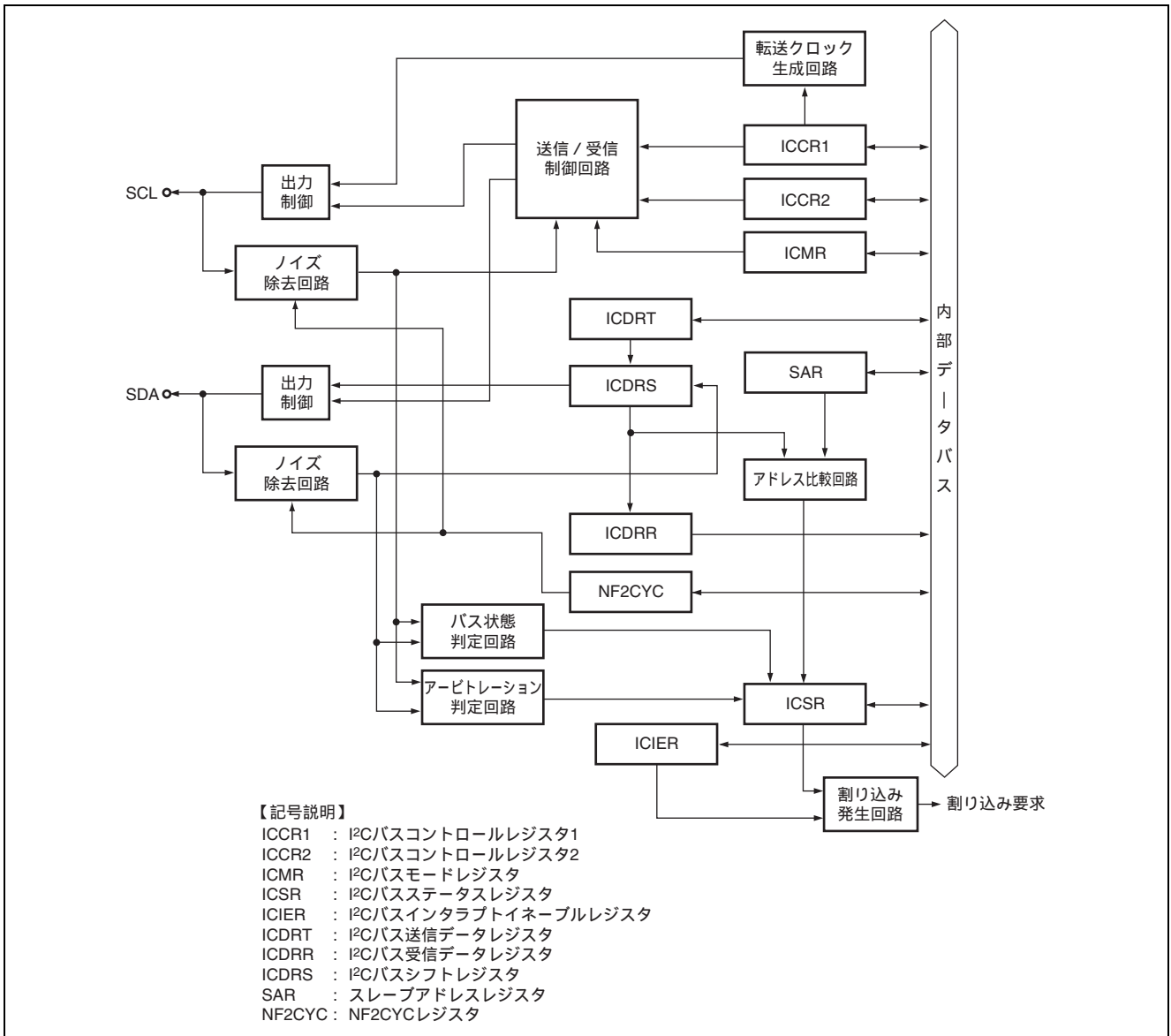
図1 IIC3 のブロック図
