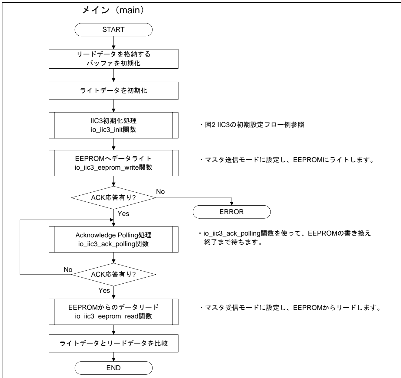
図6 参考プログラムの処理フロー (1)
