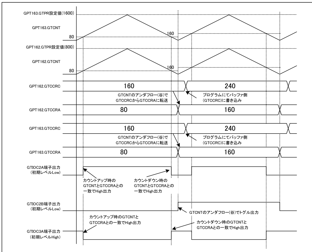
図 1.1 GPT 出力波形（GPT162、163 のみ）
