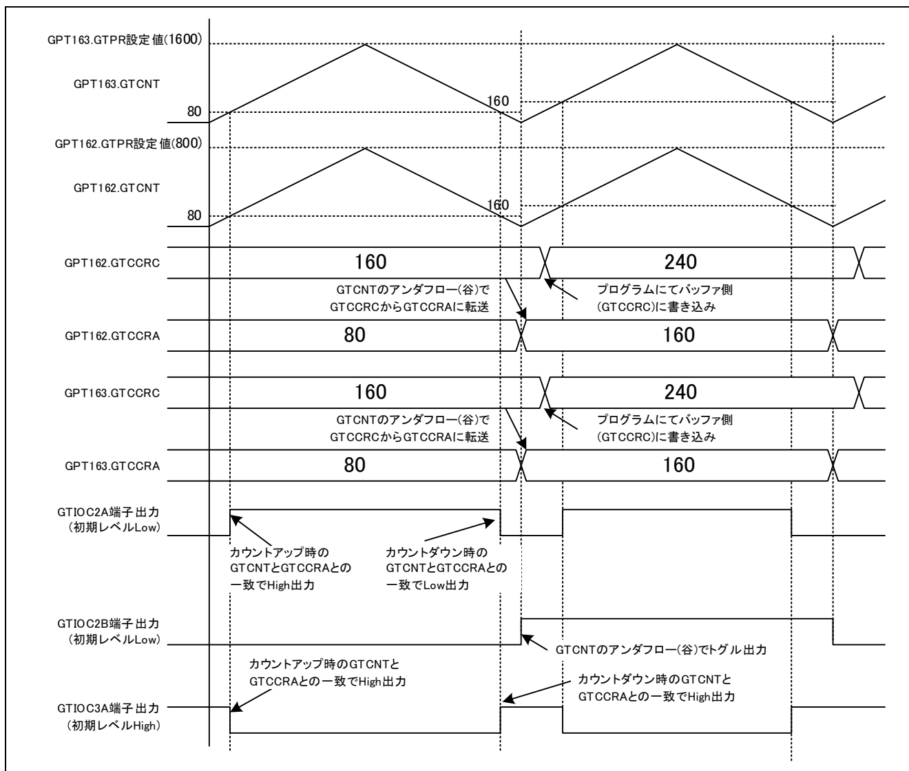
図 1.1 GPT 出力波形 (GPT162、163 のみ)
