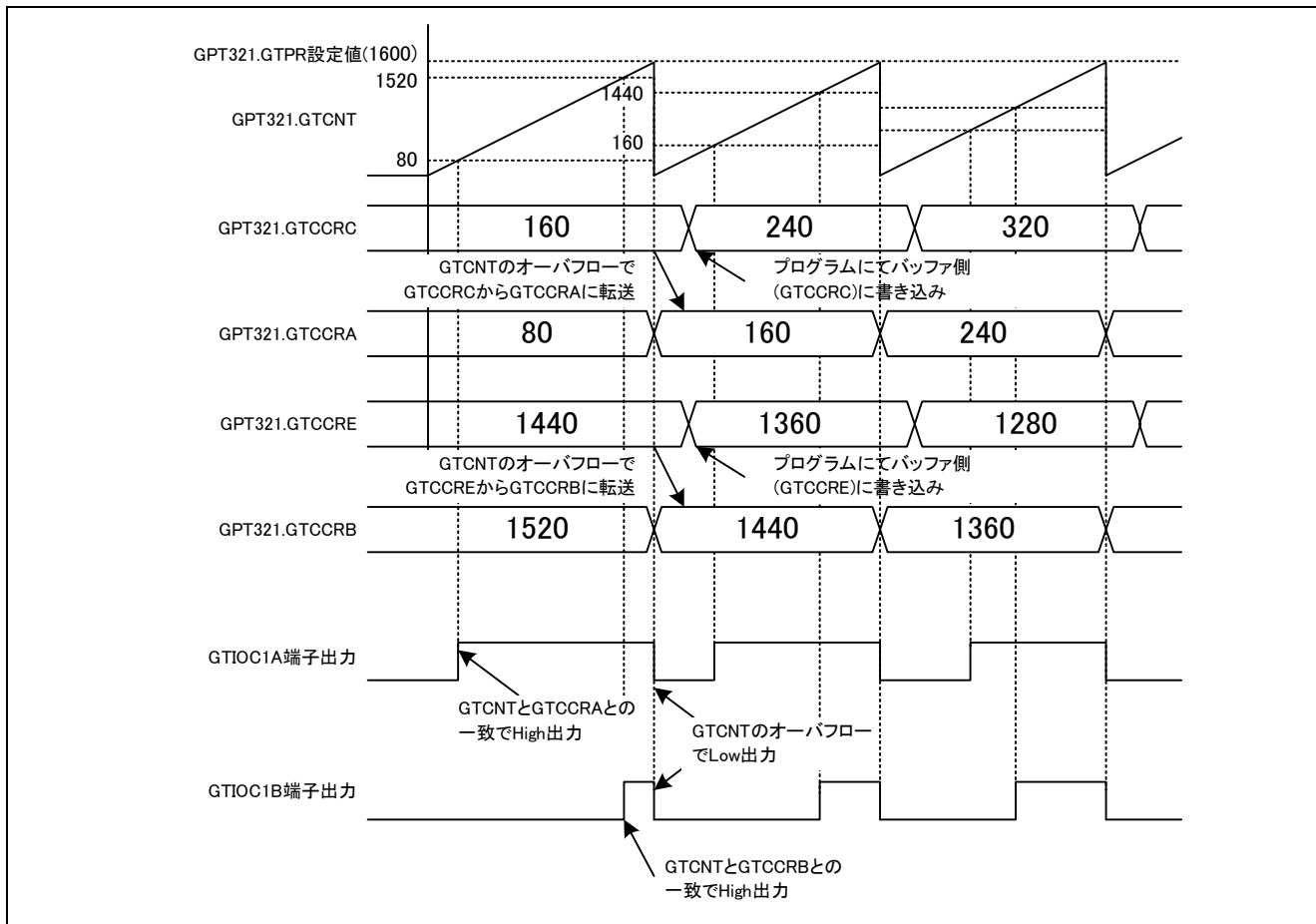
図 1.1 GPT 出力波形
