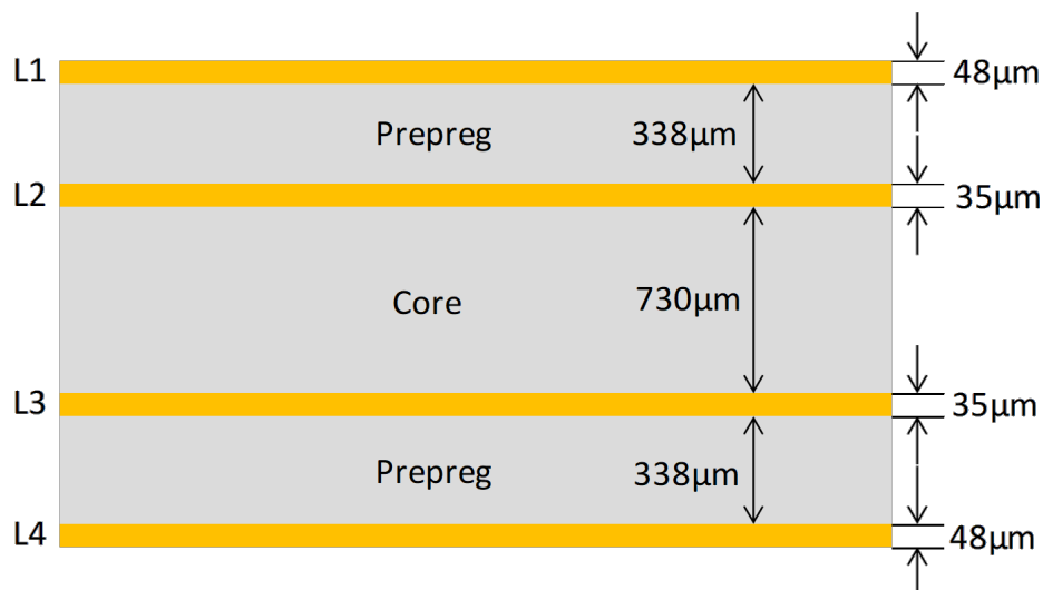
図 2 基板層構成
