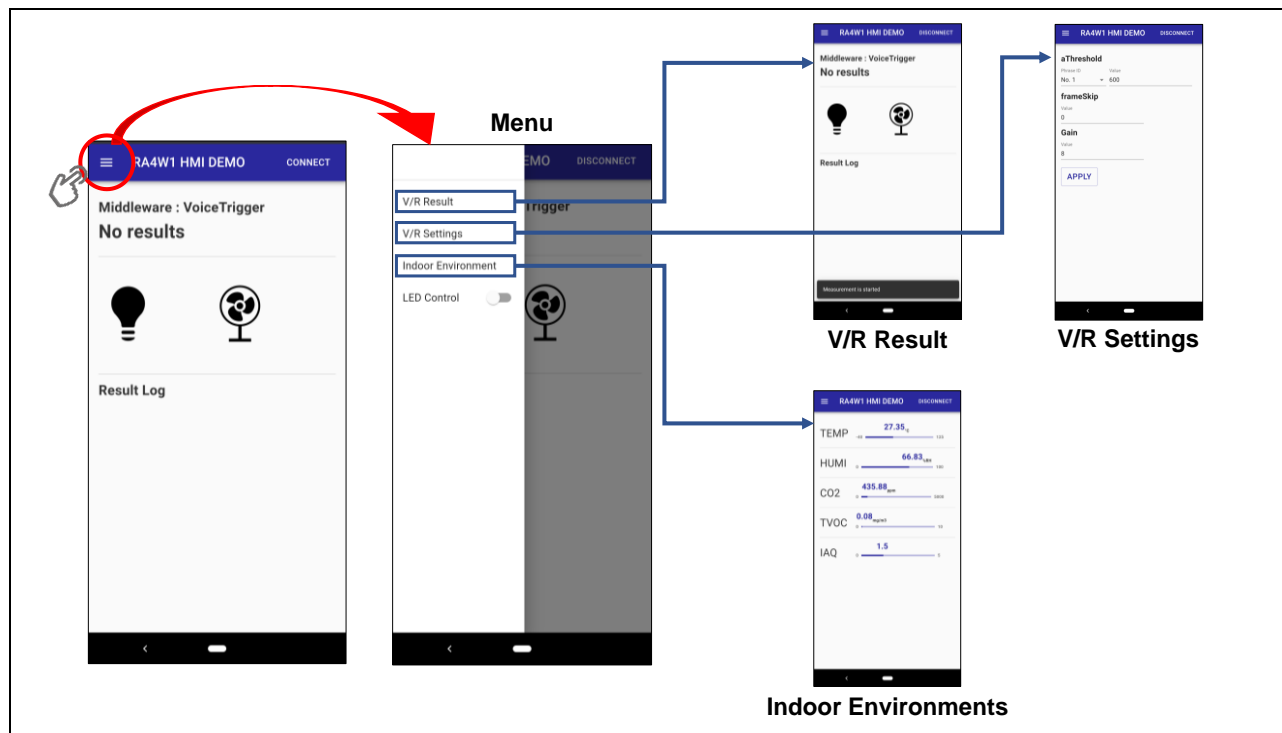
図 3.2 画面遷移
