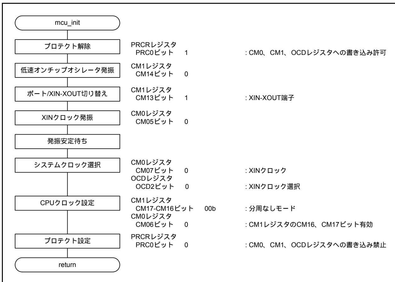
図 3.3 システムクロック設定処理
