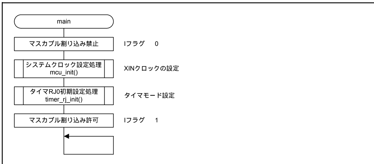
図 3.2 メイン処理
