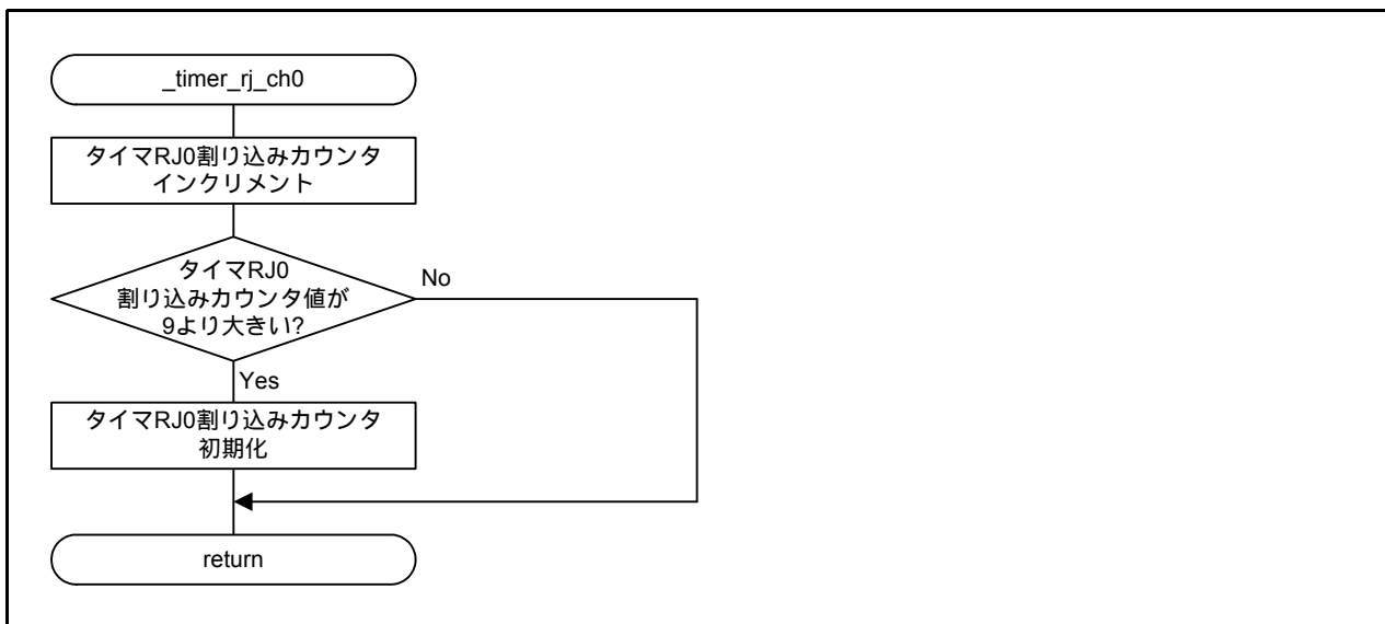
図 3.5 タイマRJ0 割り込み処理
