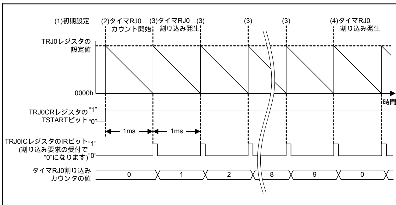
図 3.1 タイミング図
