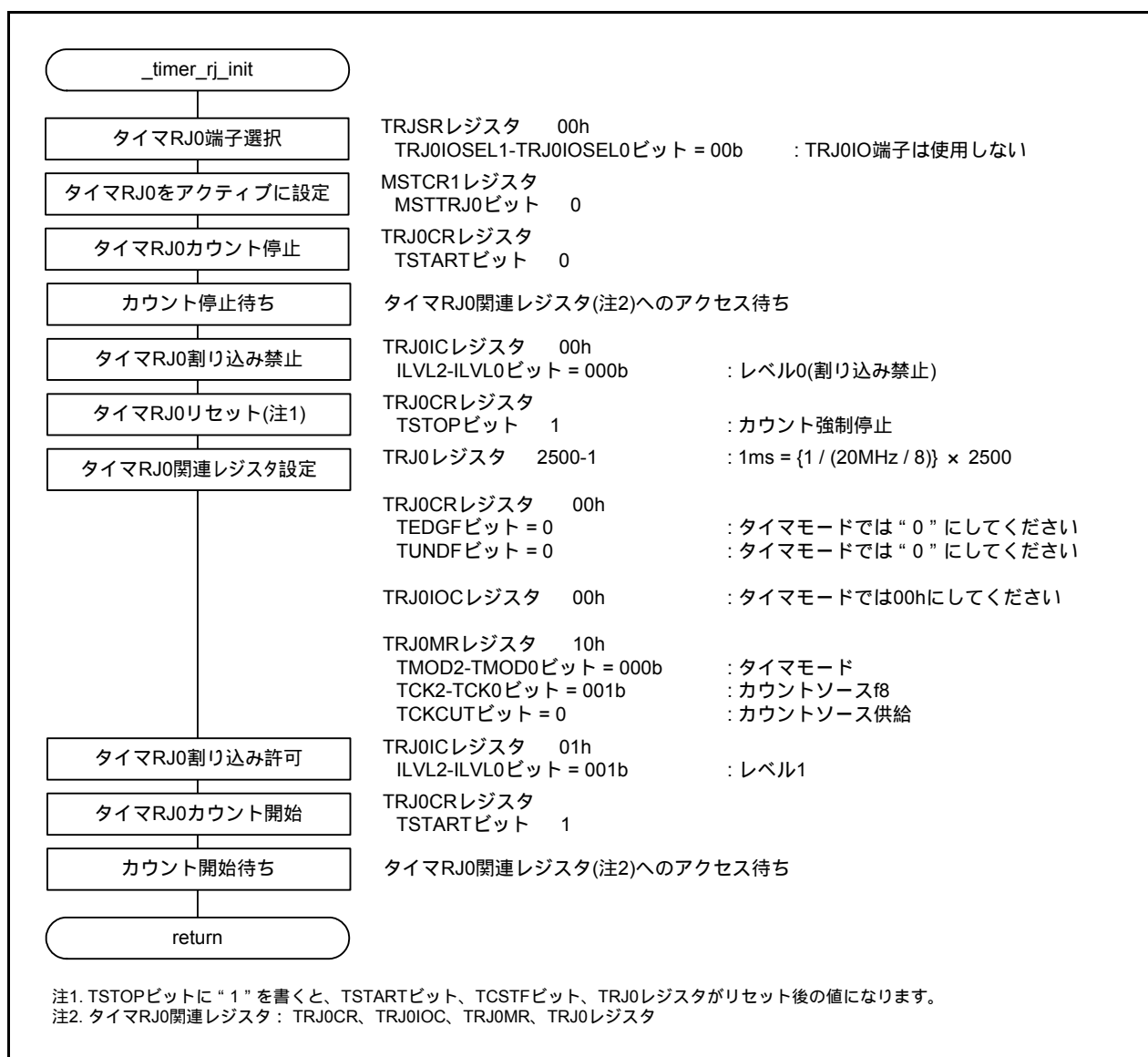
図 3.4 タイマRJ0初期設定処理
