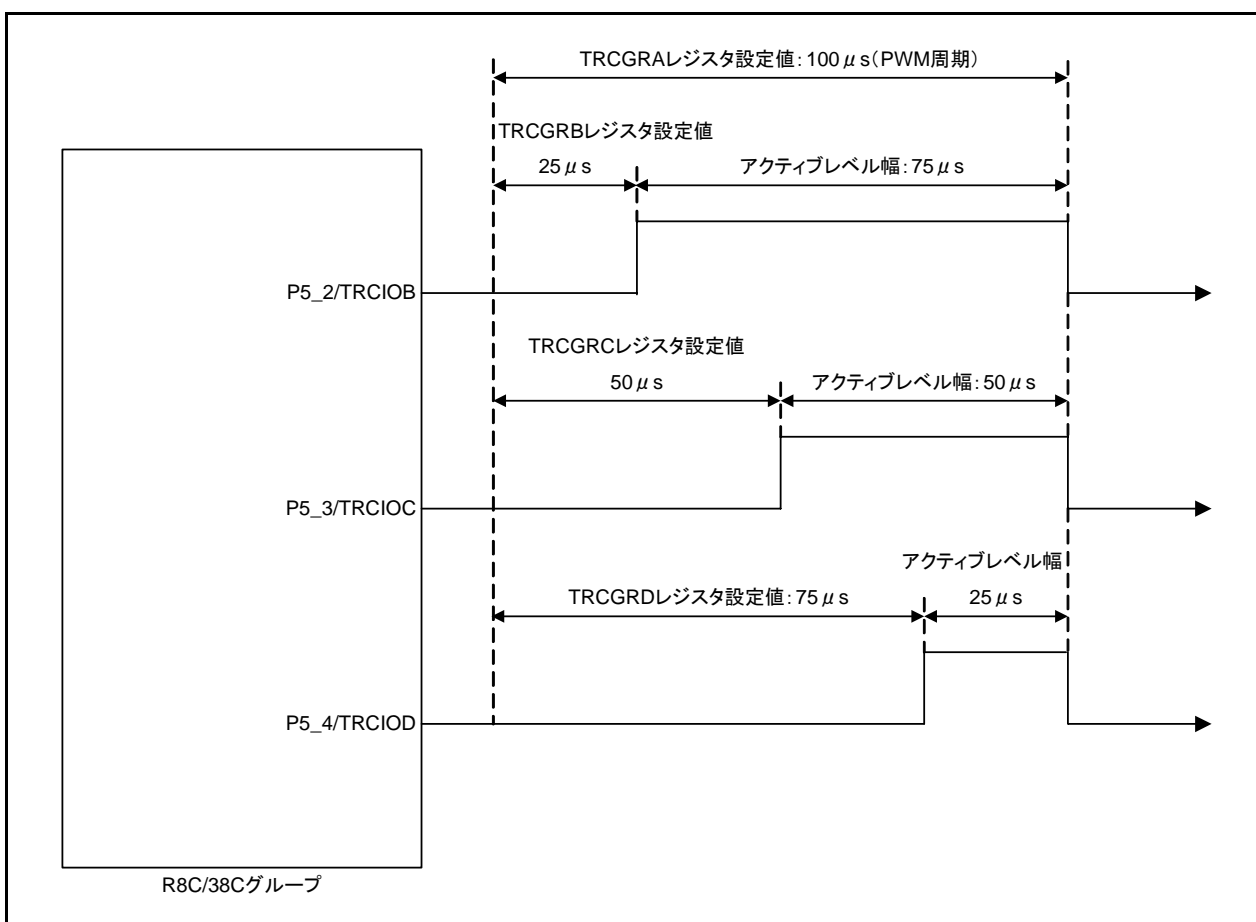
図 3.2 タイミング図
