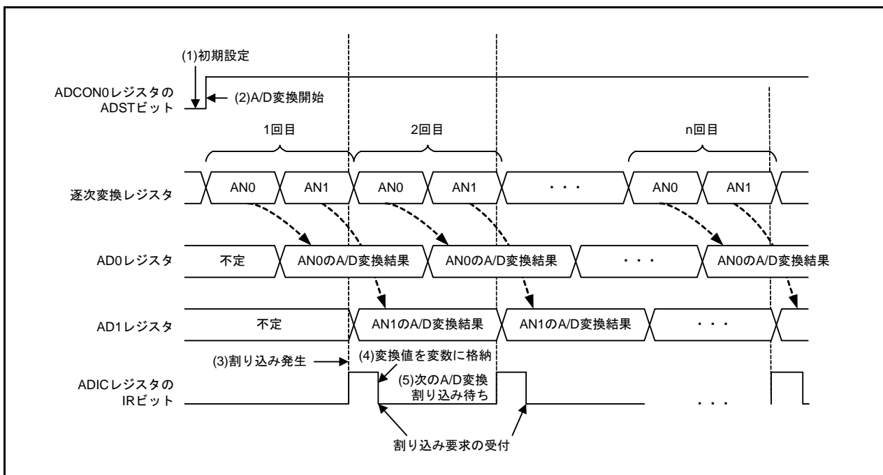
図 4.1 繰り返し掃引モードのタイミング図
