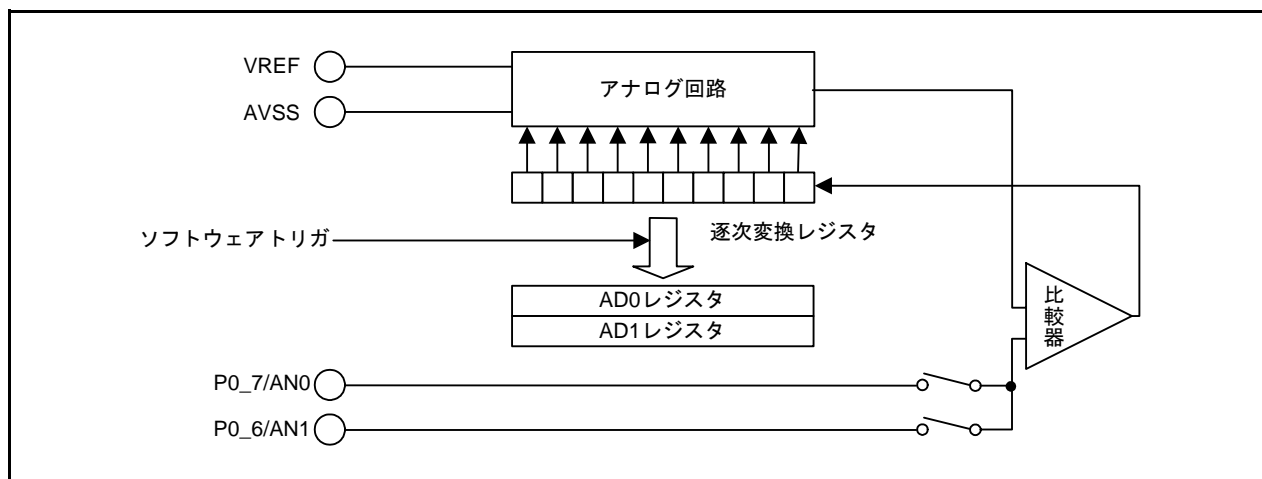
図 1.1 ブロック図
