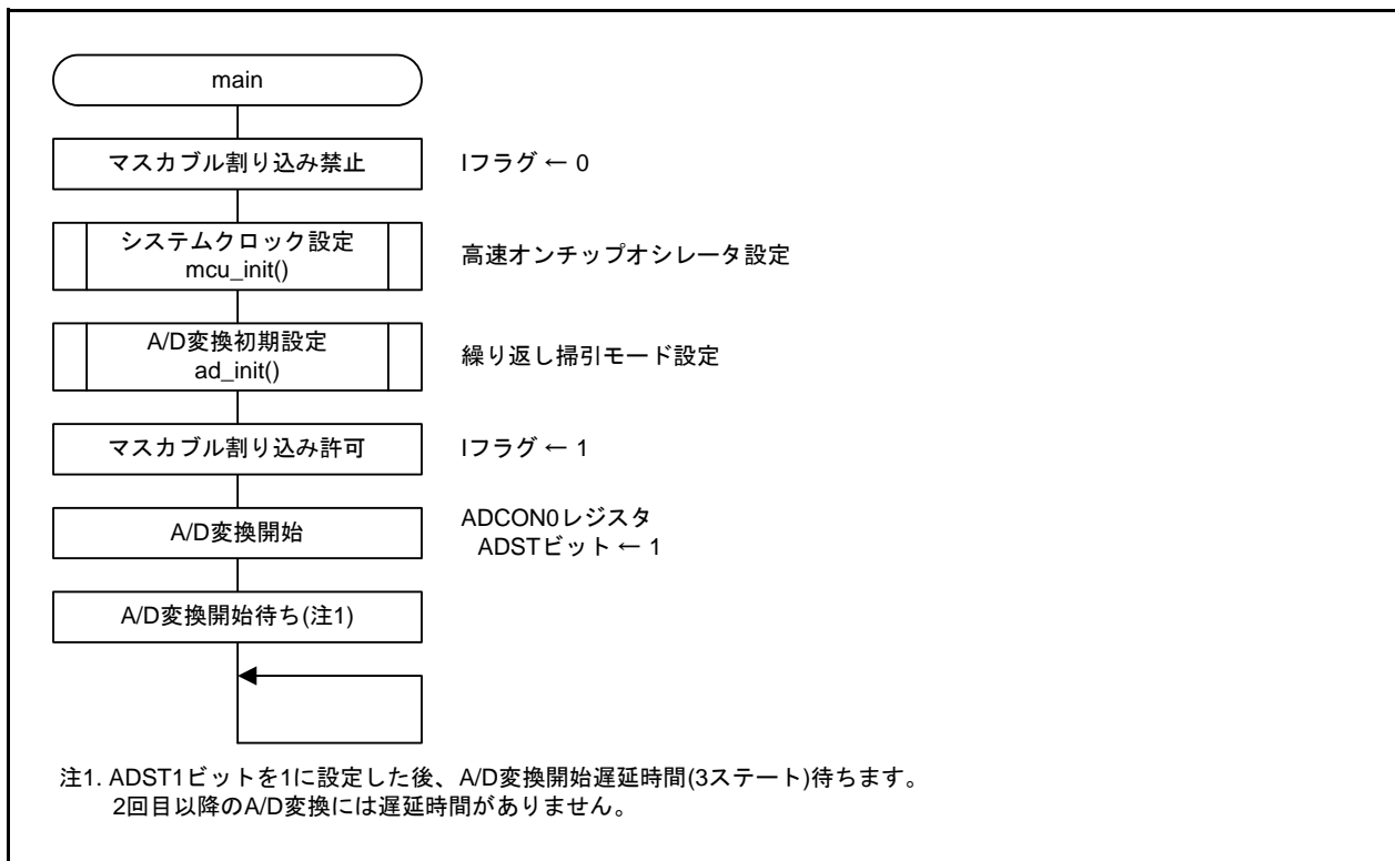
図 4.2 メイン処理
