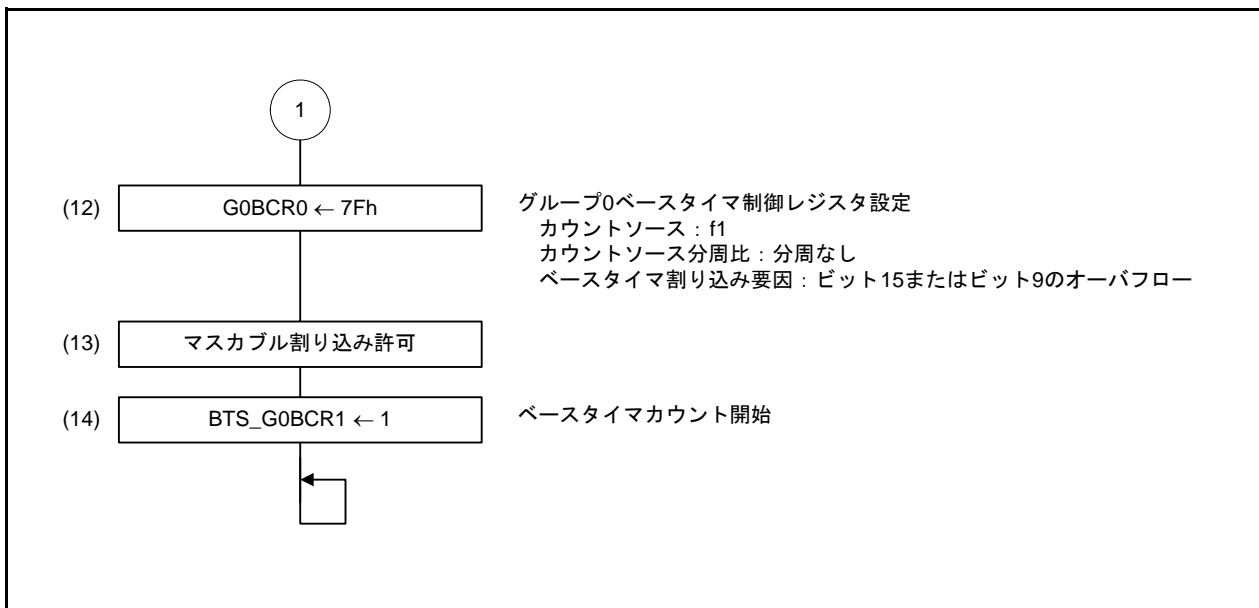
図 3.4 メイン関数のフローチャート (2/2)
