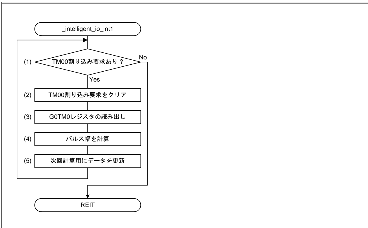
図 3.5 インテリジェント I/O 割り込み 1 のフローチャート
