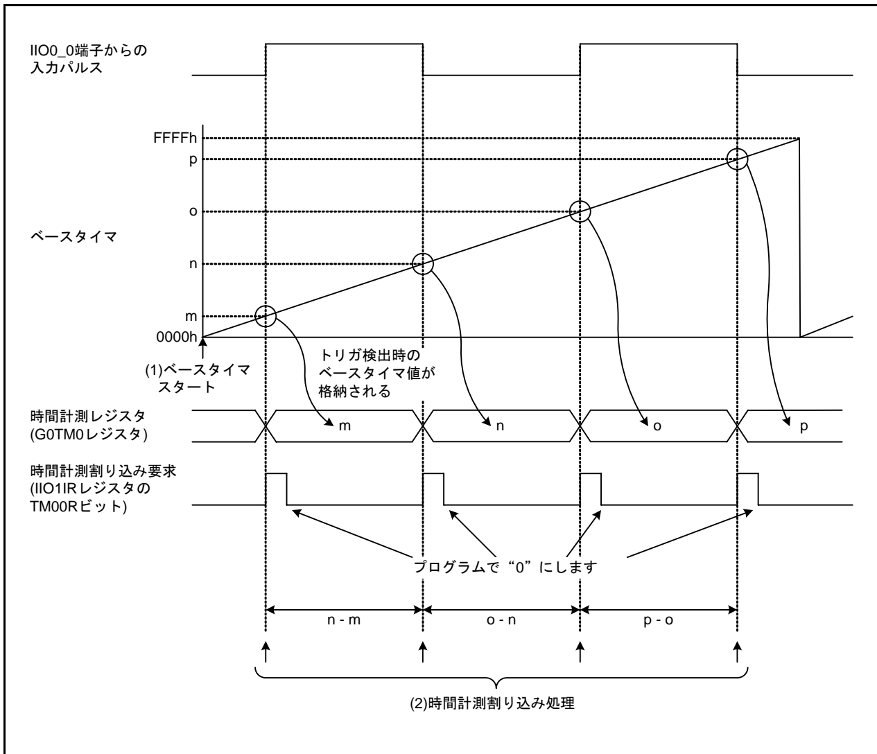
図 3.2 時間計測機能を用いたパルス幅測定の動作例
