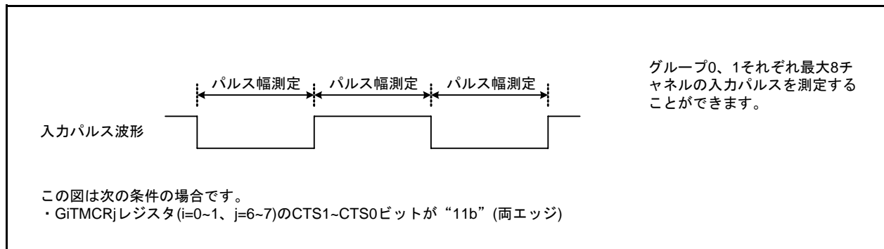
図 3.1 参考入力パルスと計測時間
