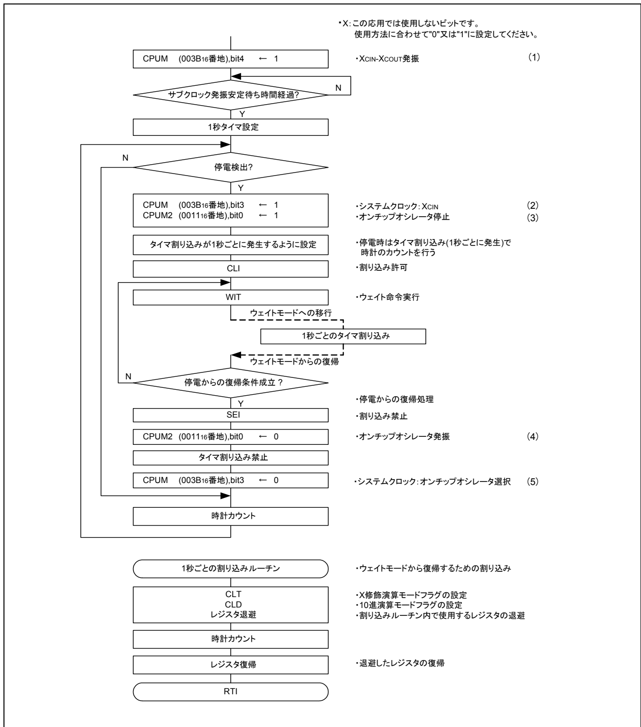
図 3.3 制御手順
