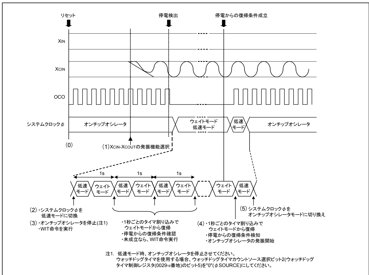
図 3.1 停電時のシステムクロック \phi のモード移行例
