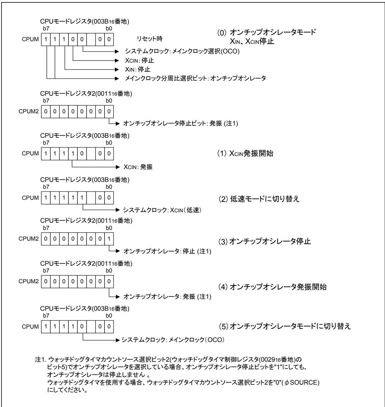
図 3.2 関連レジスタの設定
