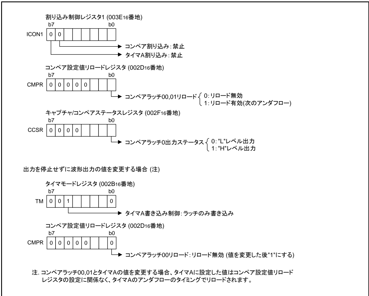
図 3.4 関連レジスタの設定 (2)
