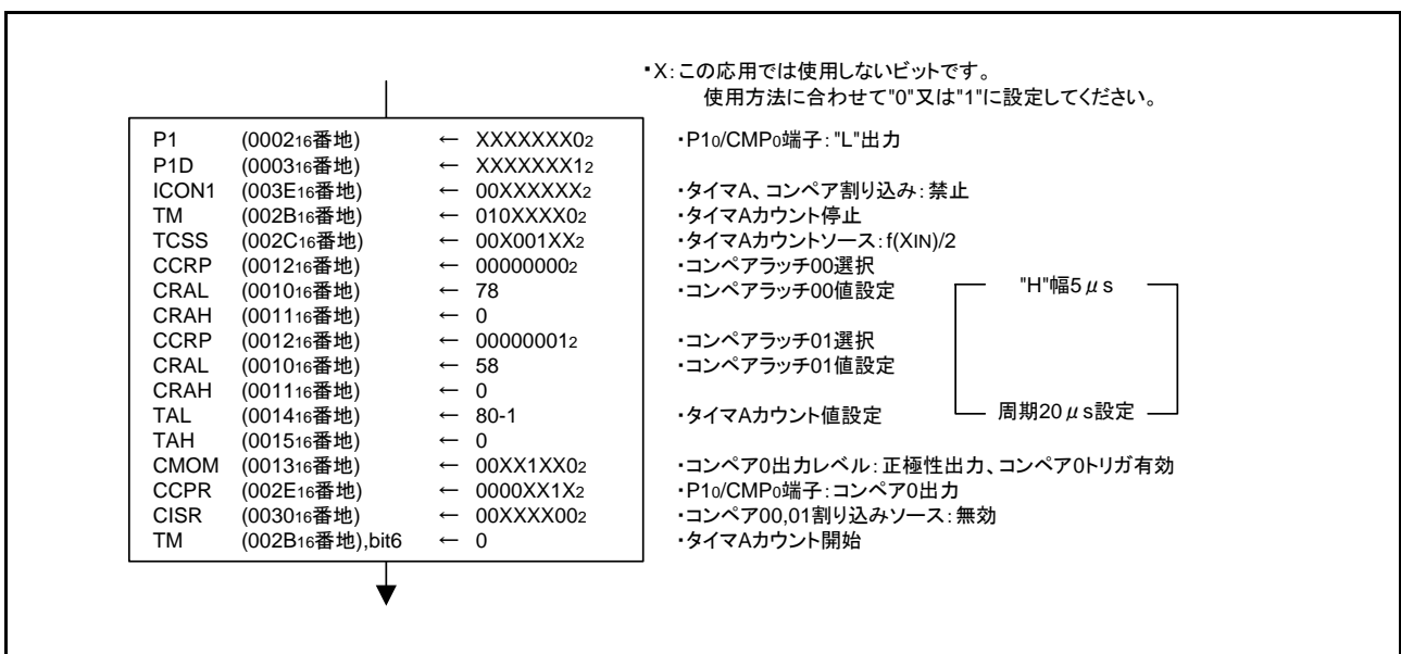
図 3.5 制御手順
