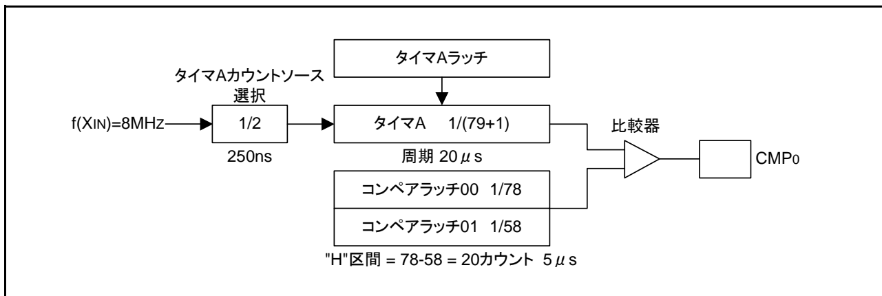
図 3.1 タイマの接続と分周比
