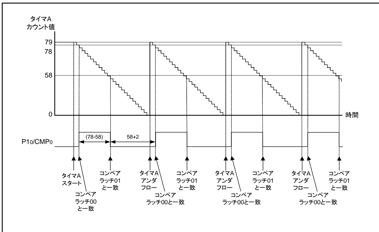
図 3.2 CMP0出力波形
