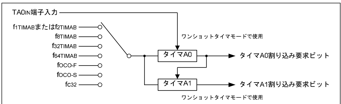
図2. ディレードワンショット出力のタイマ接続図
