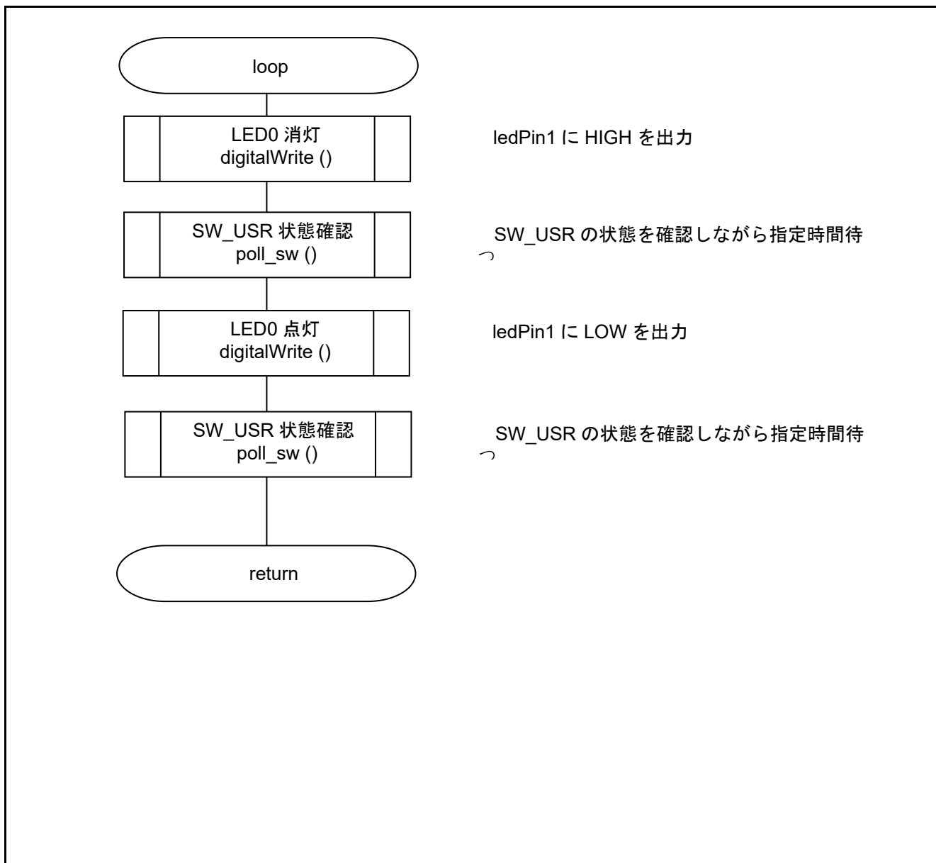
図 5.2 メイン関数
