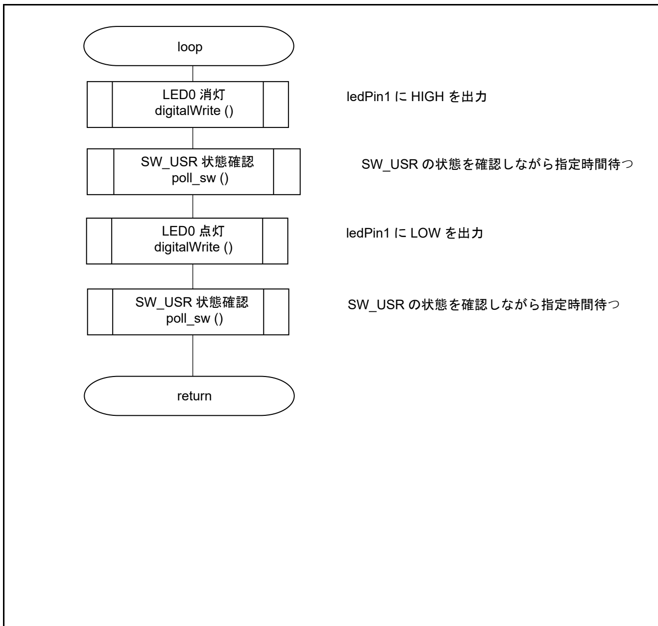
図 5.2 メイン関数
