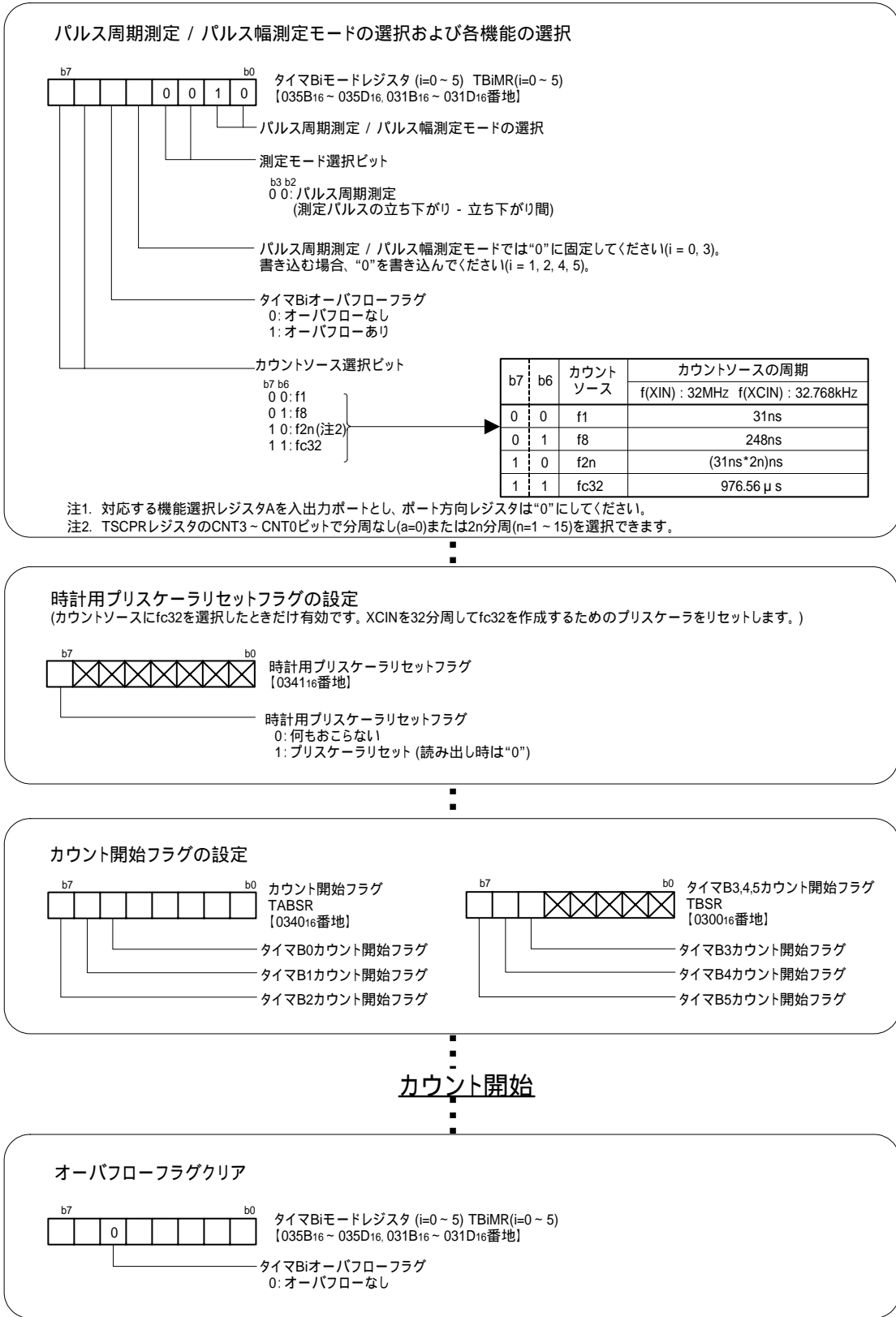
図 2. パルス周期測定モード時のレジスタ設定手順
