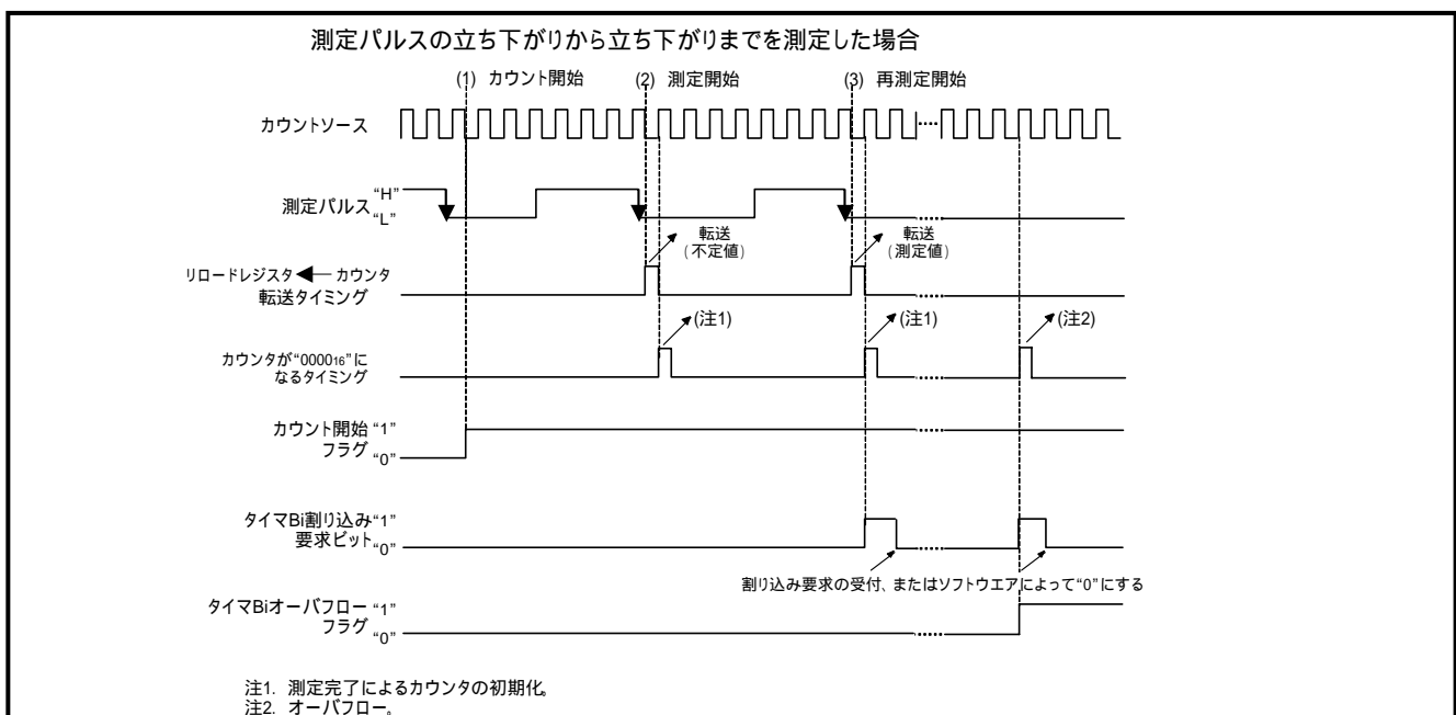
図 1. パルス周期測定モード動作タイミング図
