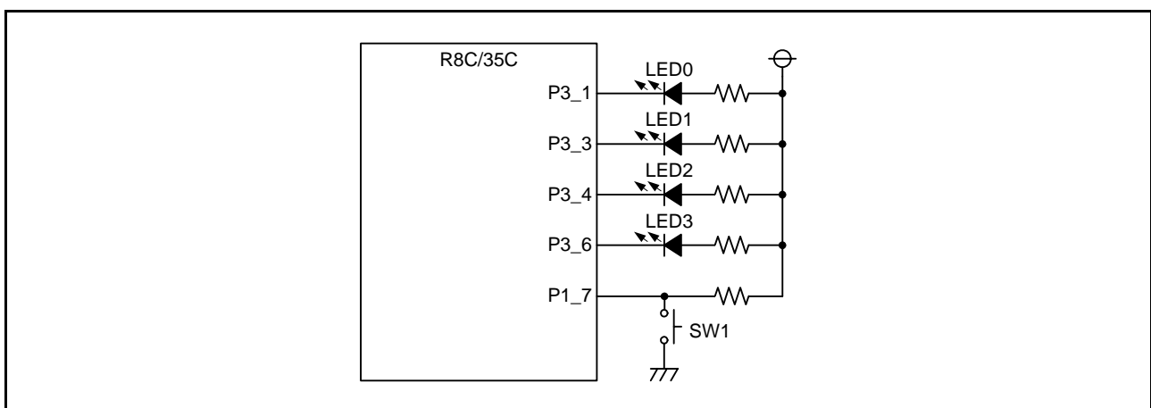
図 3.1 キーおよびLEDの接続例
