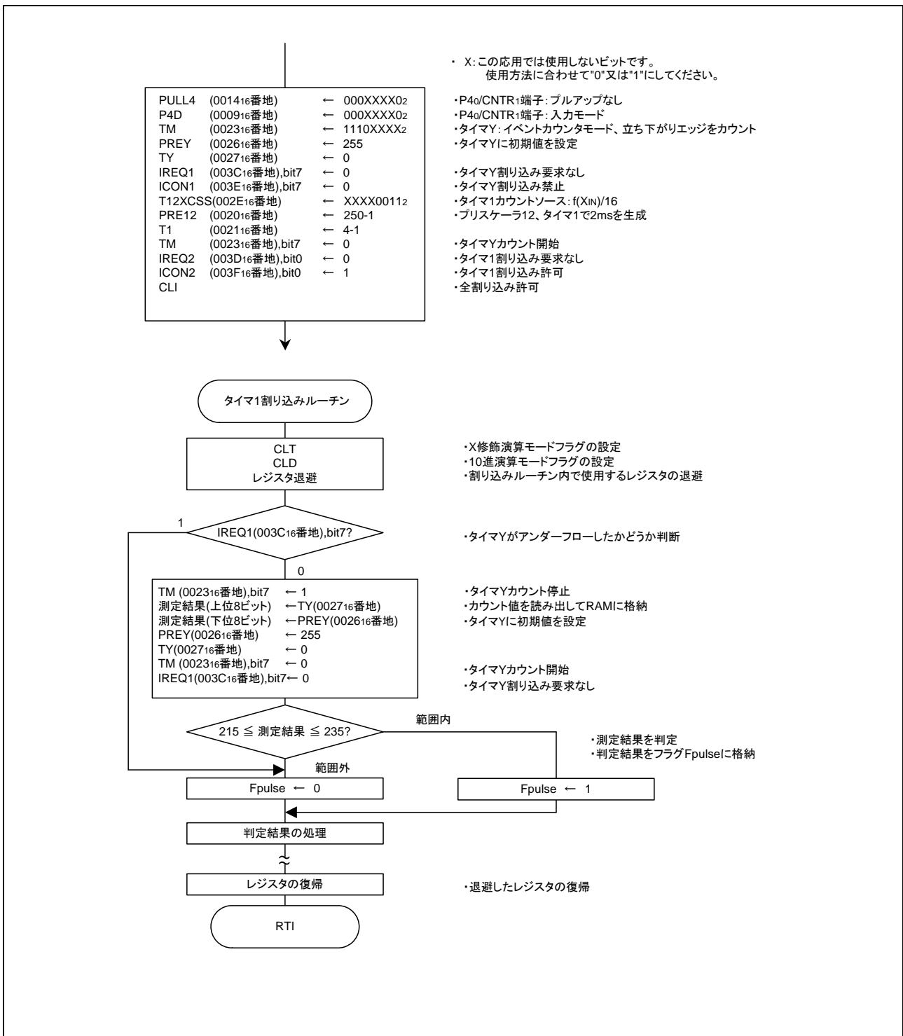
図 3.4 制御手順
