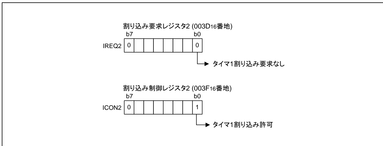
図 3.3 関連レジスタの設定 (2)
