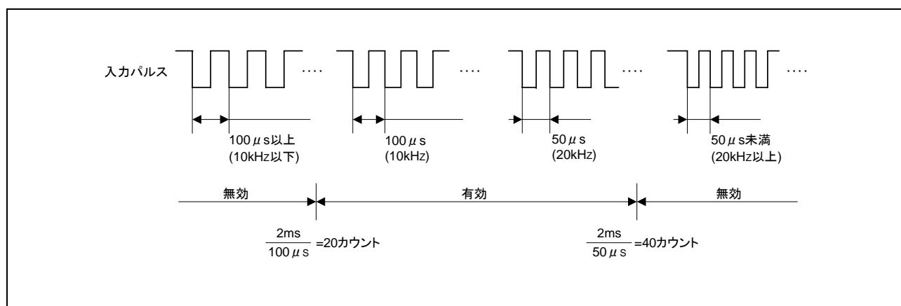
図 3.1 入力パルス有効又は無効の判定方法
