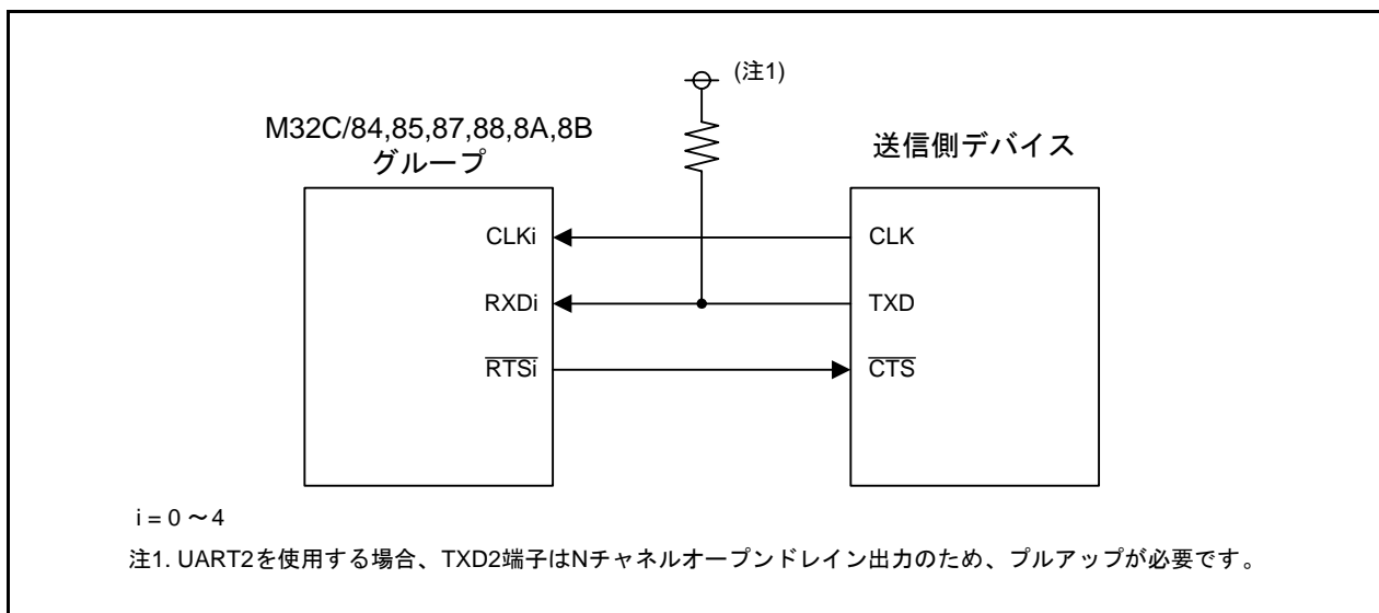
図 1.1 接続例
