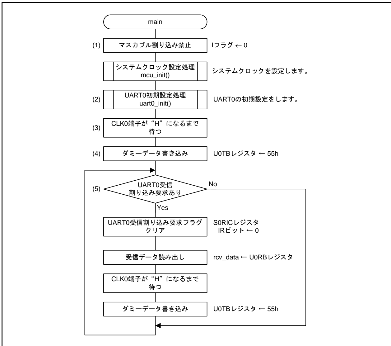
図 5.2 メイン処理
