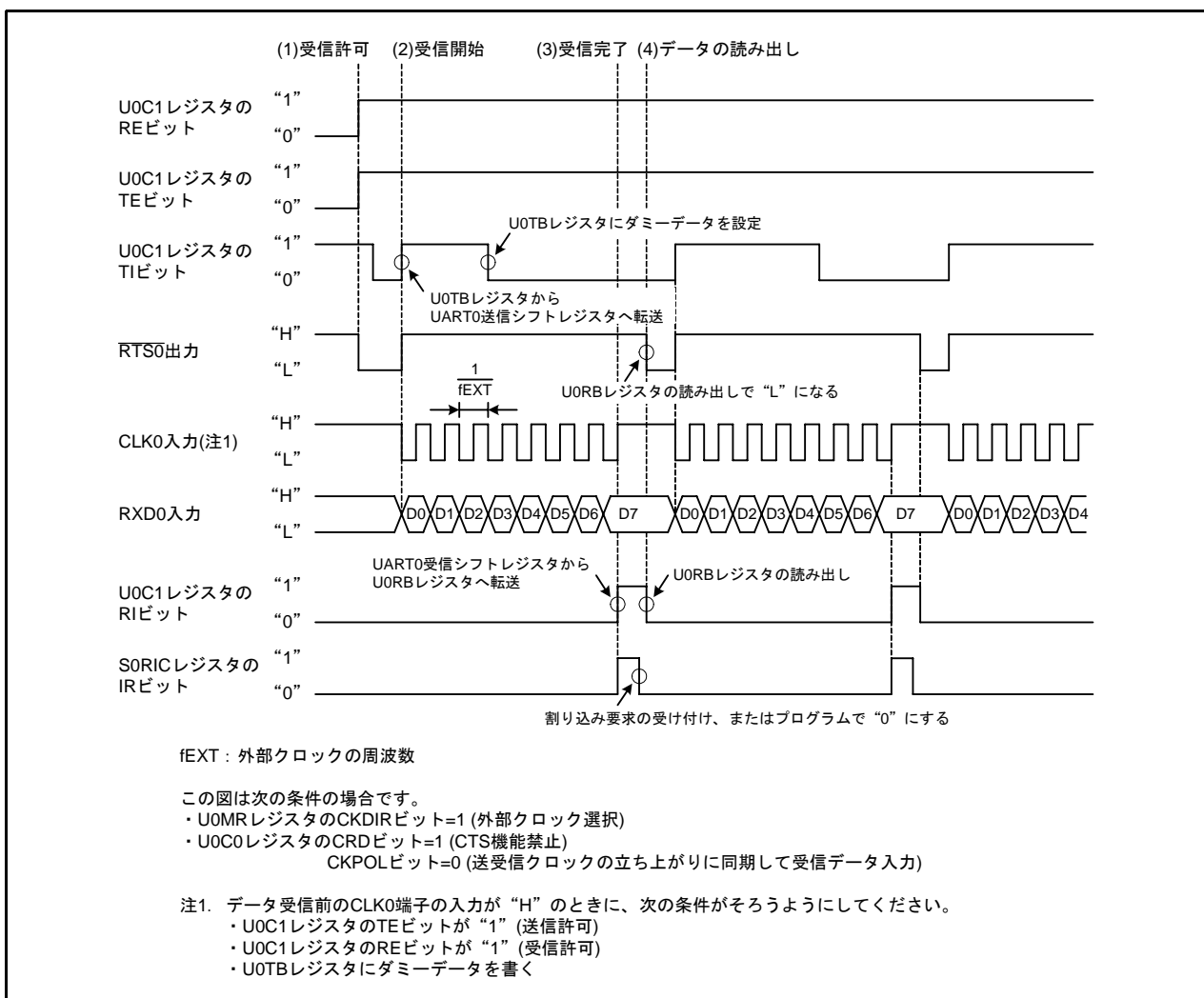
図 5.1 タイミング図
