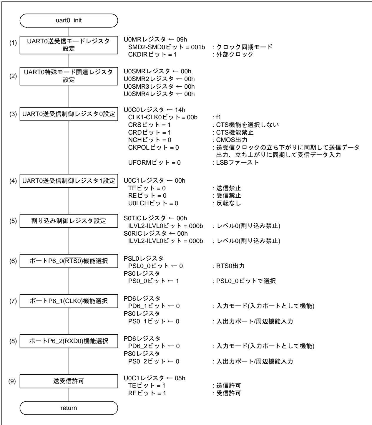
図 5.3 UART0初期設定処理
