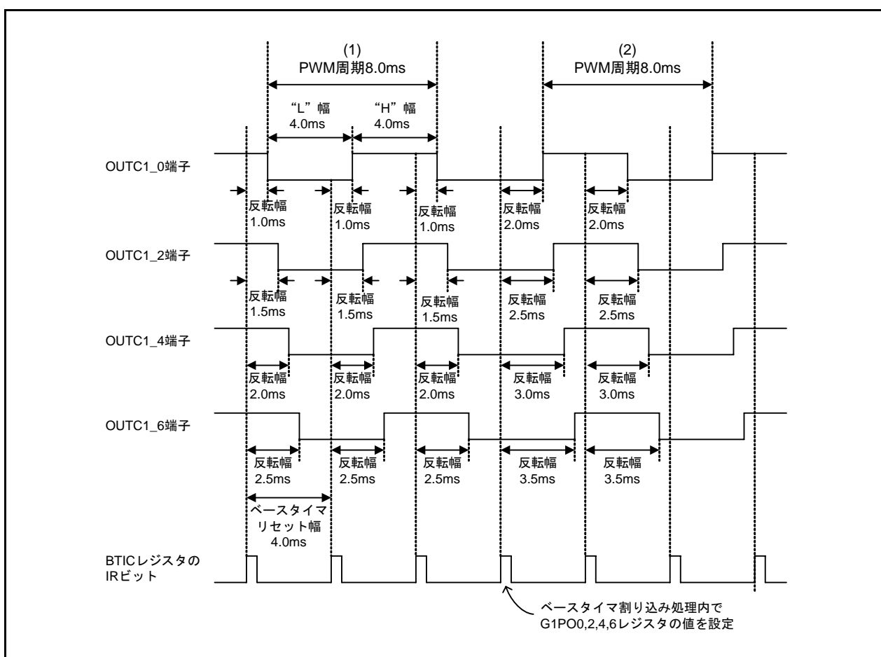
図 2.1 各端子からの出力例
