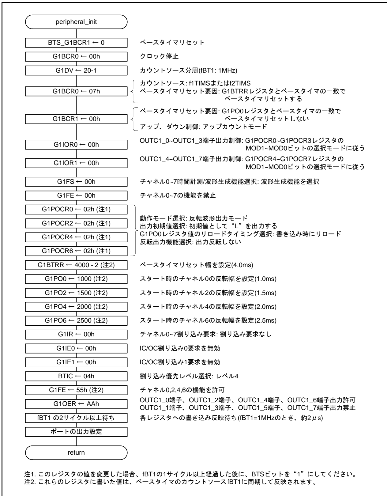
図 2.3 周辺機能初期化関数
