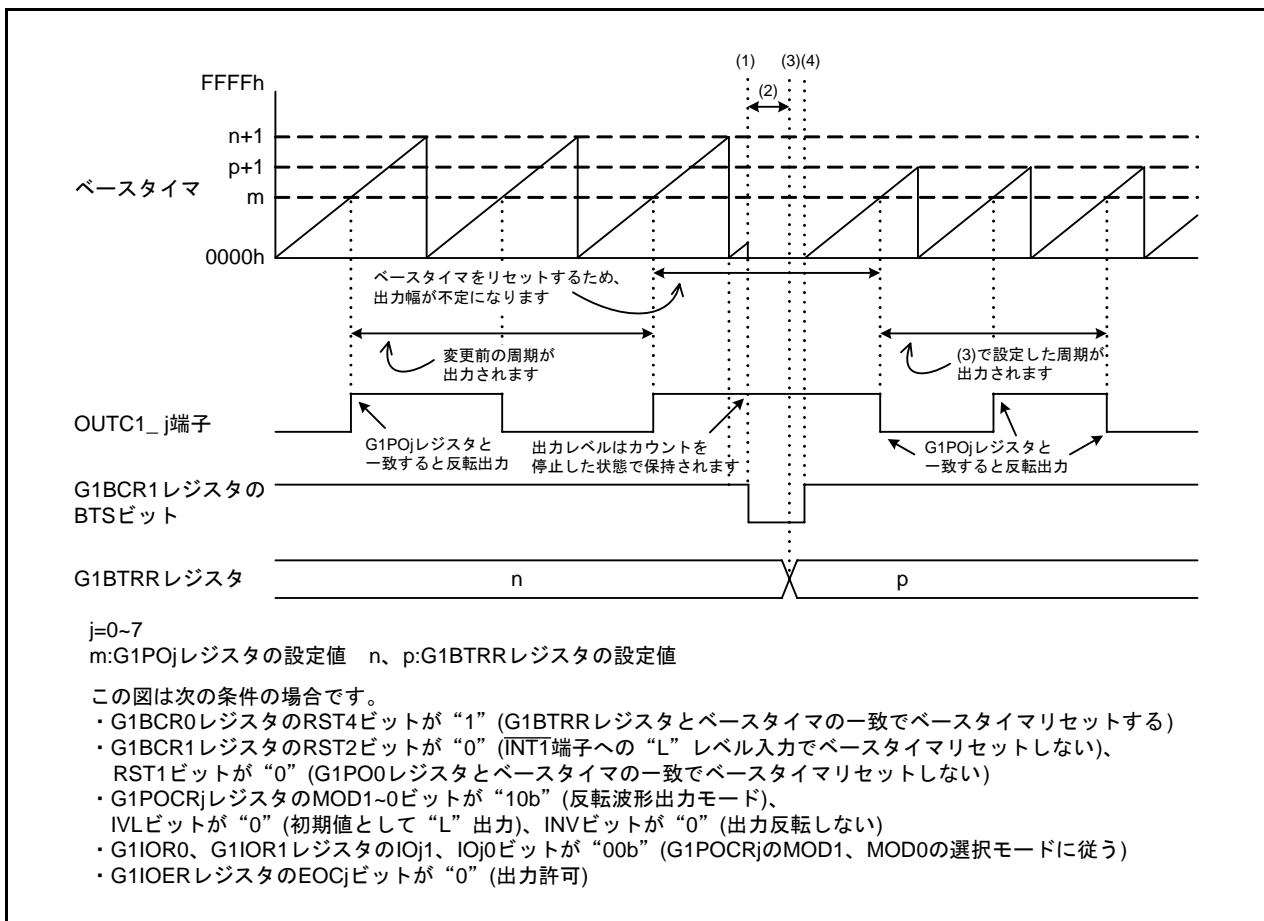
図 3.1 ベースタイマがG1POjレジスタ(j=0~7)と一致する前に周期を変更した場合の出力例
