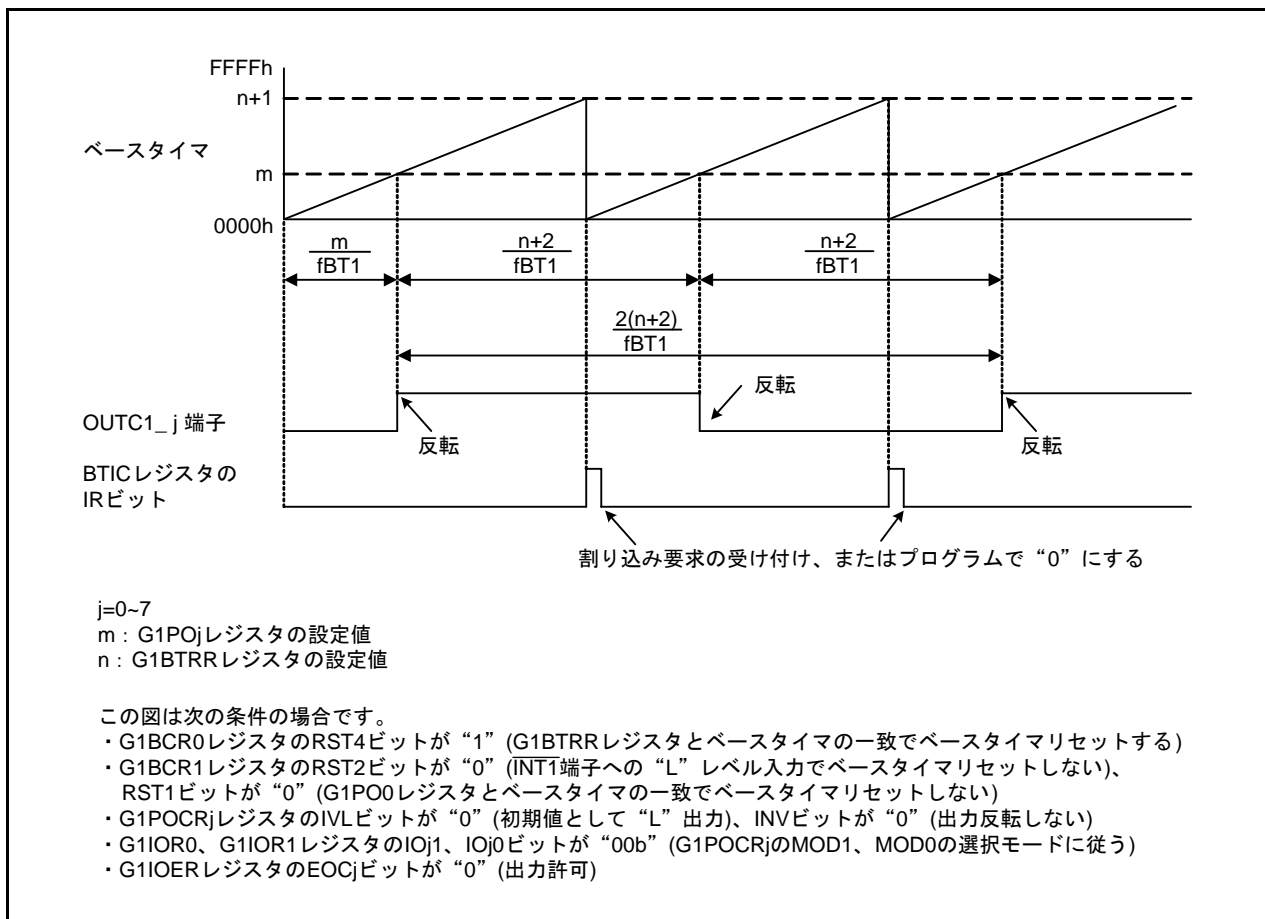
図 1.1 反転波形出力モードの動作例
