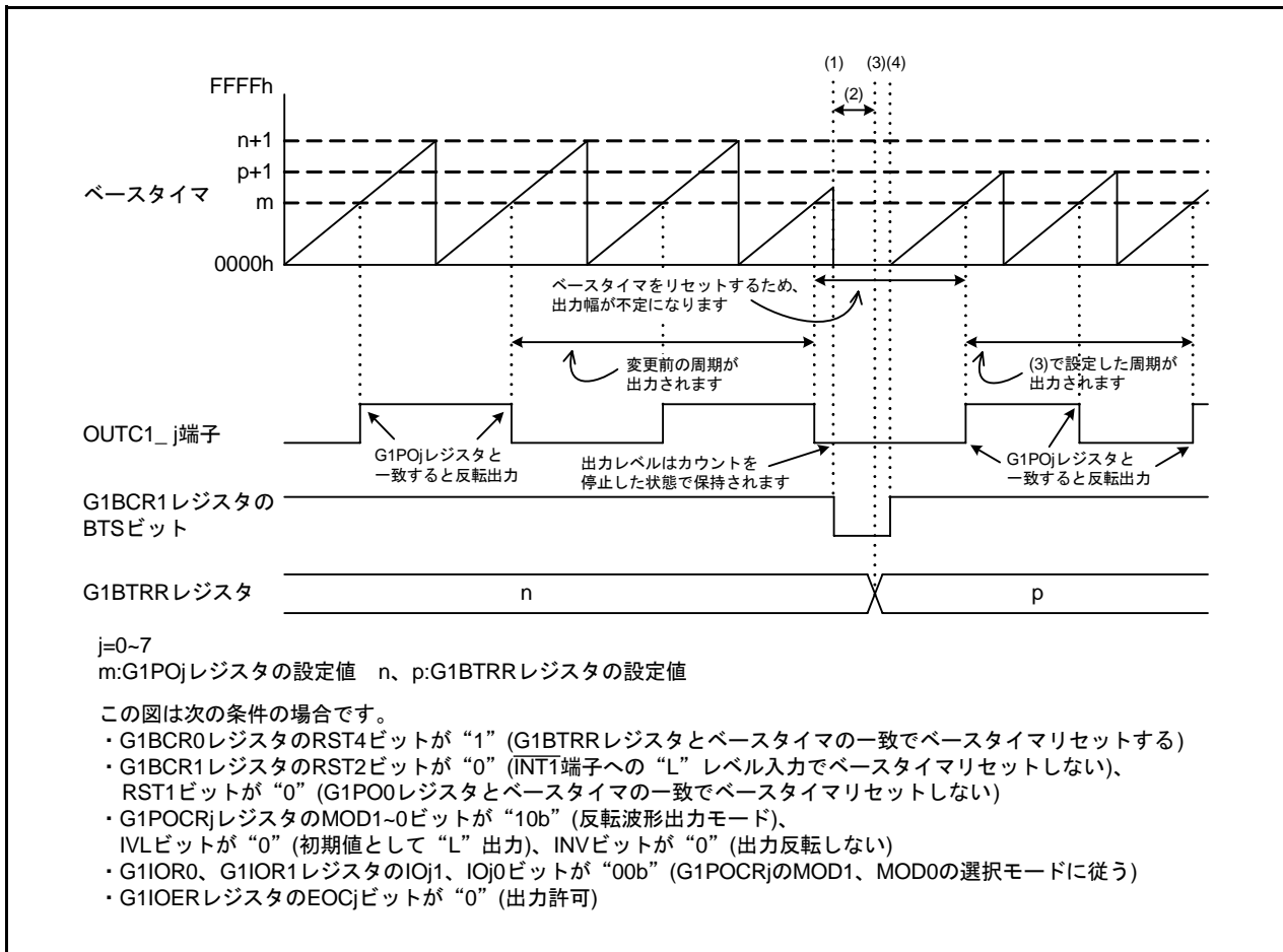
図 3.2 ベースタイマがG1POjレジスタと一致した後に周期を変更した場合の出力例
