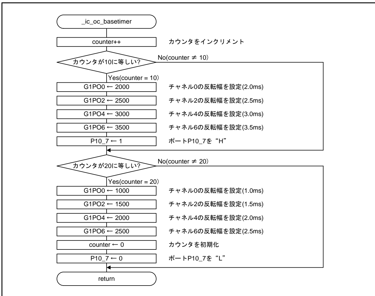
図 2.4 ベースタイマ割り込み処理関数
