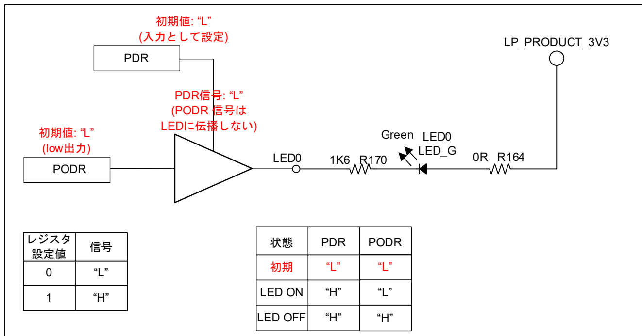
図 1-1 LED ピンの回路図
