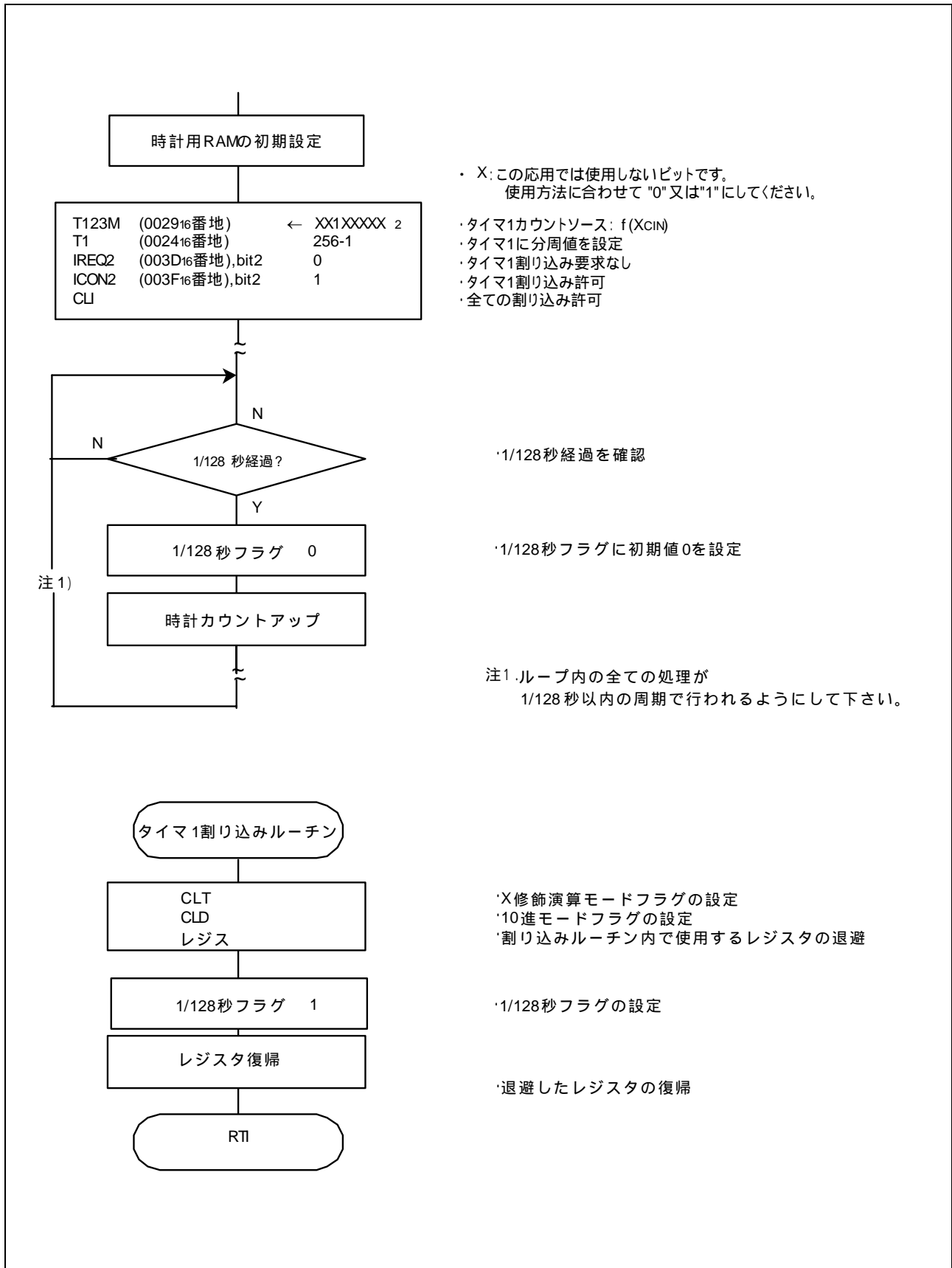
図 3.3 制御手順
