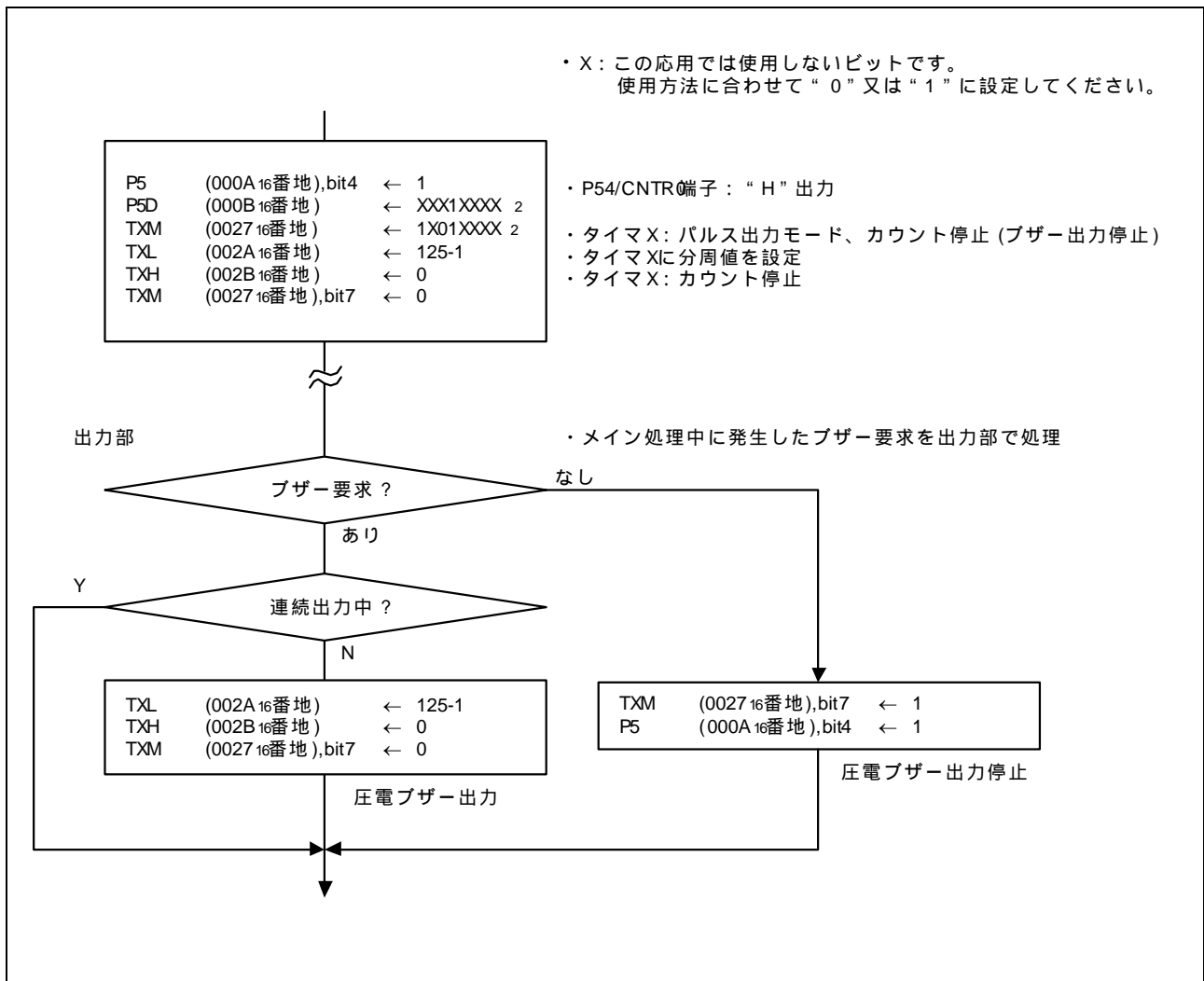
図 3.4 制御手順
