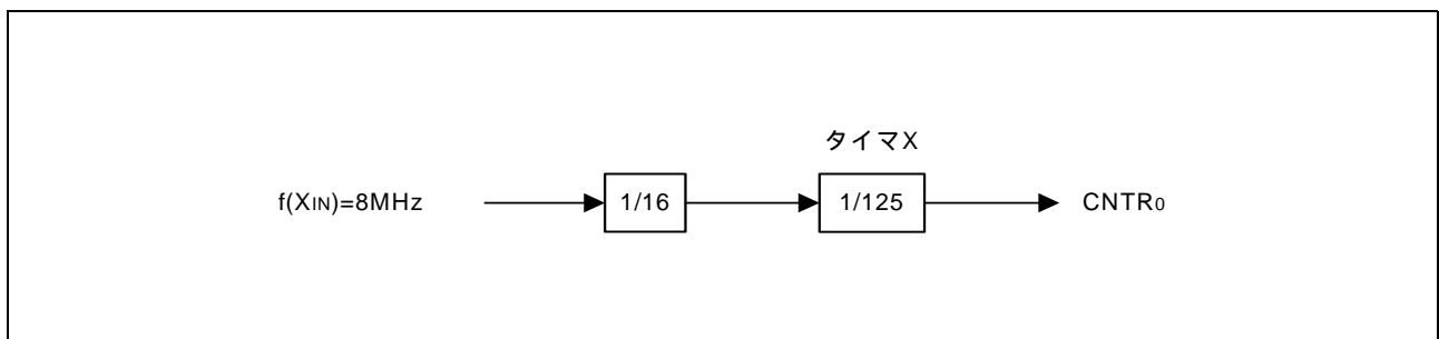
図 3.2 タイマの接続と分周比
