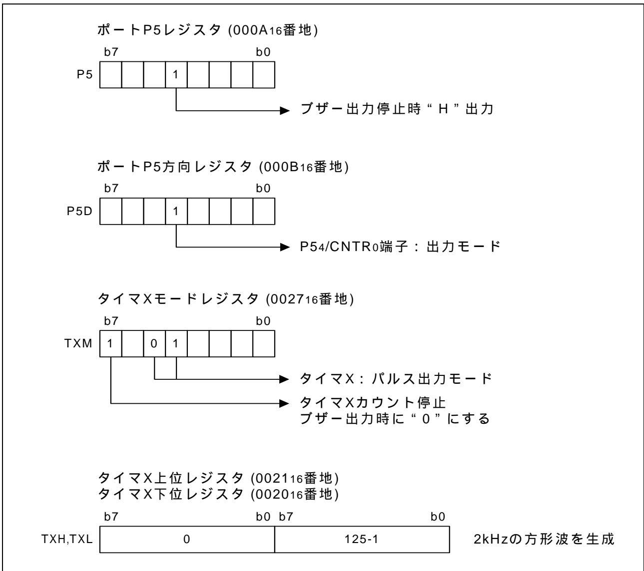
図 3.3 関連レジスタの設定
