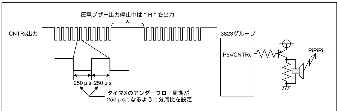
図 3.1 タイマの接続と分周比
