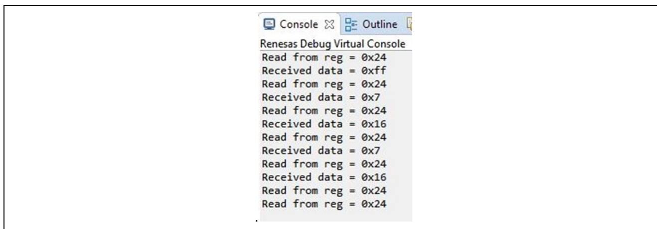
図 2 I 2 C SCI HAL モジュールのアプリケーションプロジェクトのサンプル出力
