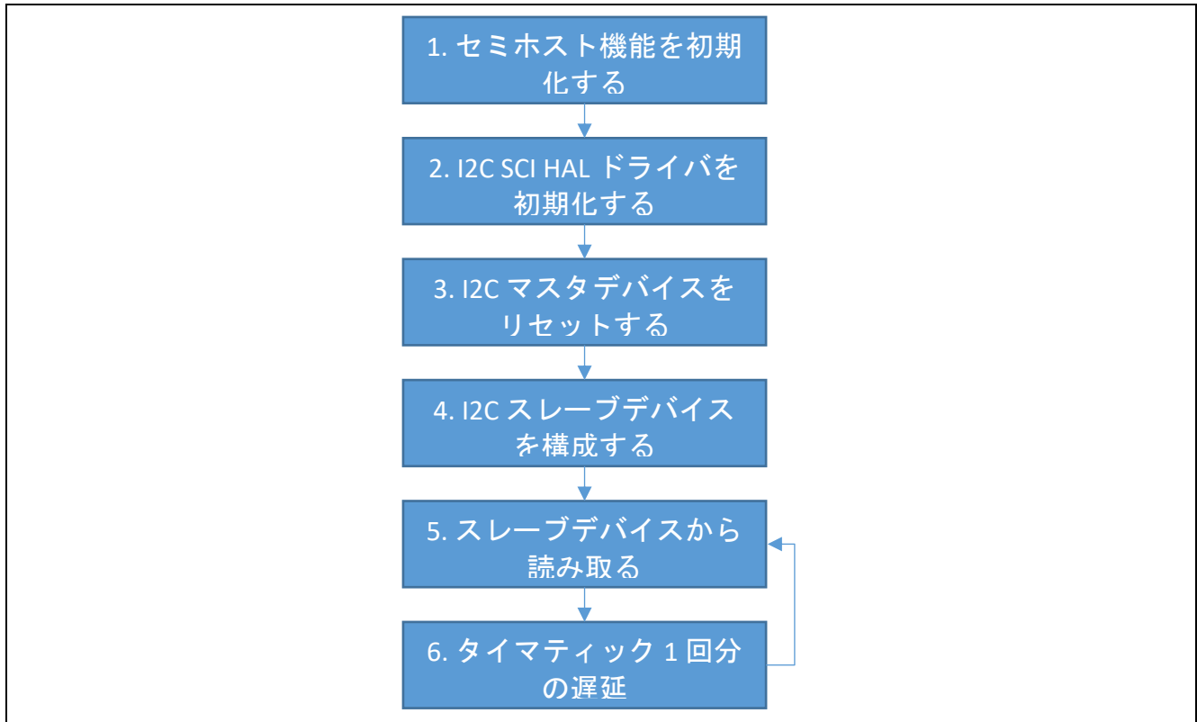
図 1 I 2 C SCI HAL モジュールのアプリケーションプロジェクトのフロー
