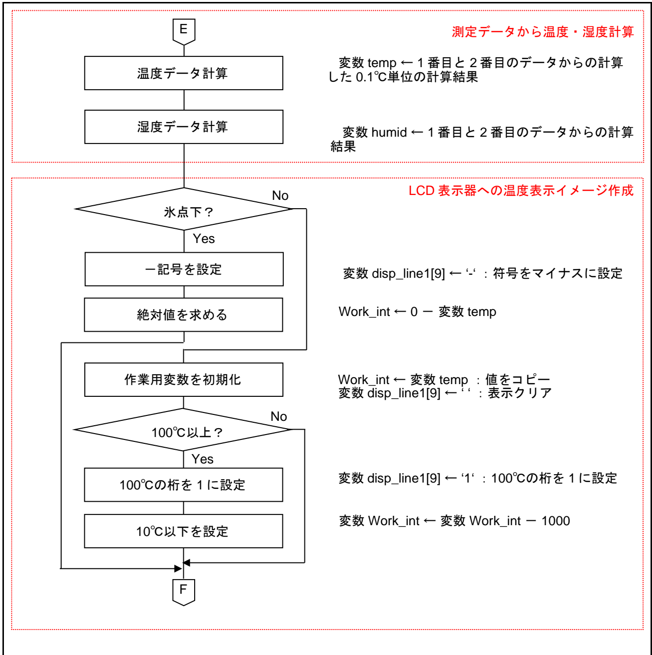
図 5.4 メイン関数 (3/4)
