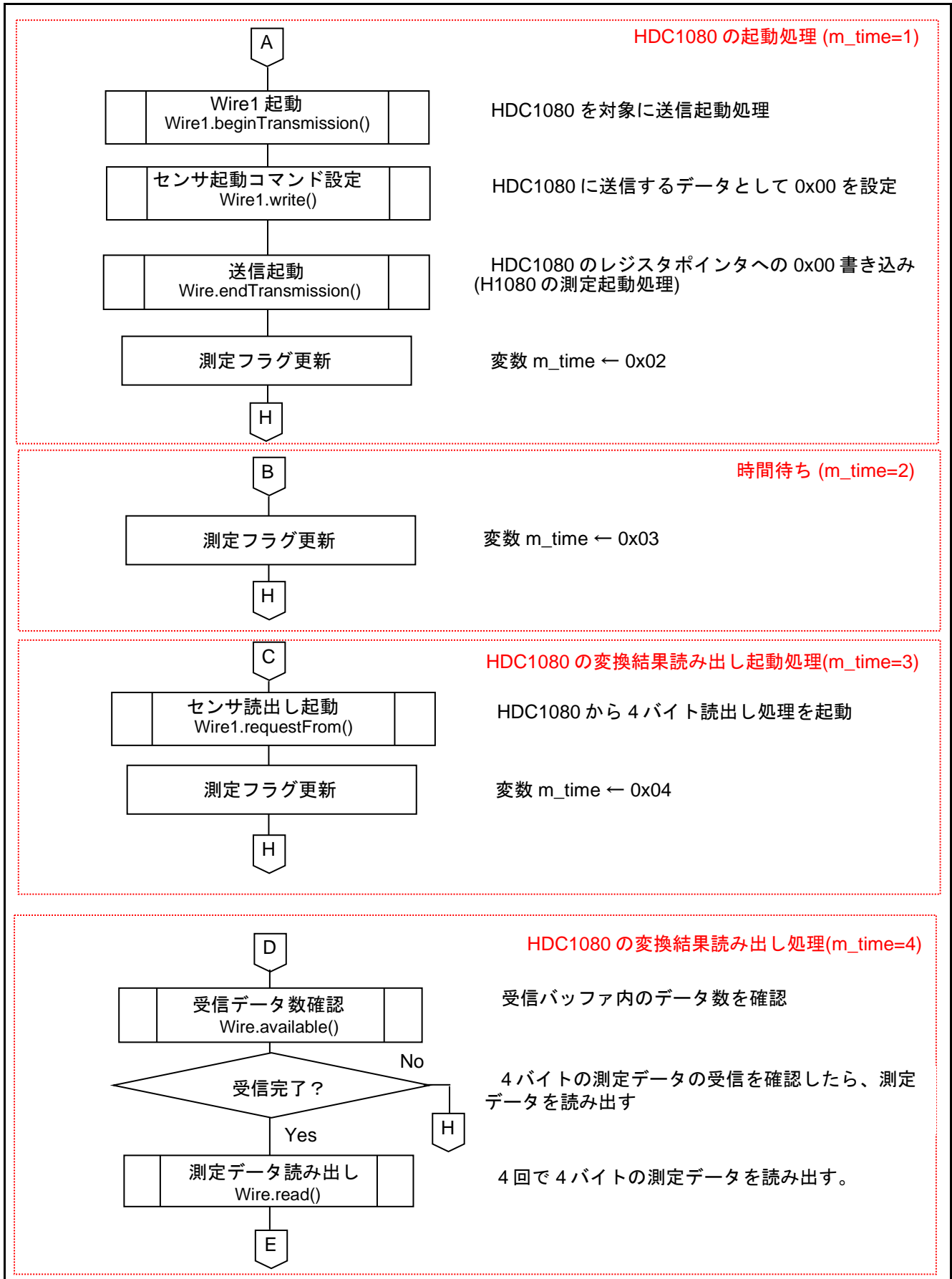
図 5.3 メイン関数 (2/4)
