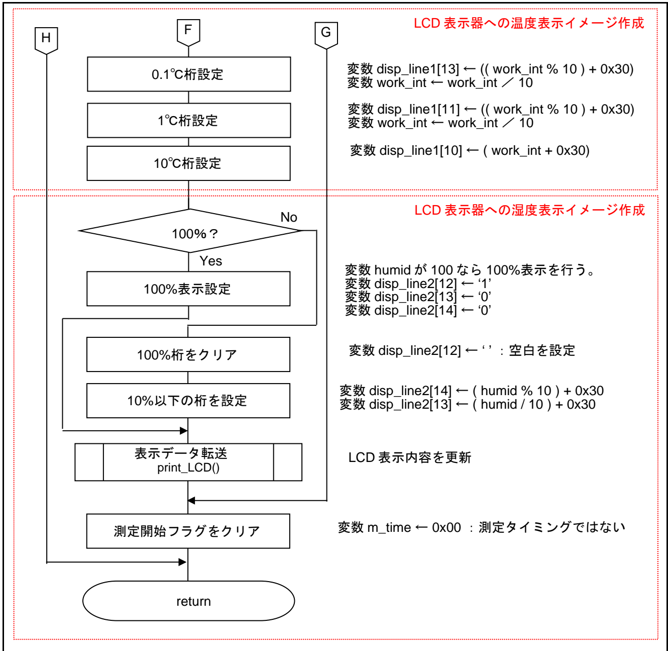
図 5.5 メイン関数 (4/4)
