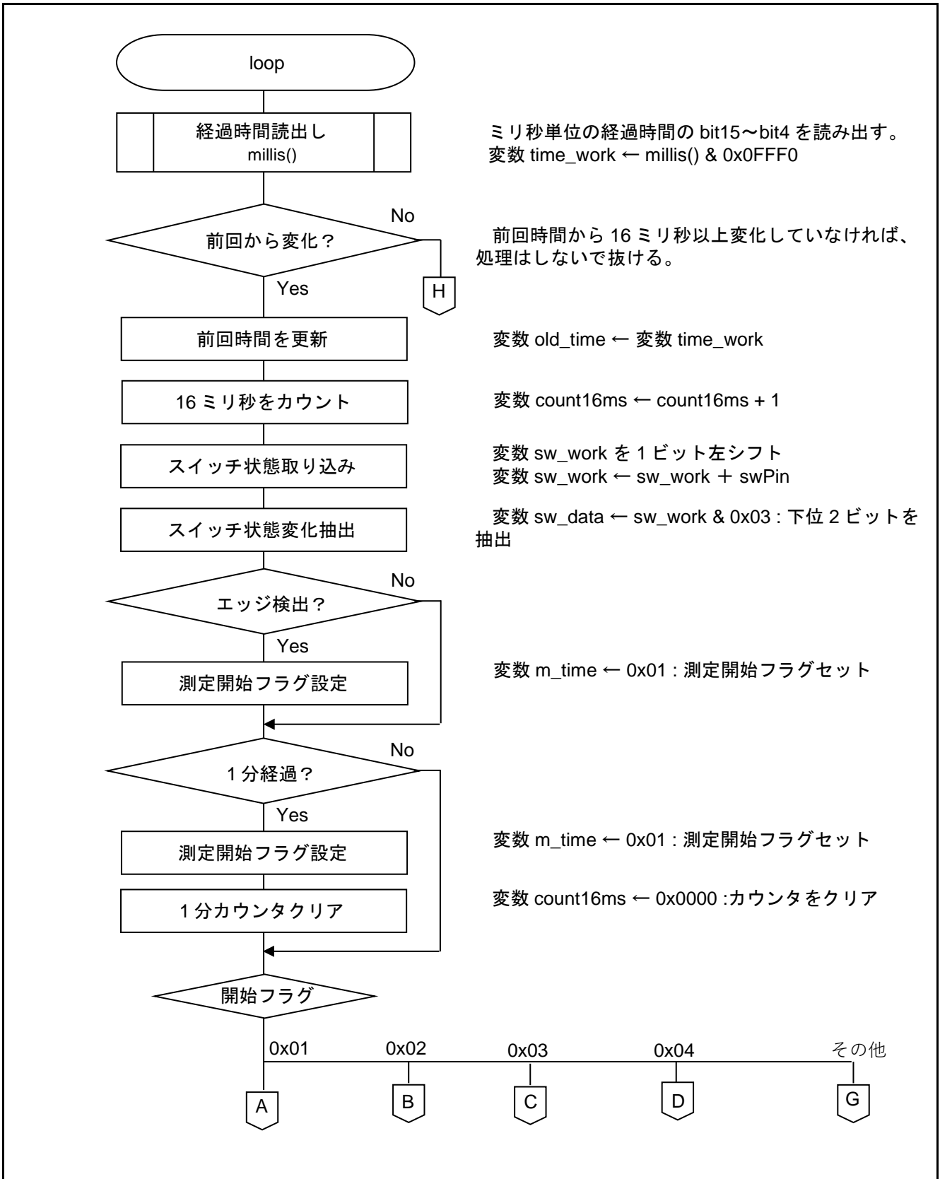
図 5.2 メイン関数 (1/4)
