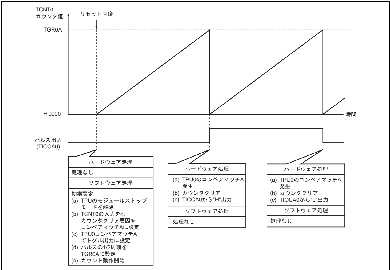
図3 パルス出力動作原理
