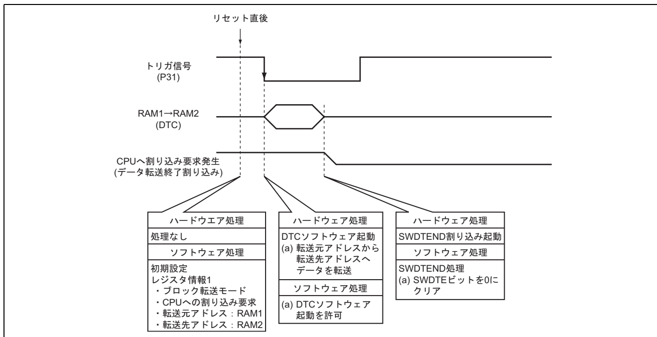
図3 ソフトウェア起動によるデータ転送動作原理
