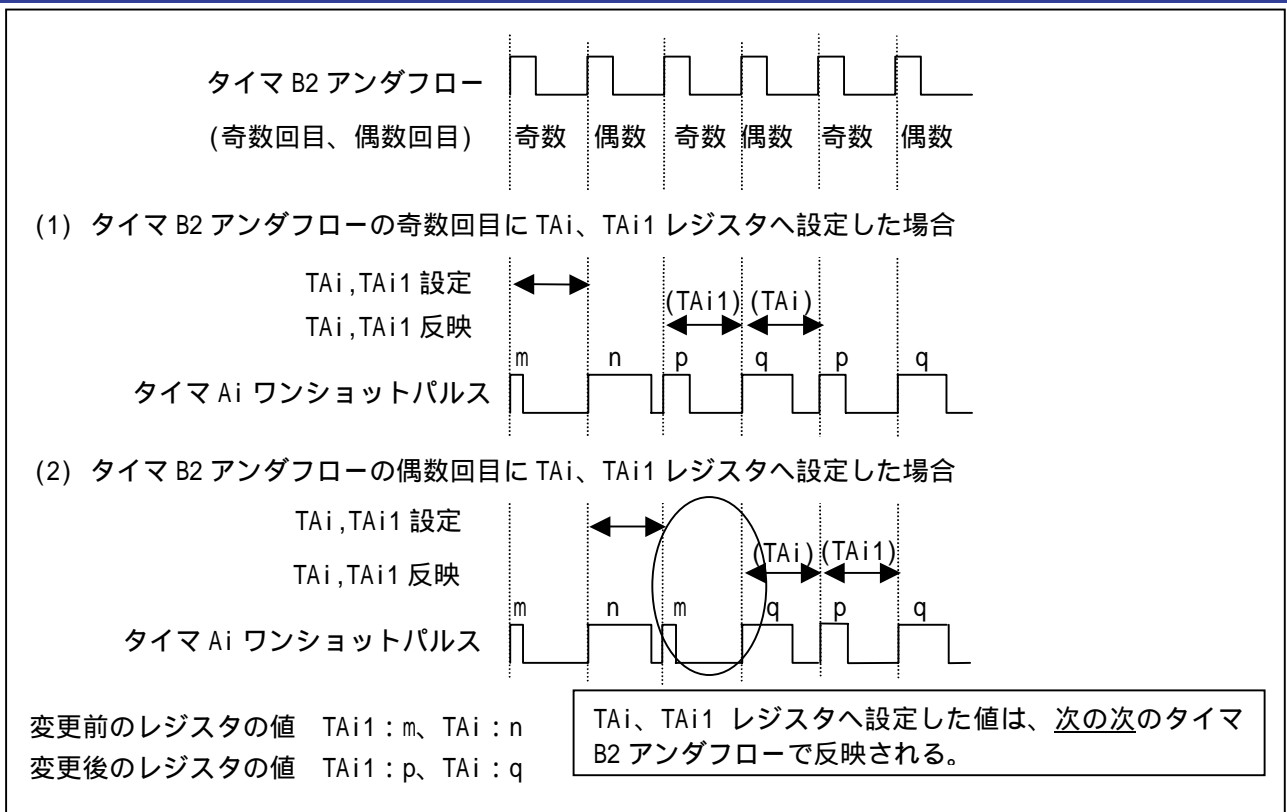
図 1. M16C/62 グループの三相モード 1
