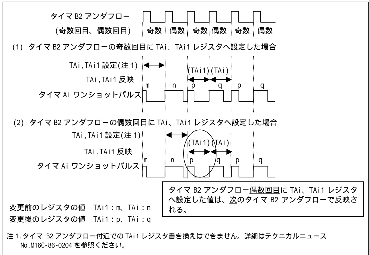
図 2. M16C/62P、M16C/80、M32C/83 グループの三相モード 1
