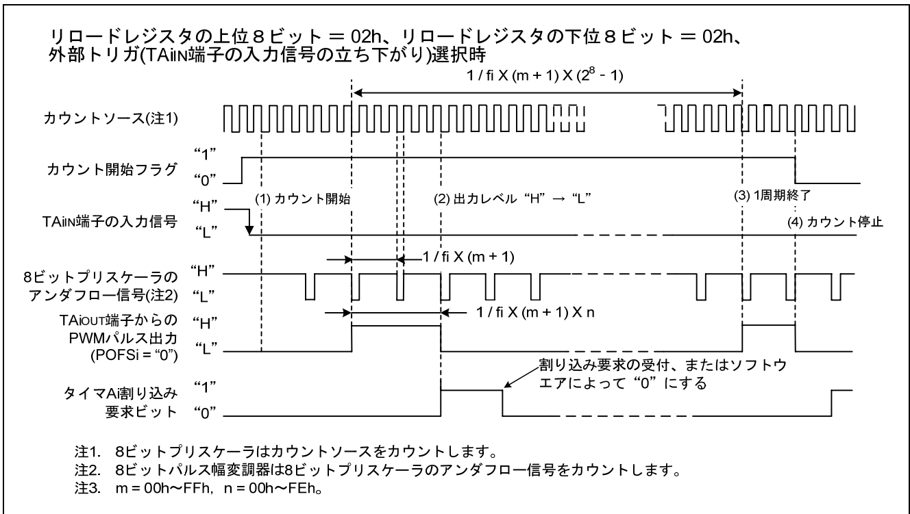
図1 パルス幅変調モード動作、8ビット PWM モード選択時のタイミング
