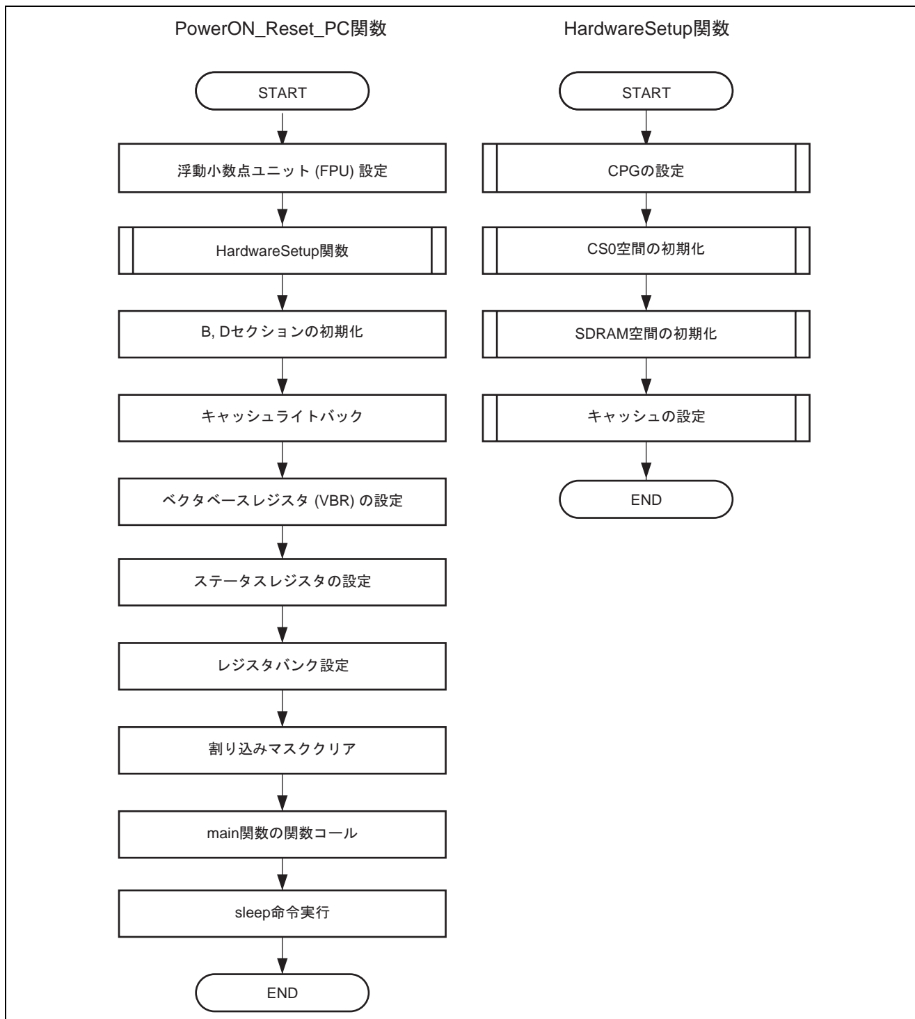
図 1 PowerON_Reset_PC 関数と HardwareSetup 関数の処理フロー
