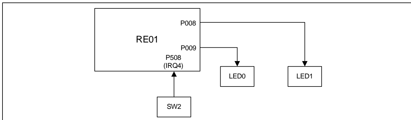
図 3.1 システム構成図
