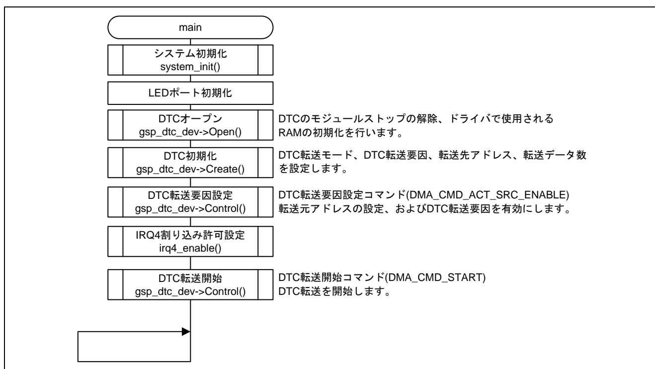
図 3-2 メイン処理
