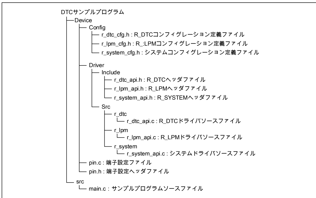
図 1-1 フォルダ構成
