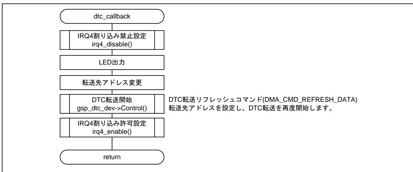
図 3-6 DTC 転送完了コールバック
