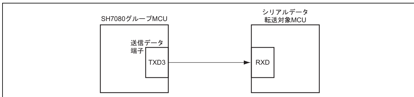
図 1 FIFO 付き調歩同期式シリアルデータ送信動作概要
