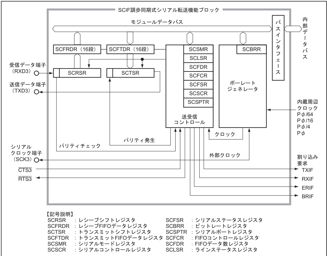
図 2 シリアルコミュニケーションインタフェース (SCIF) のブロック図
